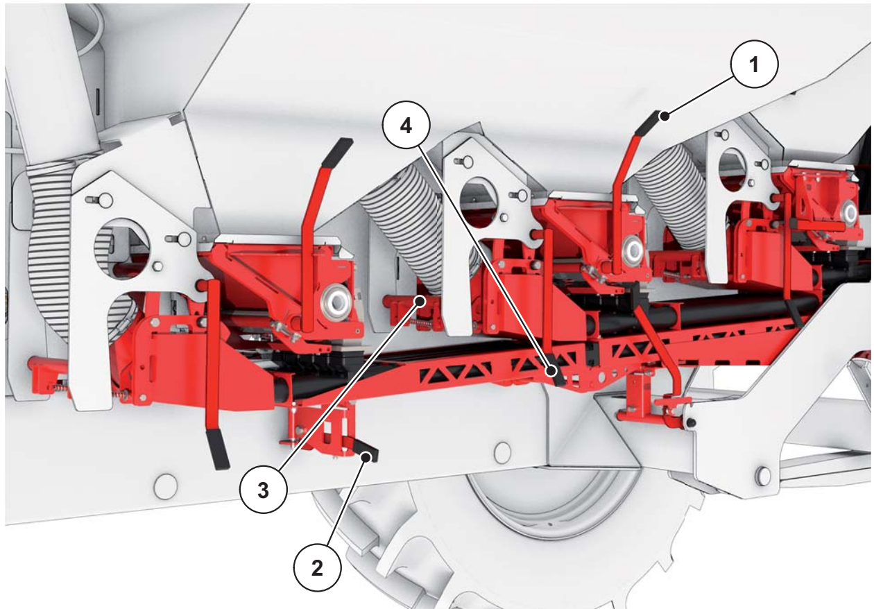
Bild 7.9: Luftführung zusammenbauen
