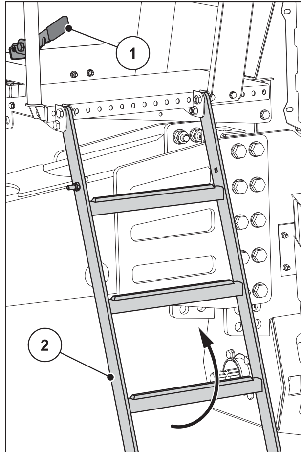
Bild 6.14: Aufstieg einklappen
