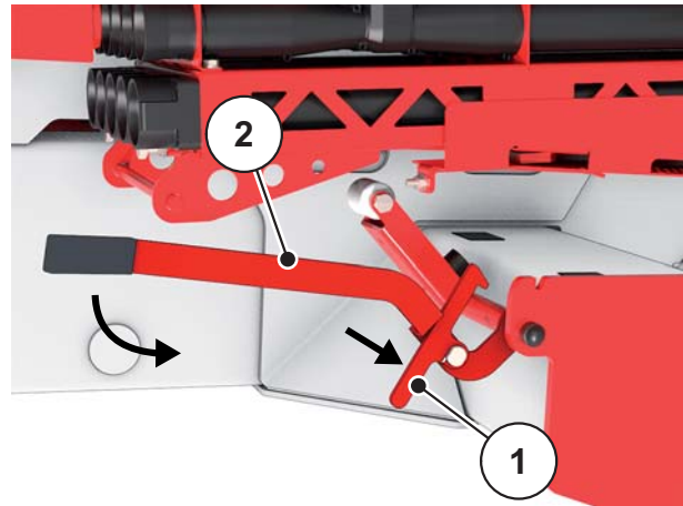
Bild 8.7: Hintere Luftführung entriegeln
