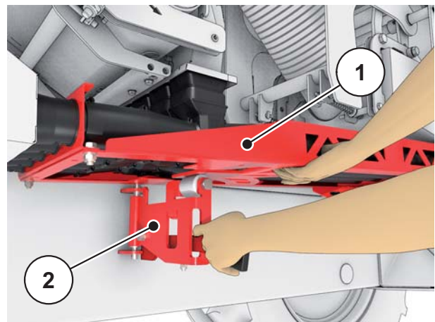
Bild 7.3: Hebel der Luftführungs-Ablage entriegeln
