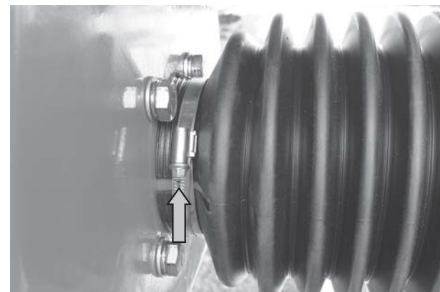
Bild 6.5: Gelenkwellenschutz sichern
