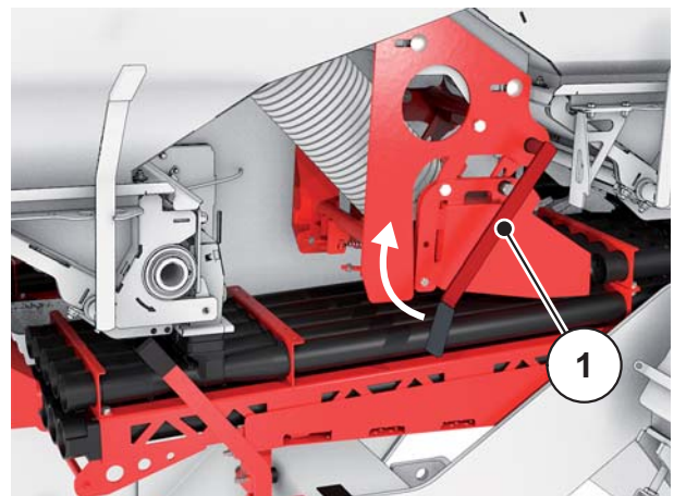
Bild 8.6: Hintere Druckkammer lösen
