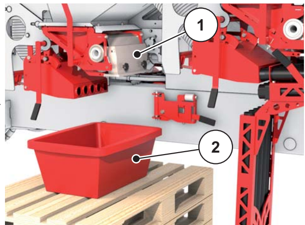
Bild 7.6: Düngemittelauffangbehälter unter der Dosiereinrichtung
