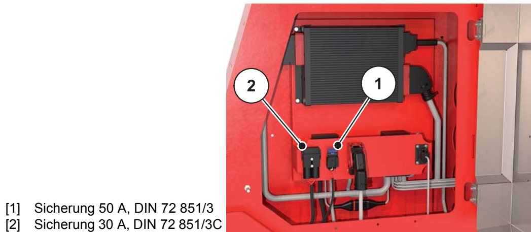
Bild 10.28: Sicherungen am RAUCH-ISOBUS-Kabel
