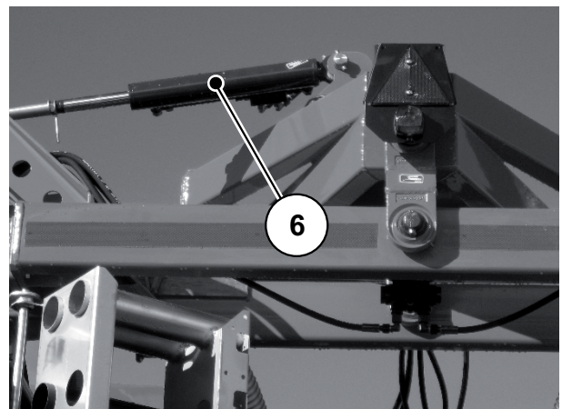
Bild 10.20: Hydrozylinder Hangneigung
