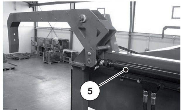
Bild 10.19: Hydrozylinder Transportverriegelung
