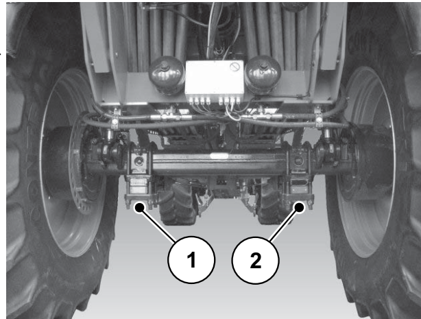
Bild 10.26: Ansetzpunkte Wagenheber
