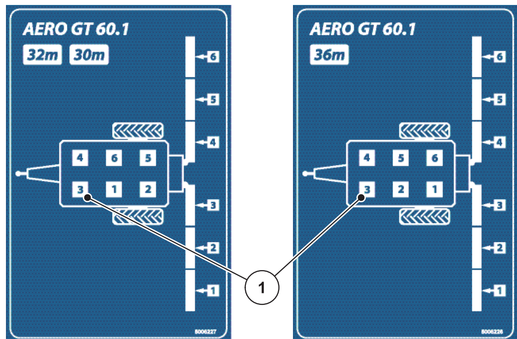
Bild 7.1: Darstellung der Teilbreiten am Ausleger-Mineraldüngerstreuer
