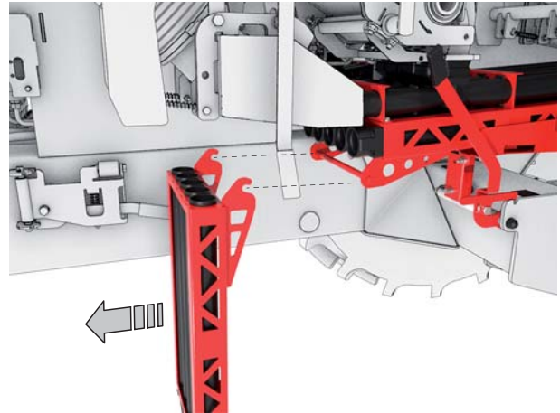
Bild 8.4: Luftführung aushängen.
