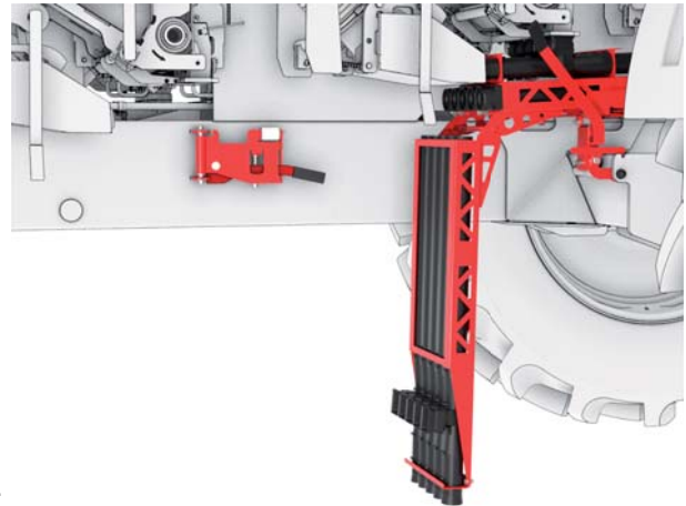
Bild 7.5: Luftführung ablassen
