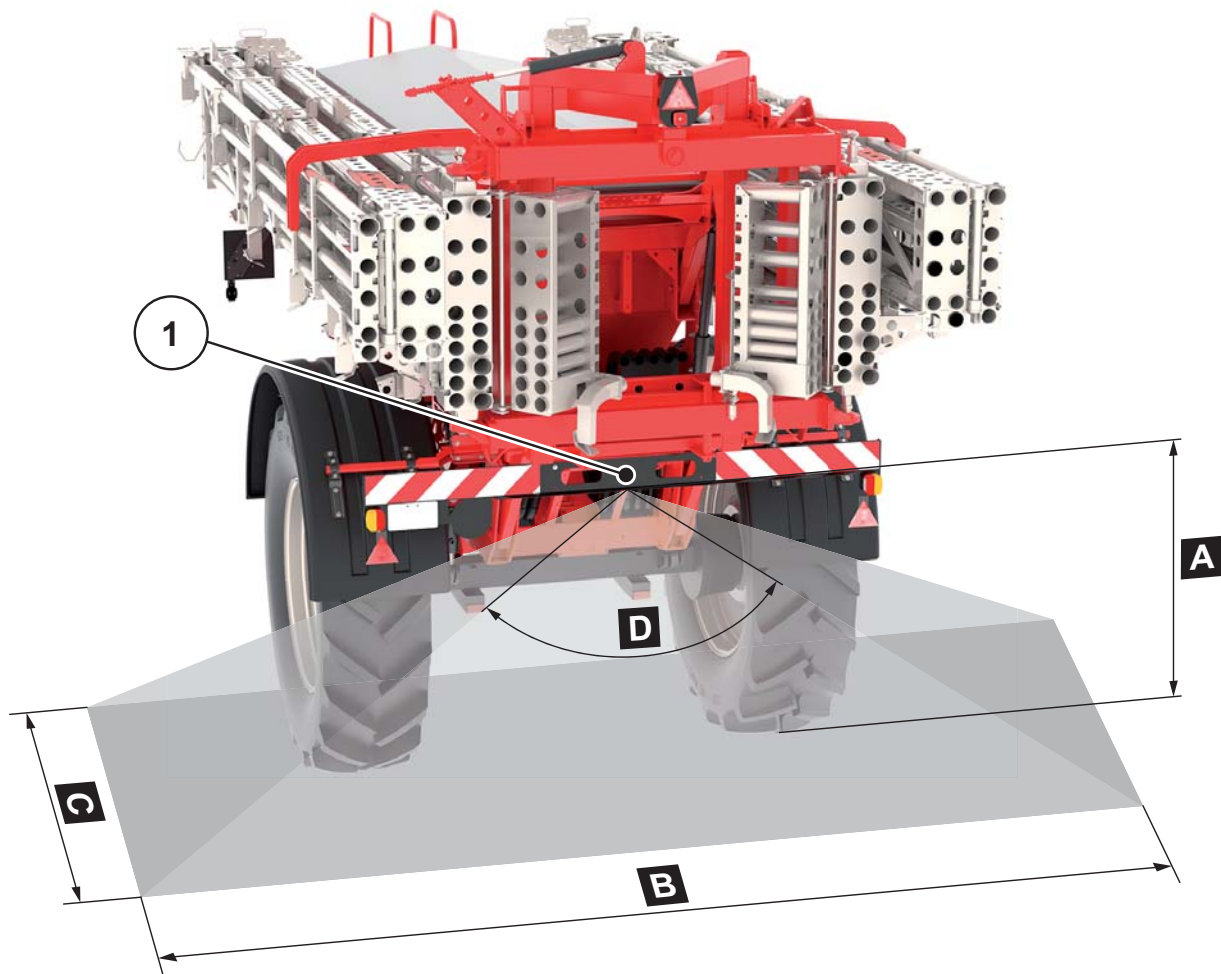
Bild 6.15: Sichtfeld Rückraumkamera
