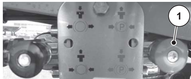
Bild 8.1: Feststellbremse lösen (pneumatische Bremsanlage)
