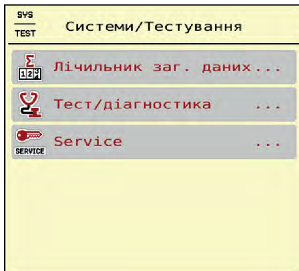
Рис. 17: Меню Система/тестування
