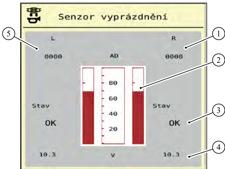
Obr. 21: Test/diagnostika; příklad: Senzor vyprázdnění
