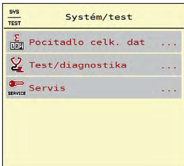
Obr. 17: Menu Systém/test
