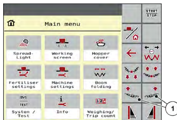
Fig. 16: Funksjonstaster justering utligger-helling
