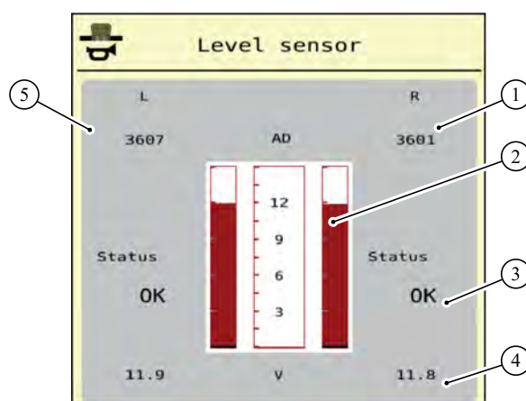
Fig. 19: Test/diagnose, eksempel: Tommeldingssensor
