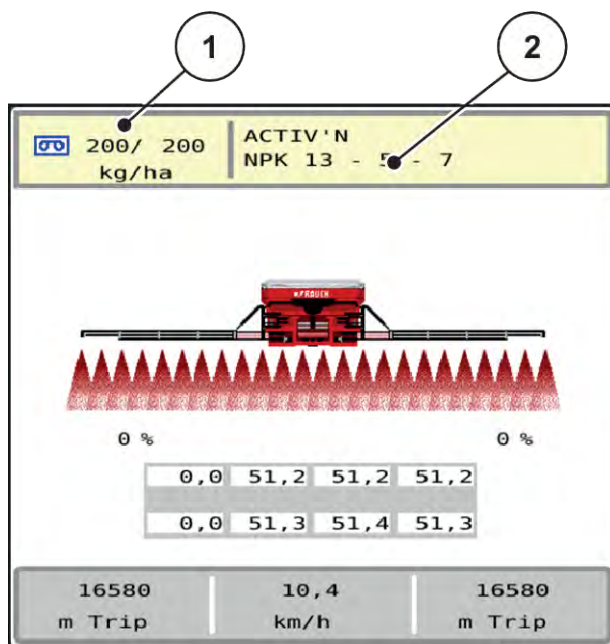
Fig. 11: Håntere spredetabell via berørings skjermen
