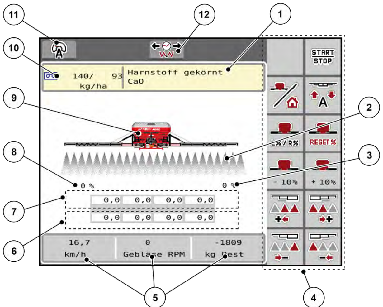
Fig. 1: Displayet på maskinstyringen
