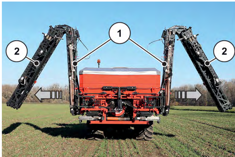
Fig. 15: Klapp ut start- og midtdeler 1
