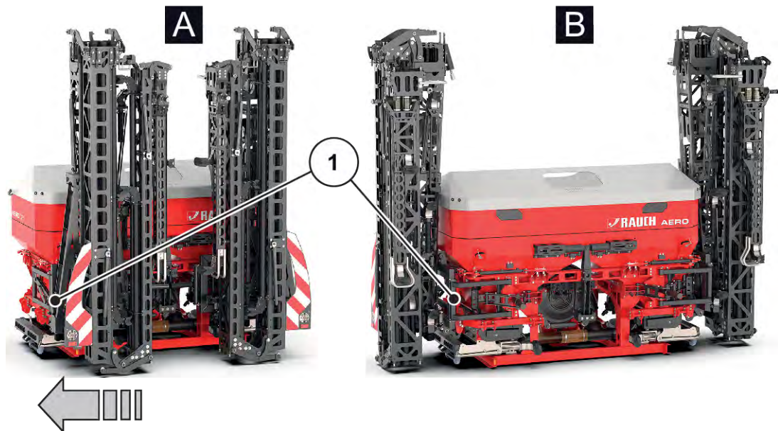
Abb. 43: Schwenkrahmen in Arbeitsposition schwenken
