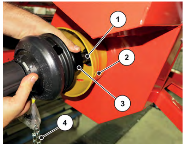
Abb. 24: Gelenkwelle sichern
