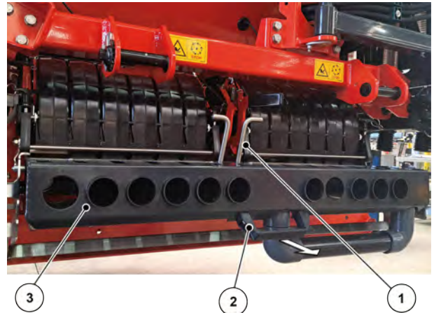
Abb. 52: Injektorkassette entriegeln
