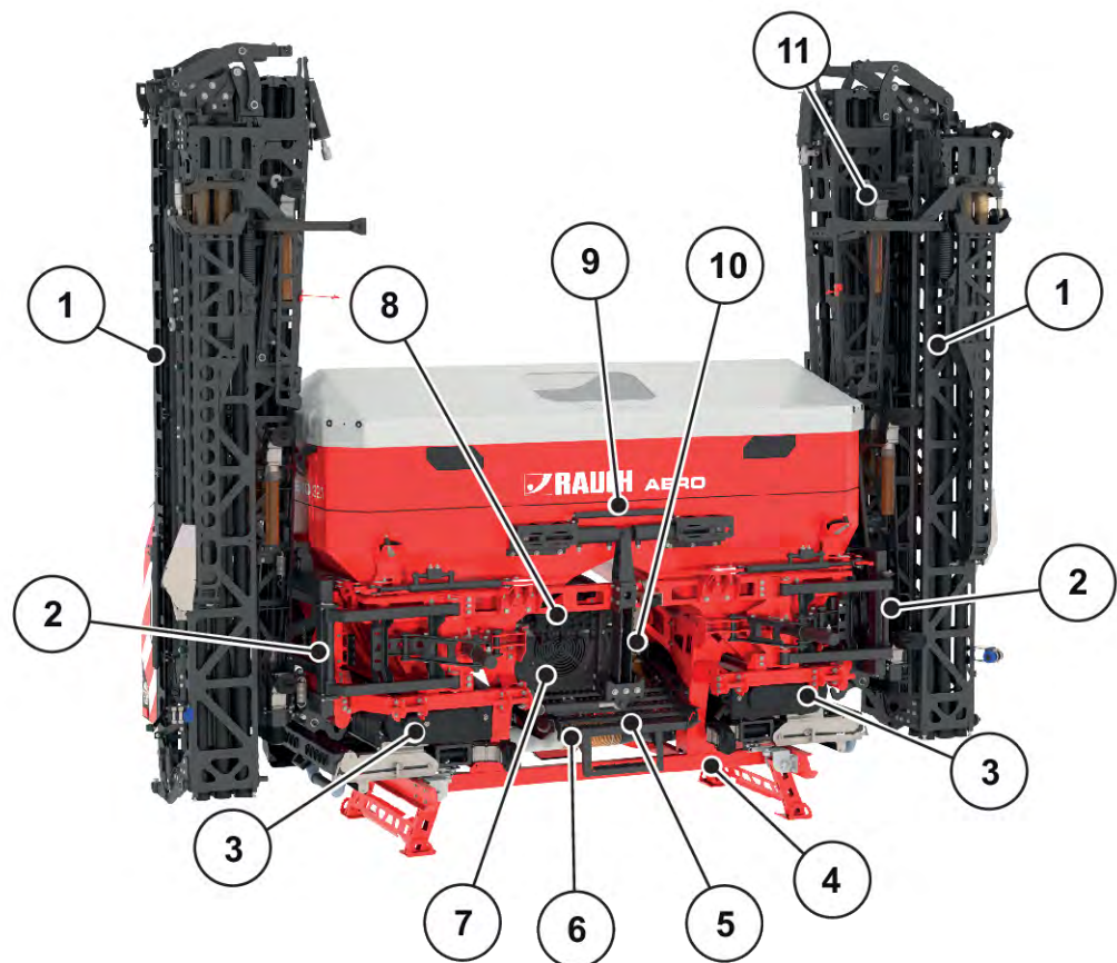
Abb. 7: Baugruppenübersicht: Rückseite
