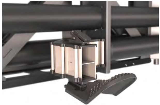
Abb. 50: Prallteller in Spätdüngung
