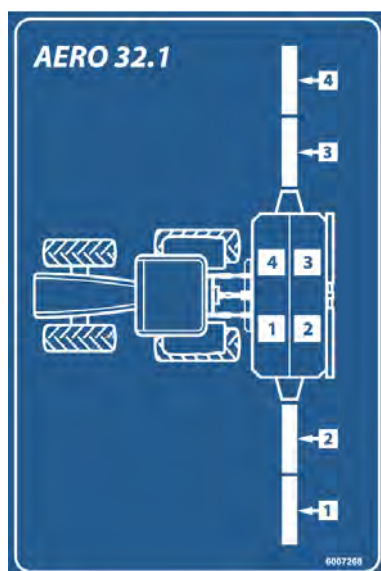
Abb. 32: Darstellung der Teilbreiten am Ausleger-Mineraldüngerstreuer
