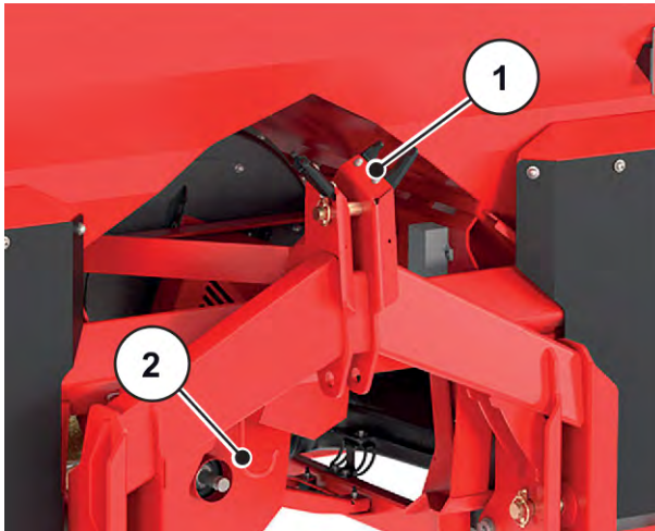
Abb. 55: Ablage der Kabel und Hydraulikschläuche
