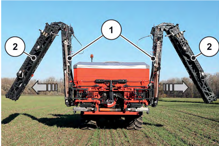
Abb. 45: Anfangs- und Mittelteile 1 ausklappen
