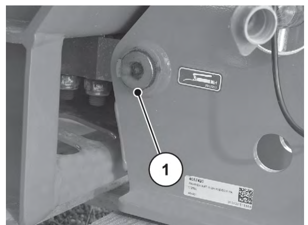
Abb. 65: Schmierstelle Wiegestreuer
