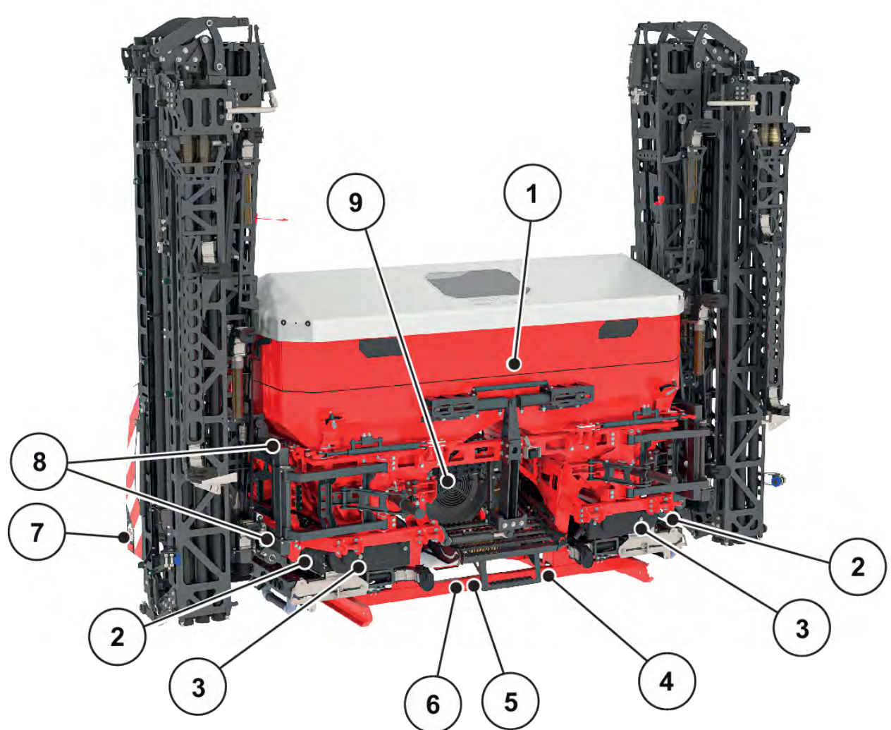
Abb. 3: Schutzeinrichtungen, Aufkleber Warn- und Instruktionshinweise, Rückseite
