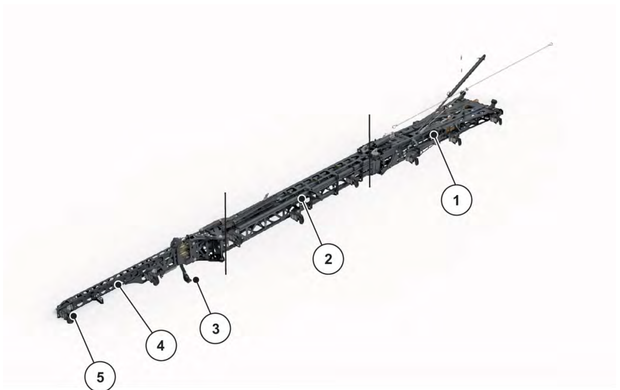
Abb. 12: Baugruppen und Funktionen der Maschine, Ausleger 21 m
