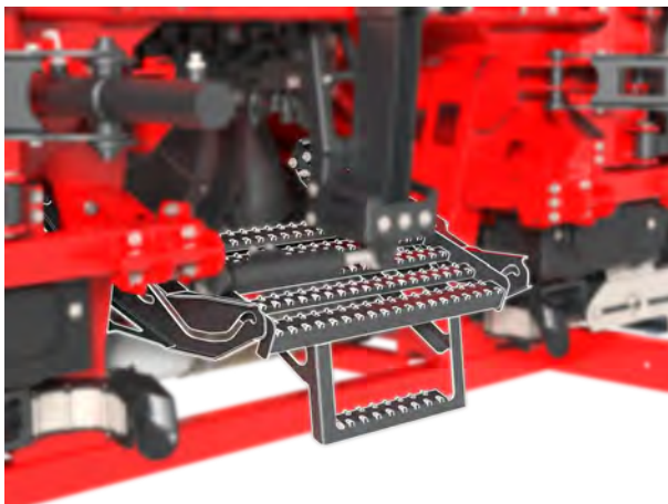
Abb. 29: Aufstieg eingeklappt
