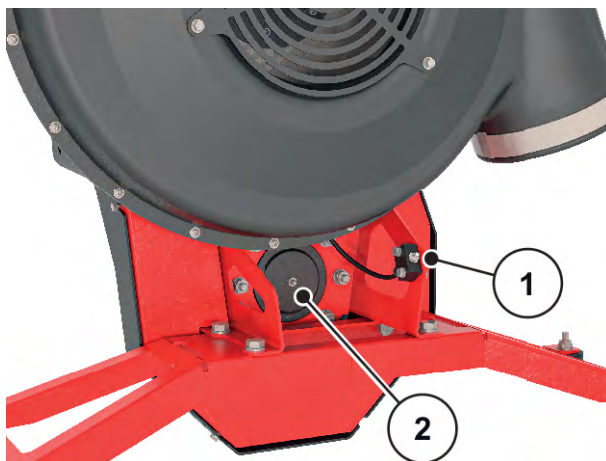
Abb. 66: Schmierstellen Gebläse
