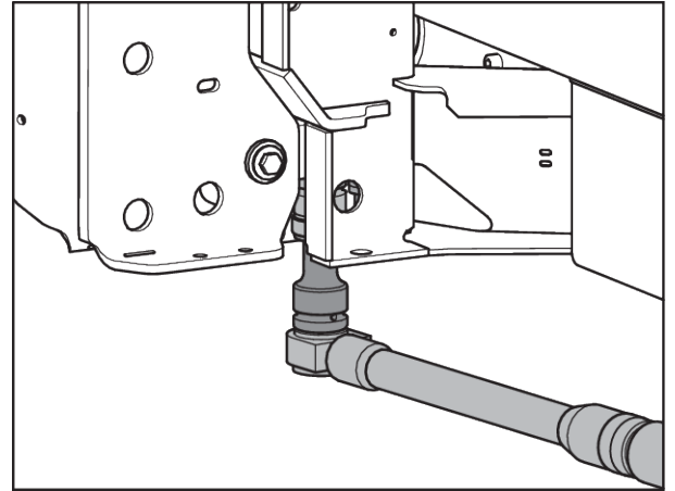
Abb. 57: Befestigung der Wiegezelle (in Fahrtrichtung links)
