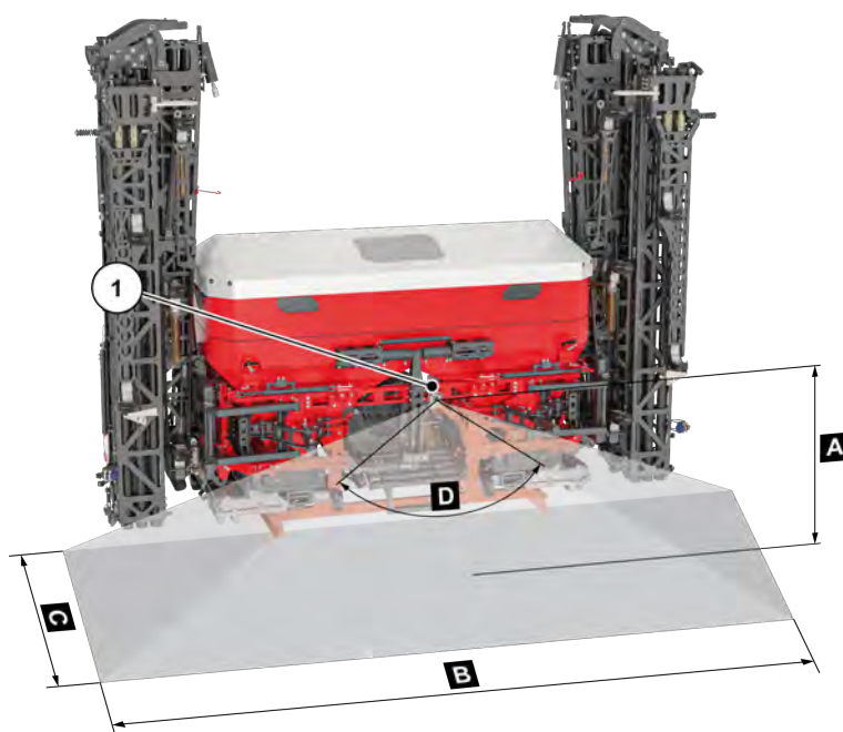
Abb. 18: Sichtfeld Rückraumkamera Maschine in Arbeitsposition
