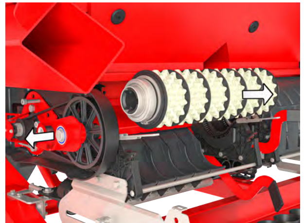
Abb. 41: Halterung Dosierwalze öffnen
