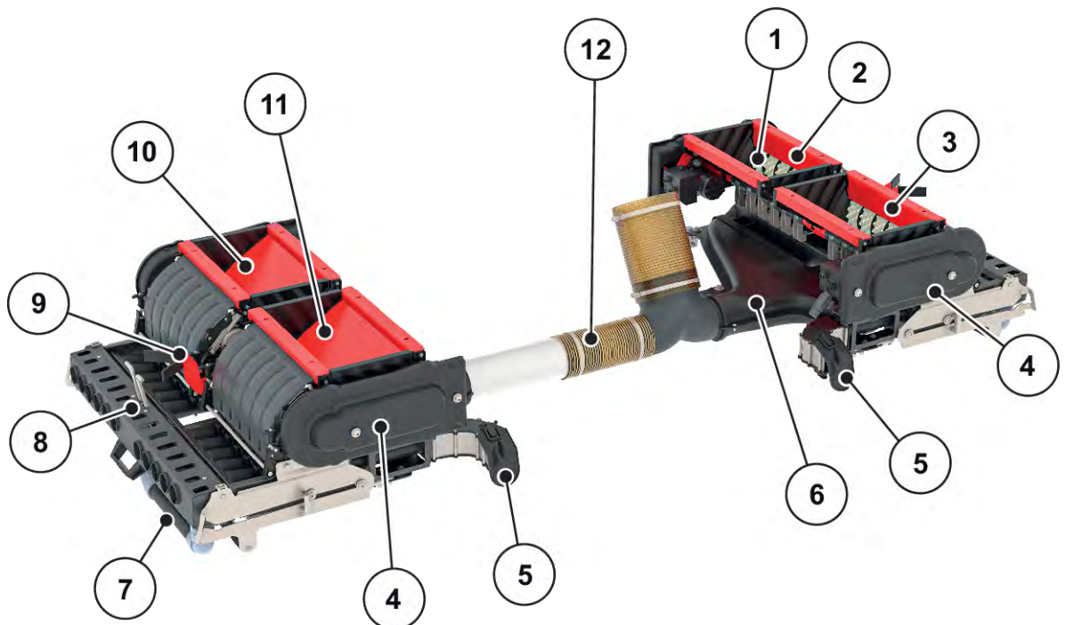
Abb. 10: Baugruppen und Funktion der Maschine, Detail Rückseite
