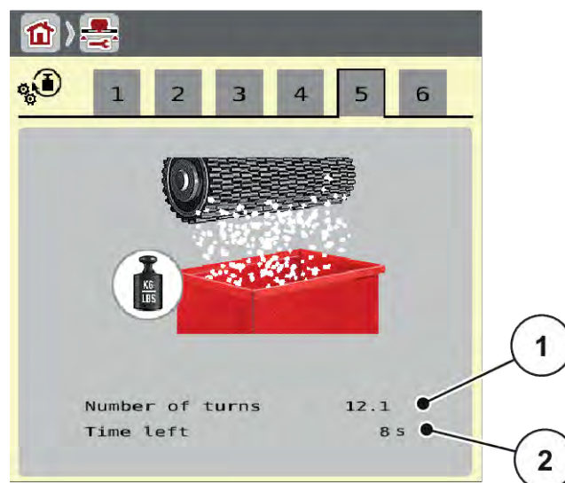
Abb. 36: Menü Abdrehprobe, Seite 5
