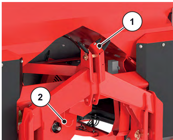
Abb. 25: Ablage der Kabel und Hydraulikschläuche
