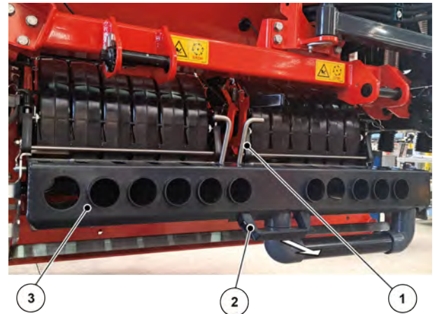
Abb. 33: Injektorkassette entriegeln
