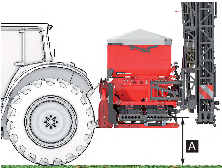
Abb. 28: Optimale Anbauhöhe in der Normal- und Spätdüngung
