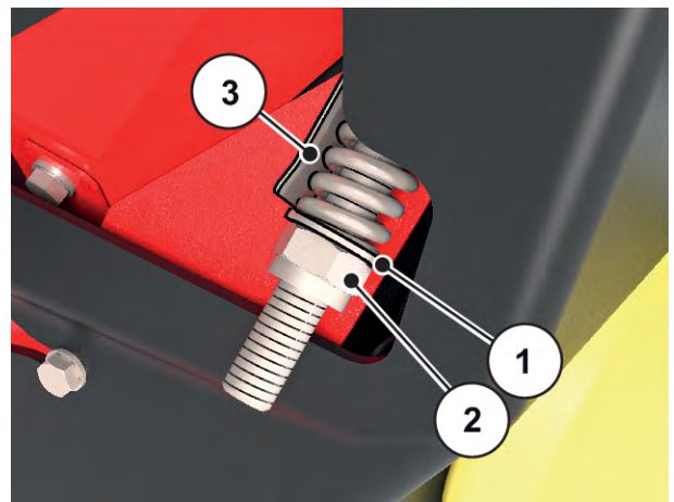
Abb. 63: Nachspannvorrichtung des Gebläseriemens
