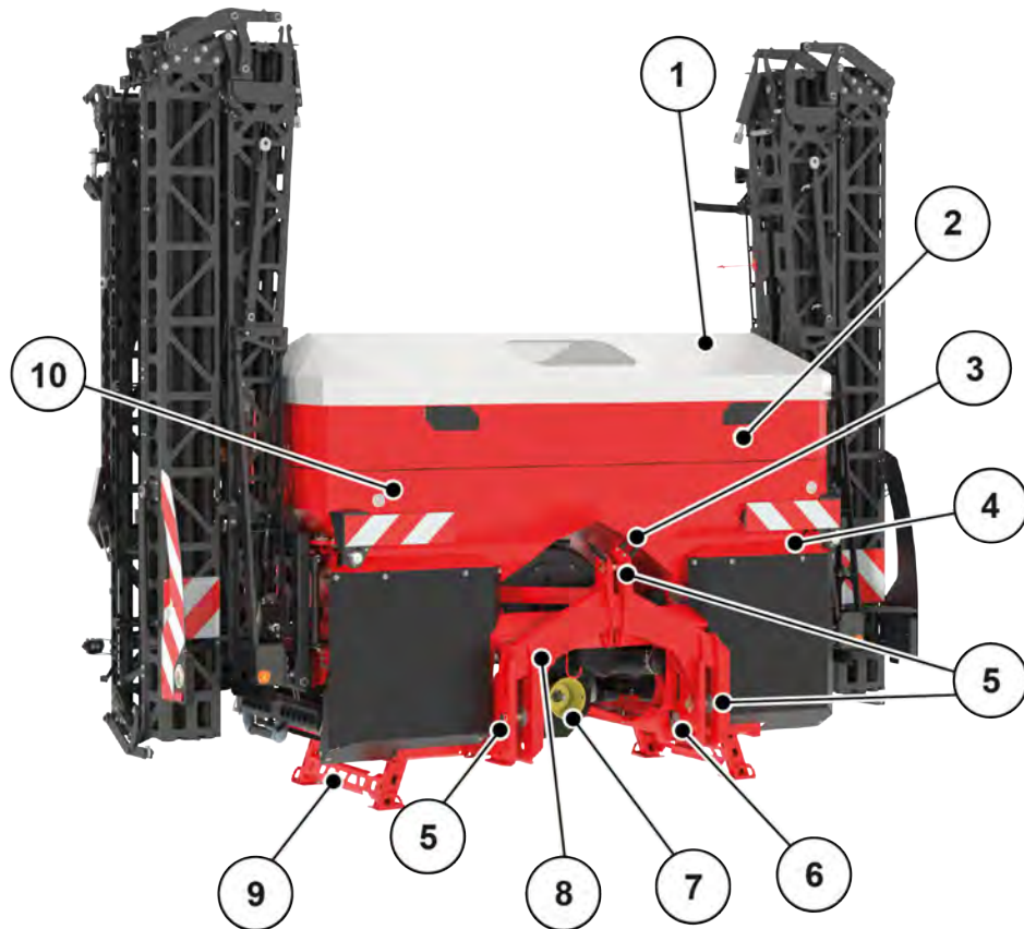
Abb. 6: Baugruppenübersicht: Vorderseite
