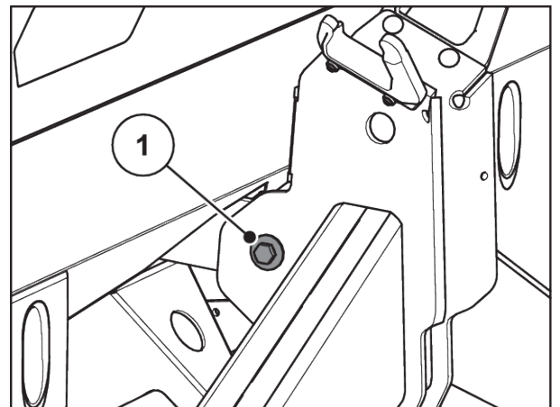
Abb. 58: Befestigung des Zugstabes am Wiegerahmen
