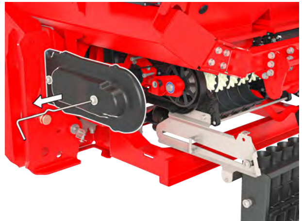
Abb. 39: Riemenabdeckung entfernen
