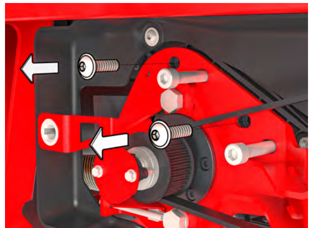
Abb. 40: Schrauben am Motor lösen
