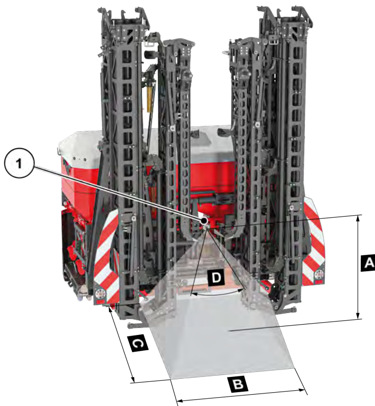
Abb. 17: Sichtfeld Rückraumkamera Maschine in Transportposition
