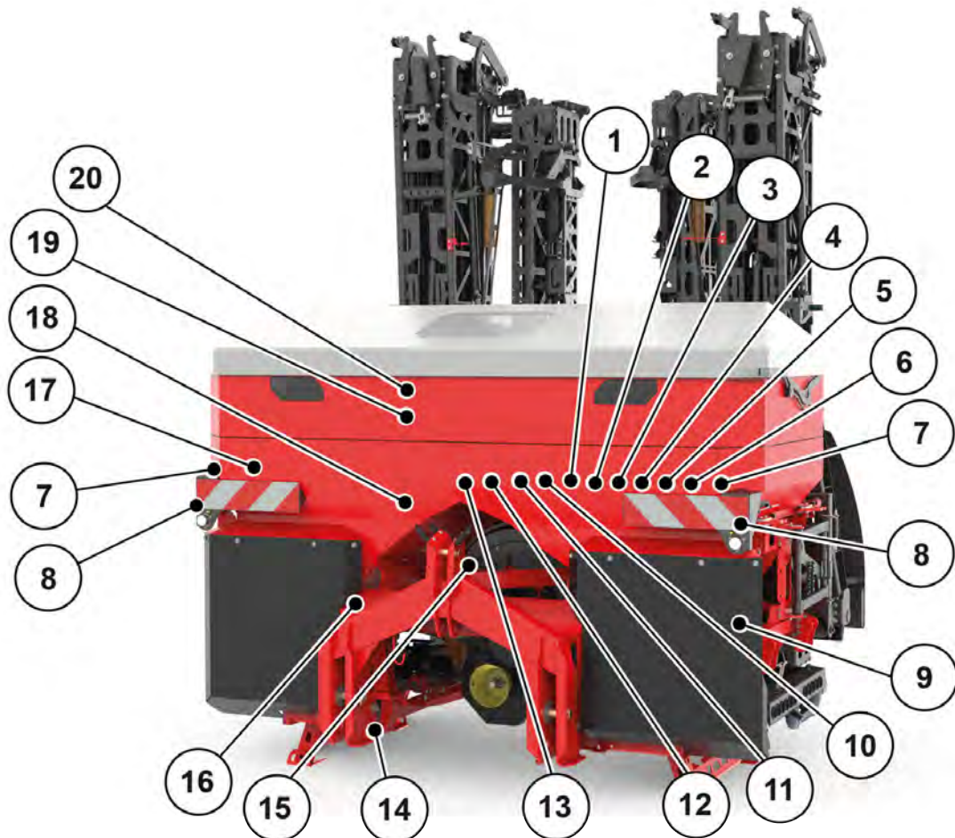
Abb. 2: Schutzeinrichtungen, Aufkleber Warn- und Instruktionshinweise, Vorderseite
