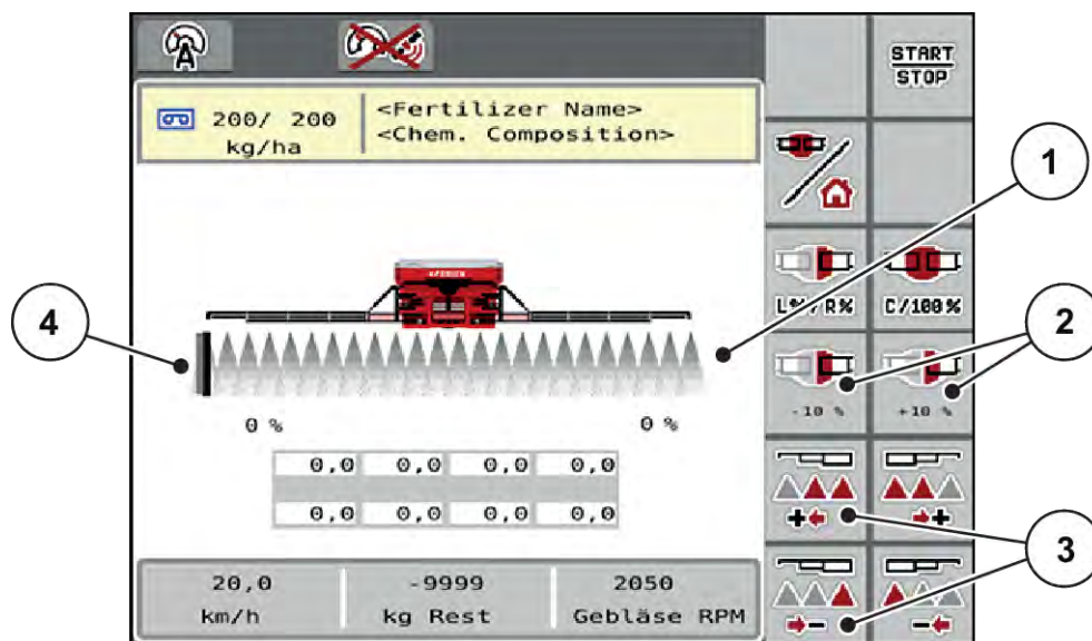
Att. 32: Darba ekrāns ar aktivizētu daļējo platumu, izkliešana gar robežu kreisajā pusē
