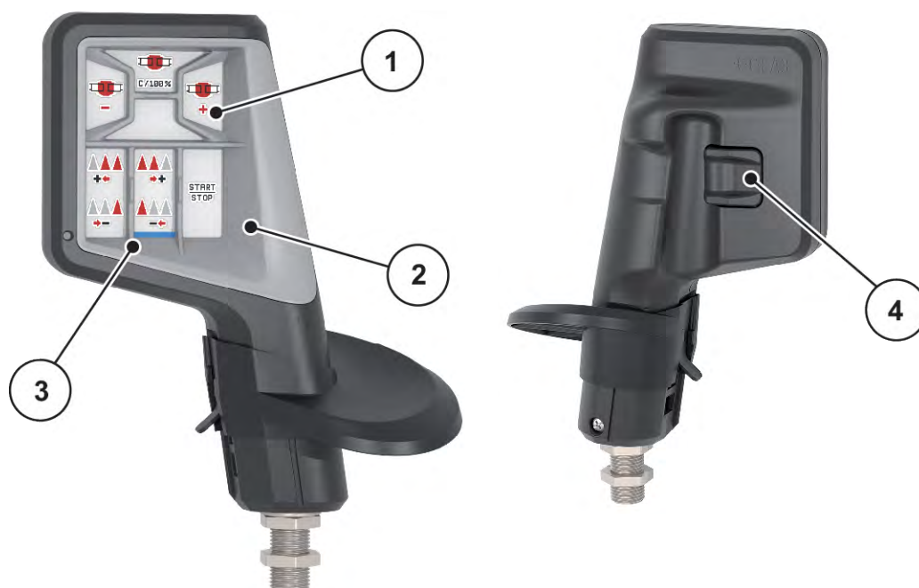
Att. 27: CCI A3 kursorsvira, priekšpuse un aizmugure
