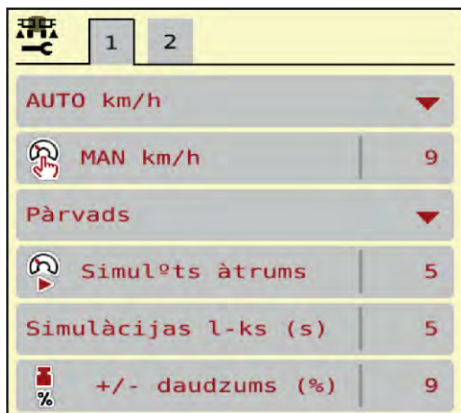
Att. 12: Izvēlne Mašīnas iestatījums
