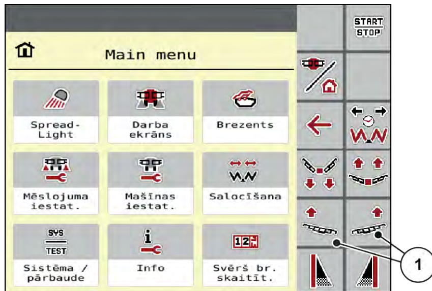
Att. 15: Funkciju taustiņi Strēles slīpuma regulēšana
