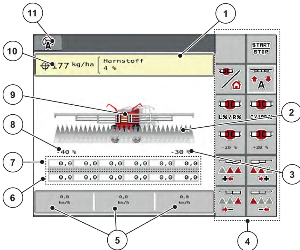
Ábr. 1: A vezérlőegység kijelzője
