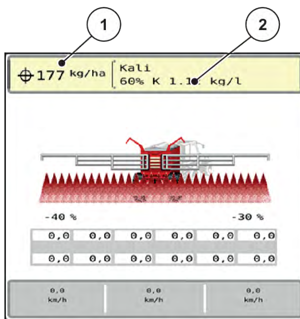
Ábr. 8: Kihordott mennyiség megadása az érintőképernyőn
