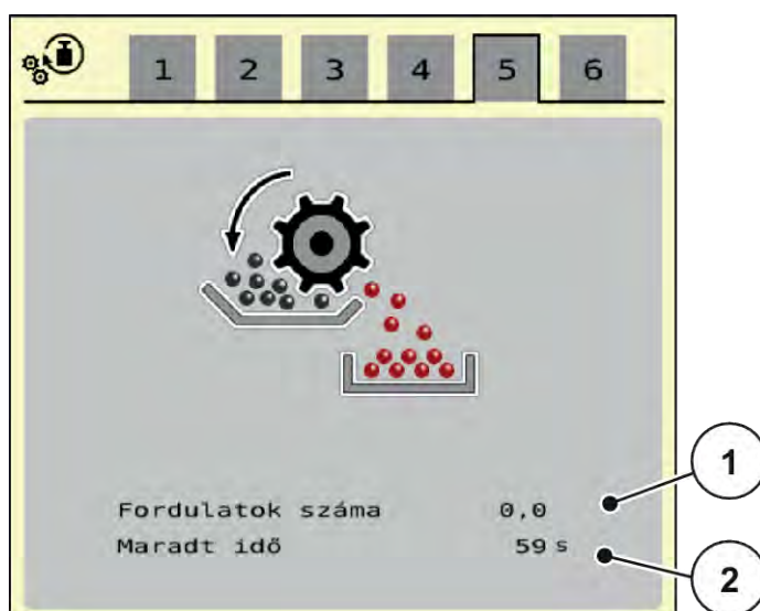
Ábr. 10: Leforgatási próba menü, 5. oldal
