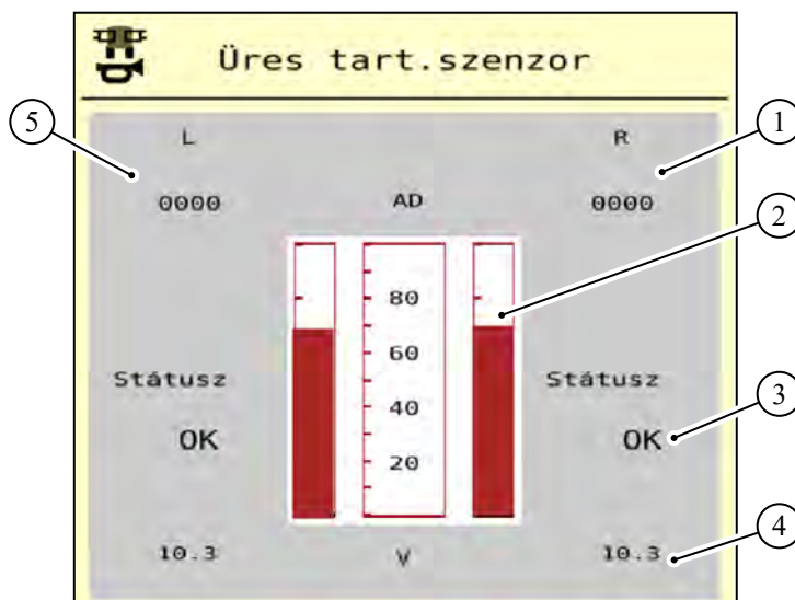
Ábr. 22: Teszt/diagnózis; példa: Üres tart.szenzor
