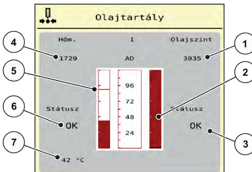
Ábr. 20: Teszt/diagnózis; példa: Olajtartály
