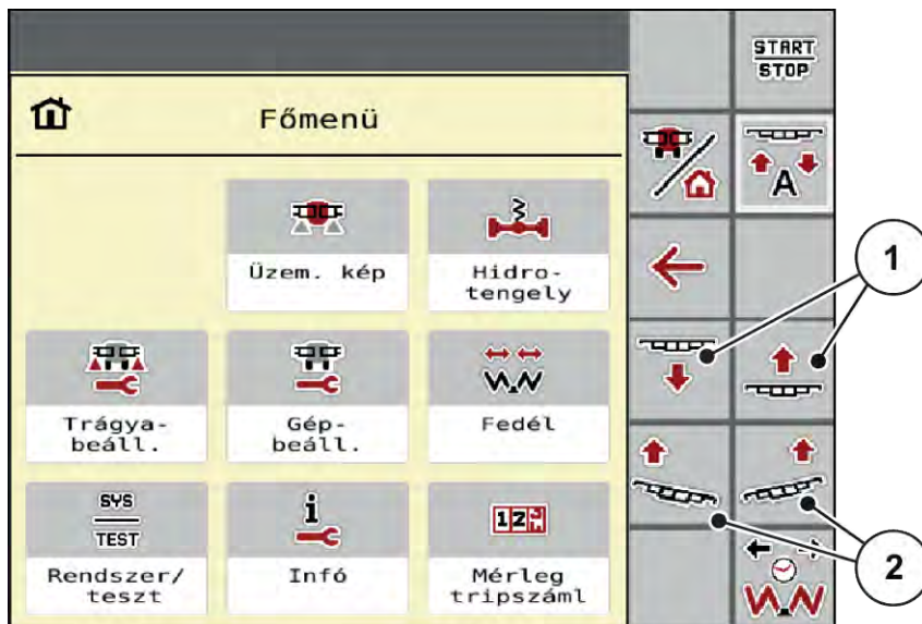
Ábr. 17: Gémdőlés/-magasság állítása funkciógombok
