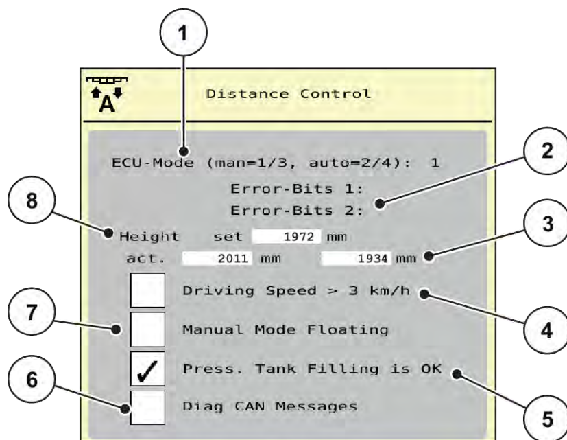
Ábr. 23: Teszt/diagnózis; példa: Távvezérlés
