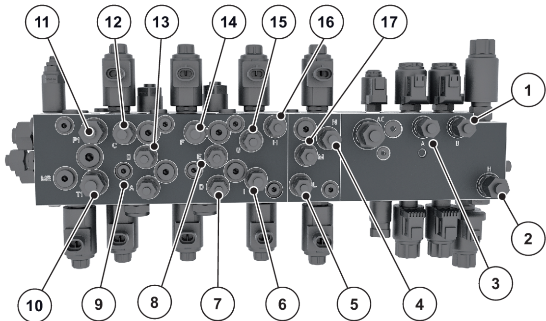
Fig. 17: Aperçu du raccordement du bloc de commande
