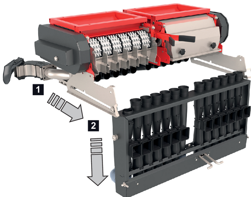
Fig. 35: Descente de la cassette de l'injecteur
