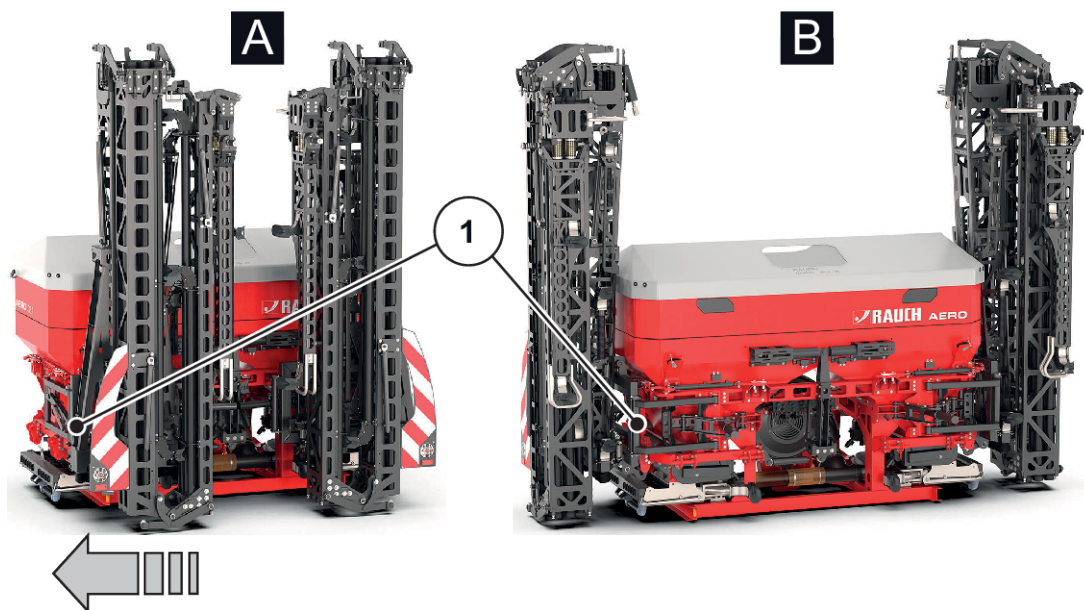
Fig. 25: Pivotement du châssis pivotant en position de travail
