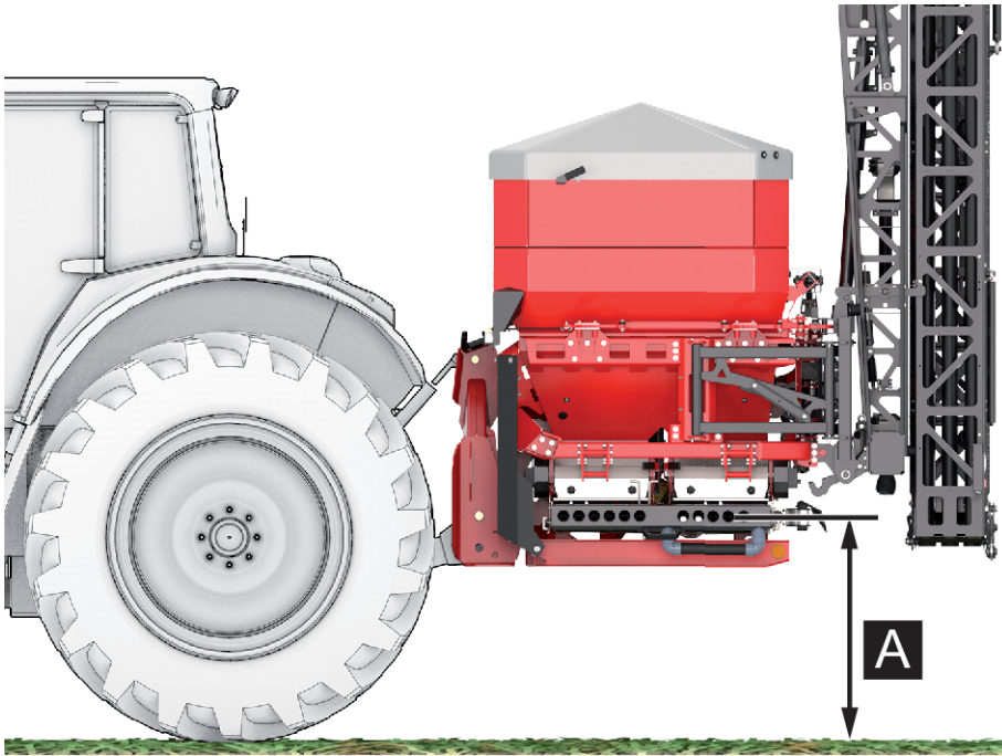
Fig. 15: Position de montage
