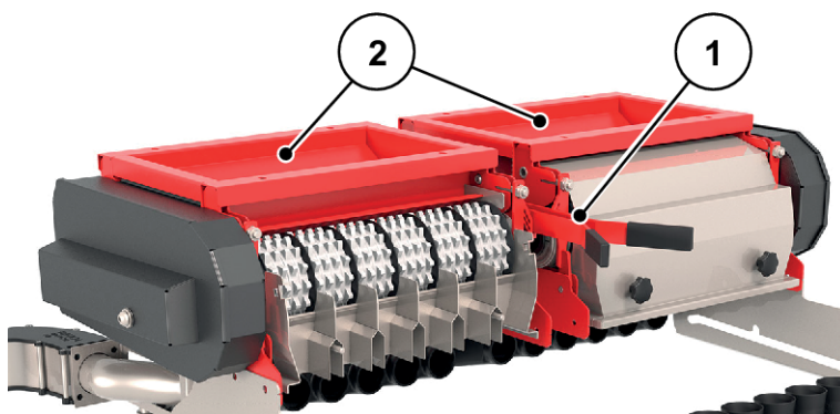
Fig. 36: Ouverture de la cuve de dosage
