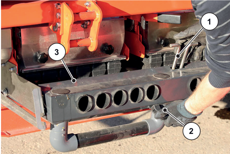
Fig. 20: Déverrouillage de la cassette de l'injecteur
