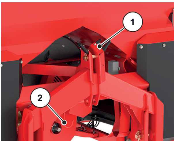
Fig. 14: Rangement des câbles et des tuyaux hydrauliques
