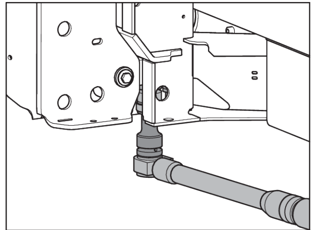
Fig. 39: Fixation des pesons (à gauche dans le sens d'avancement)
