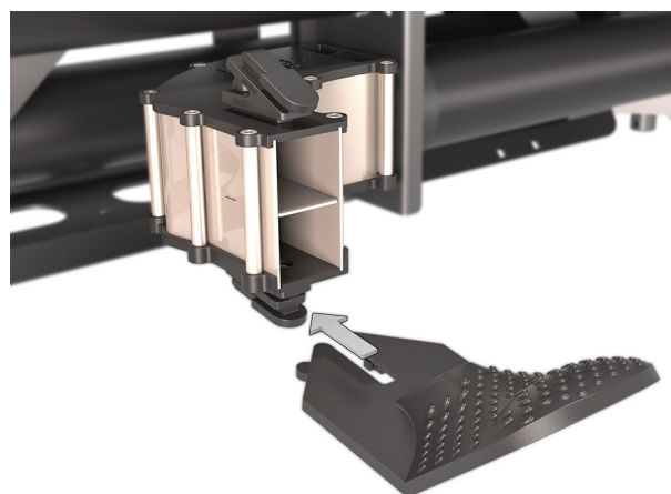
Fig. 31: Changement de position du déflecteur
