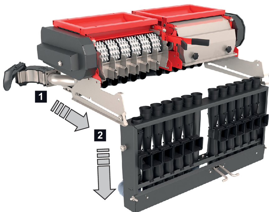
Fig. 21: Descente de la cassette de l'injecteur
