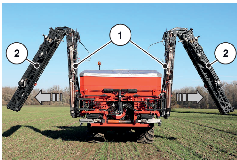
Fig. 27: Déplier les sections initiales et centrales 1
