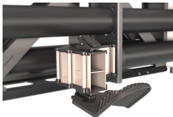
Fig. 32: Déflecteur en position d'épandage tardif
