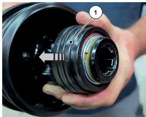
Fig. 12: Repousser le manchon coulissant
