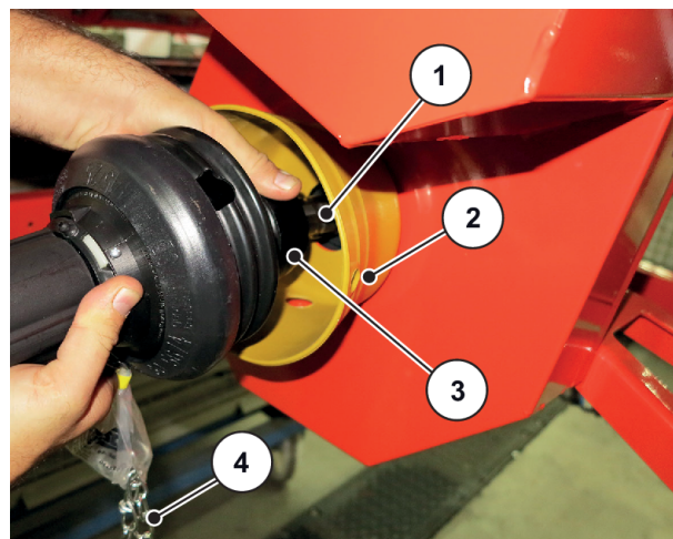
Fig. 13: Blocage de l'arbre de transmission
