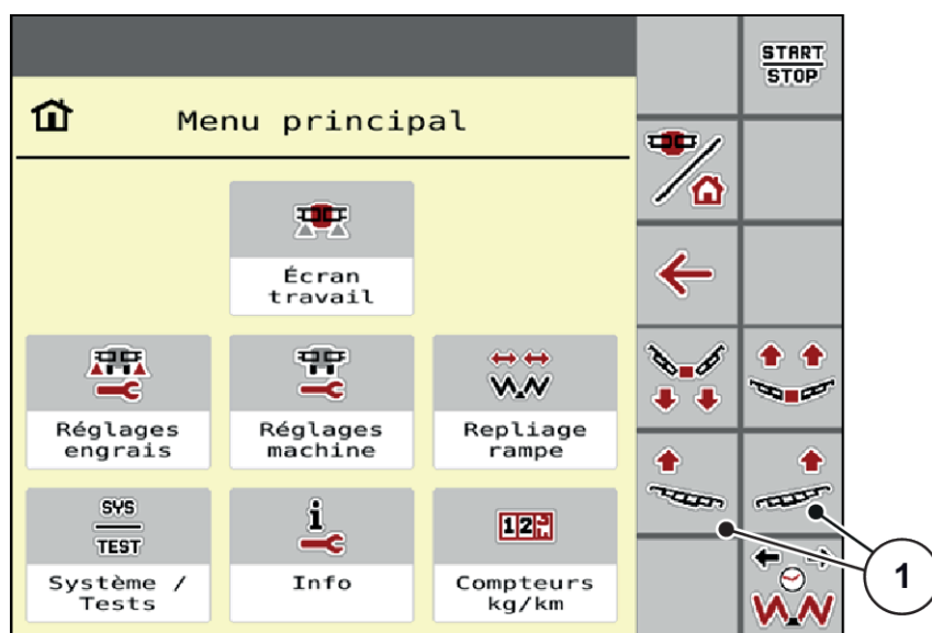
Fig. 28: Touches de fonction Réglage de l'inclinaison de la rampe
