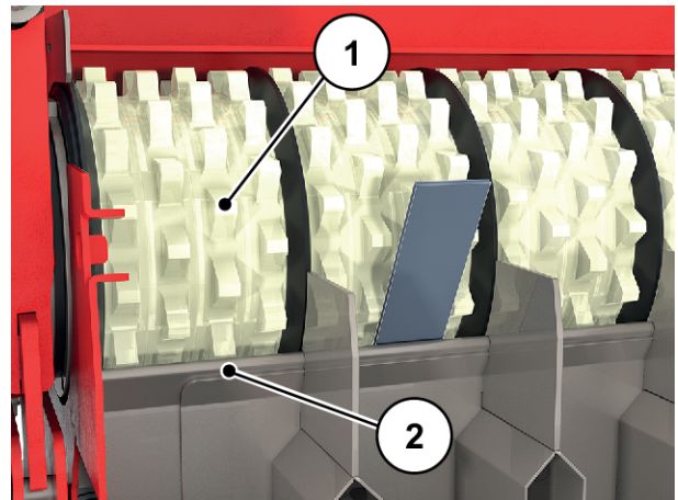
Fig. 45: Distance des roues à came - vérification de la cuve d'épandage
