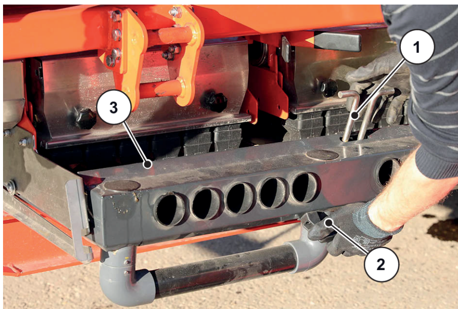
Fig. 34: Déverrouillage de la cassette de l'injecteur
