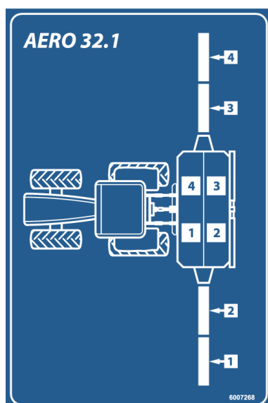
Fig. 19: Représentation de la largeur partielle sur le distributeur à balancier pour engrais minéral
