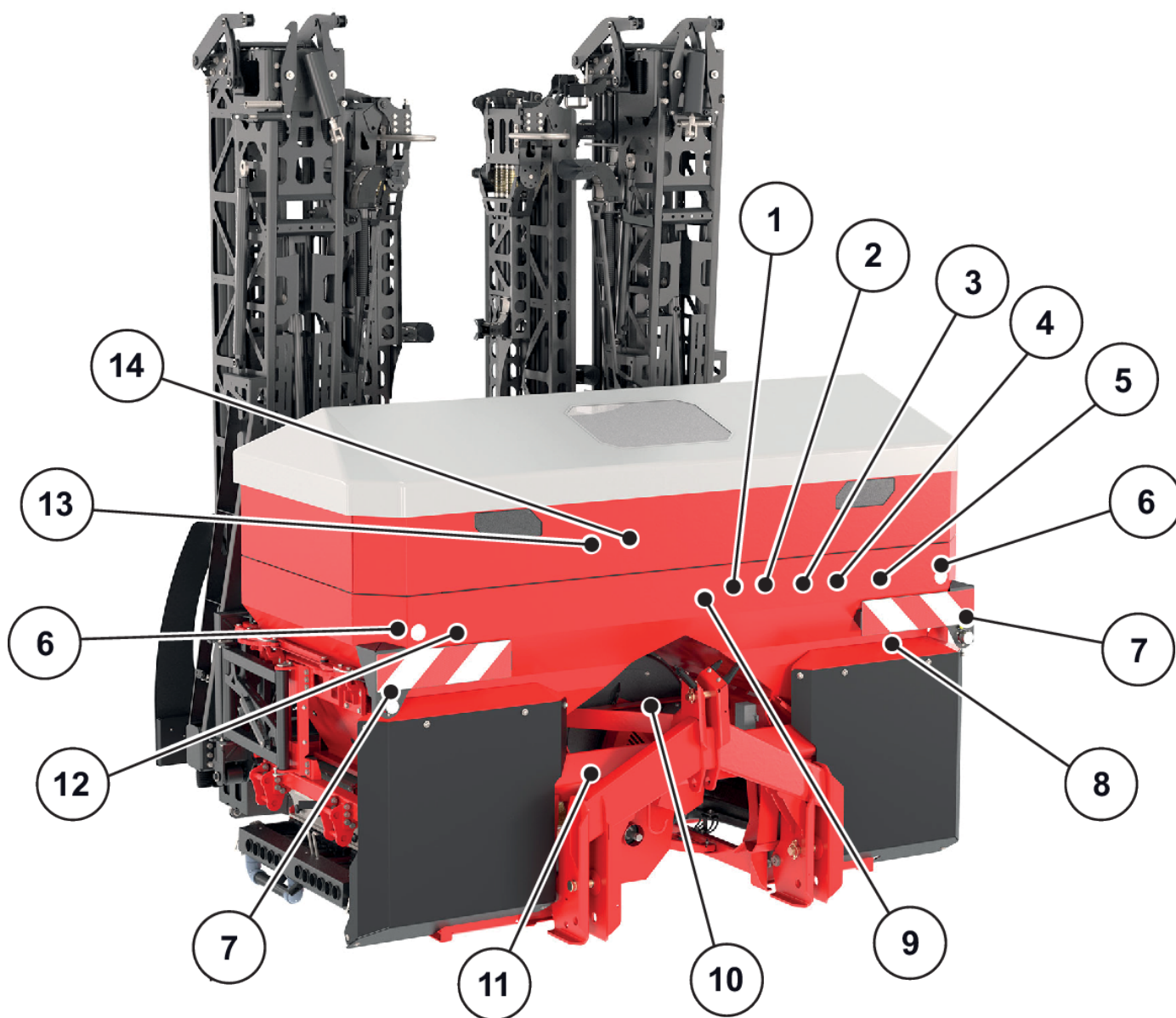
Fig. 2: Dispositifs de protection, autocollants de consignes de sécurité et d'instructions, face avant
