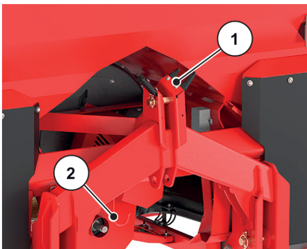
Fig. 38: Rangement des câbles et des tuyaux hydrauliques
