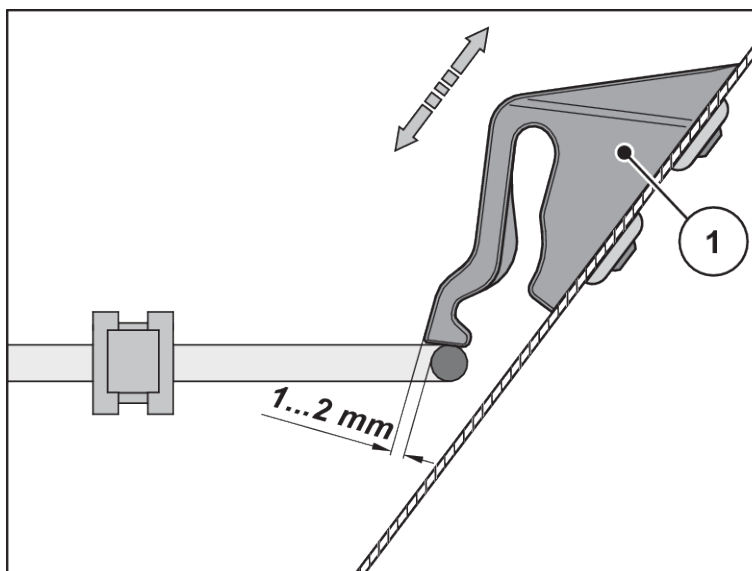
Fig. 43: Mesure de référence pour le contrôle de fonctionnement du blocage de la grille de protection
