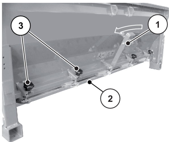
Ábr. 17: A műtrágyaszóró gyorsleürítése UKS GB, lazítsa meg a csillagfogantyúkat
