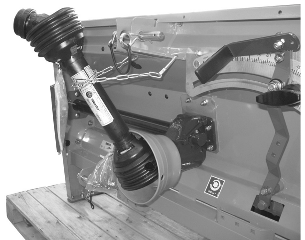
Ábr. 11: Kardántengely felakasztása
