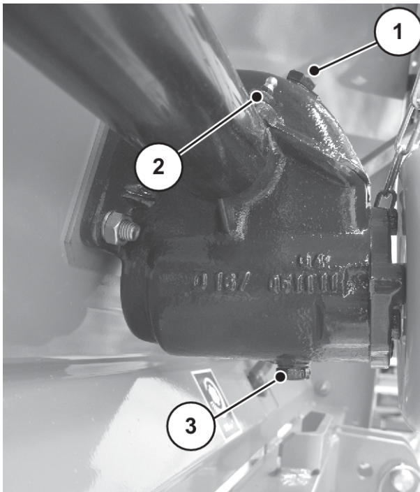
Ábr. 20: Hajtóműolaj betöltési és leeresztési helyei
