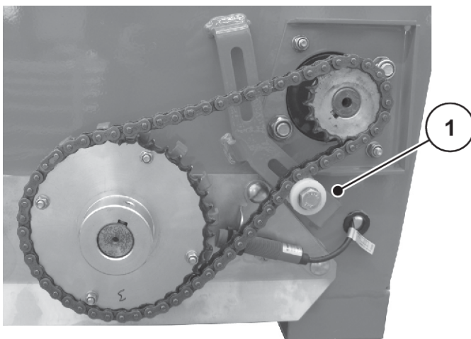
Fig. 5: Montage du rouleau tendeur de chaîne (prise de force tournant à droite)
