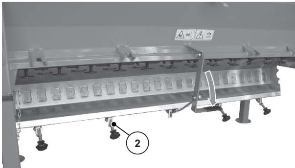
Fig. 18: Vidange rapide, épandeur d'engraisUKS GB, faire pivoter le fond de la cuve d'épandage vers le bas
