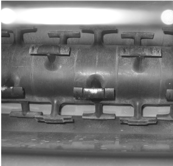
Fig. 19: Vérifier l'absence d'usure sur les doigts d'agitation
