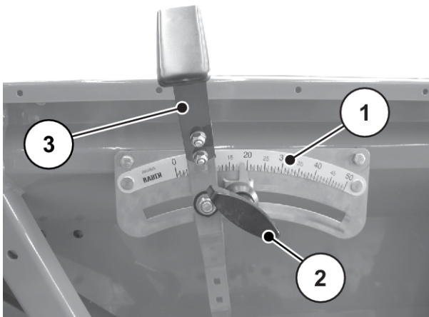
Fig. 15: Réglage des vannes de dosage
