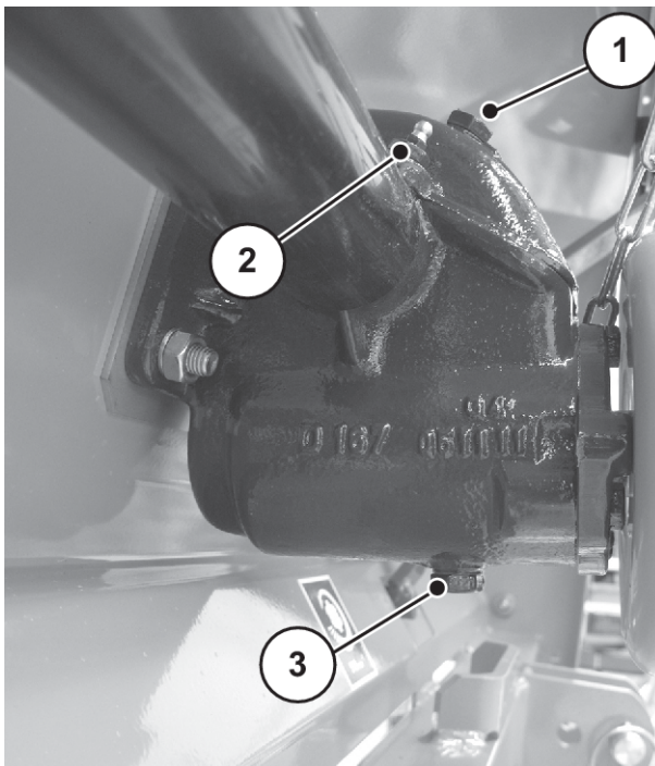
Fig. 20: Påfyllnings- och avtappningsställen för växellådsolja
