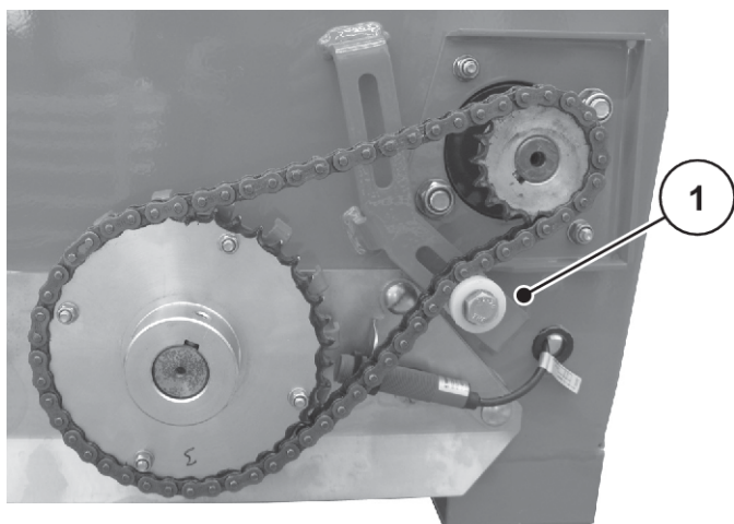
Fig. 5: Montering spännrulle (högerroterande kraftuttagsdrivning)
