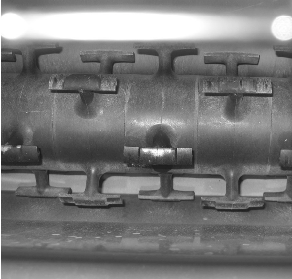
Fig. 19: Kontroll av omrörarfingret avseende slitage
