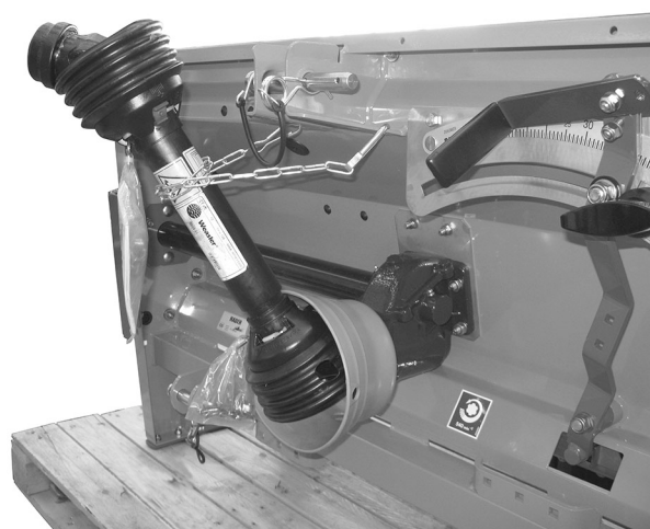
Fig. 11: Upphängning av kraftöverföringsaxeln
