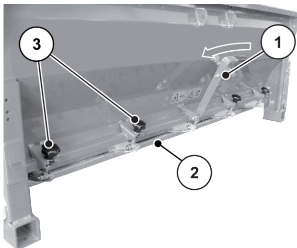
Fig. 17: Hurtigtømning af gødningsspreder UKS GB, løsning af stjernegreb
