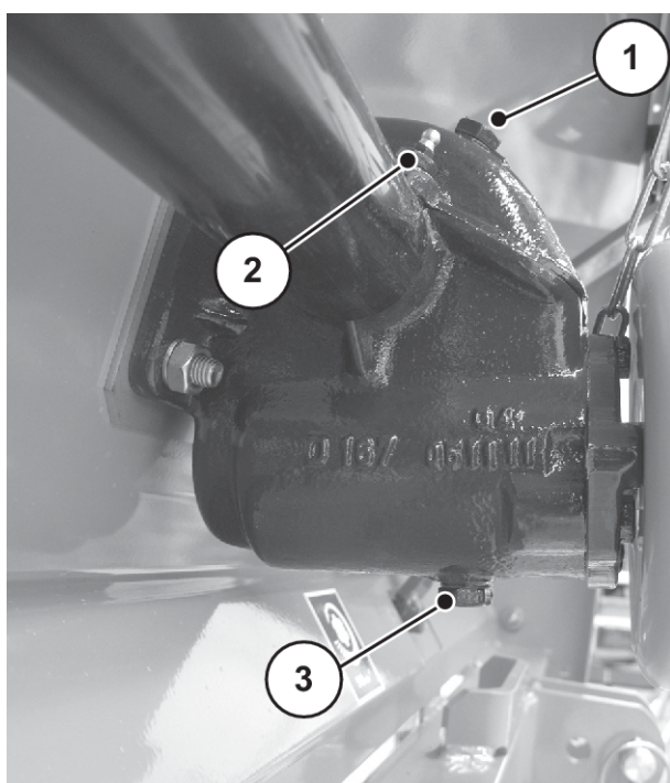
Fig. 20: Påfyldnings- og aftapningssteder til gearolie
