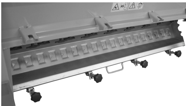
Fig. 16: Hurtigtømning UKS 80 til UKS 120
