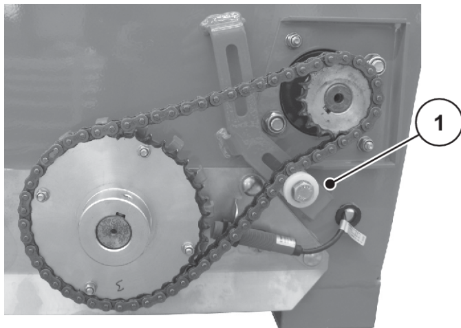
Fig. 5: Montering af kædestrammerulle (højreroterende kraftudtag)
