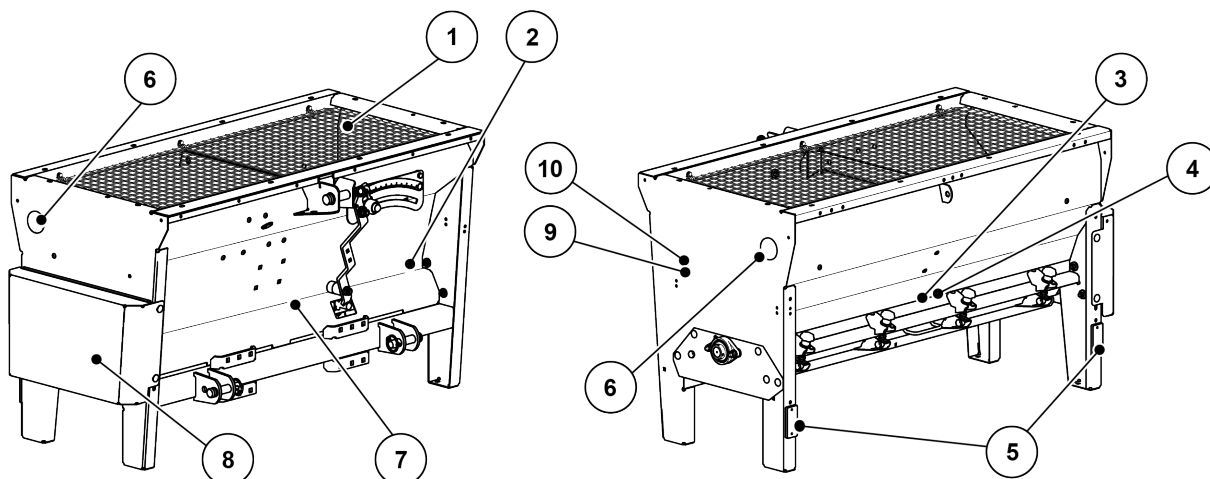
Fig. 1: Beskyttelsesanordninger samt advarsels- og instruktionsmærkater
