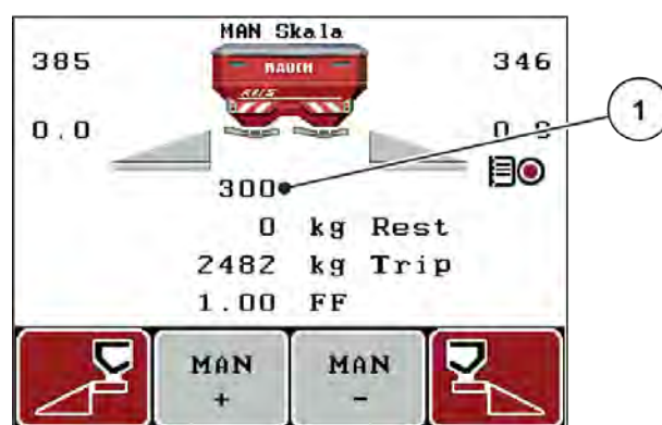
Рис. 35: Робочий екран ВРУЧНУ шкала
