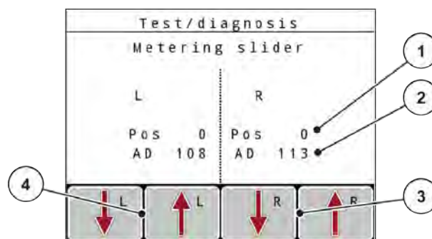
Рис. 43: Тестування/діагностика; приклад: Заслінка дозатора
