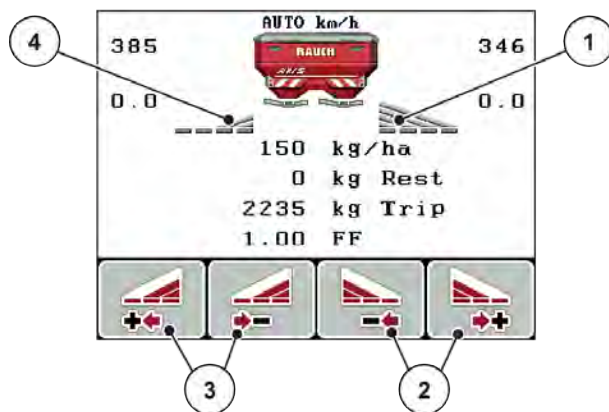
Рис. 51: Робочий екран режиму внесення добрива за допомогою секцій штанги
