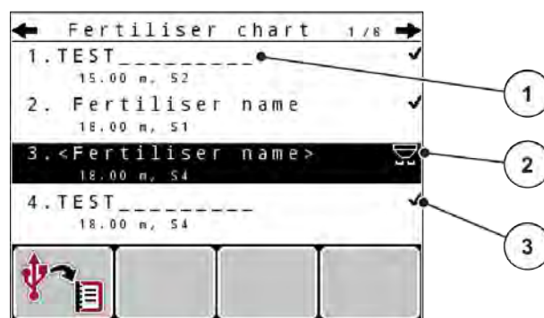
Рис. 29: Меню Таблиця дозування
