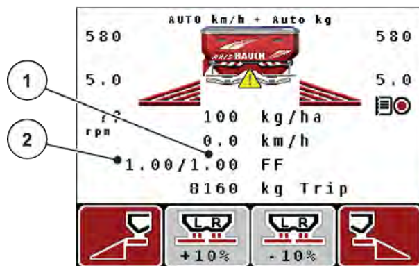
Рис. 27: Окреме регулювання коефіцієнта текучості ліворуч та праворуч (активна функція M EMC)
