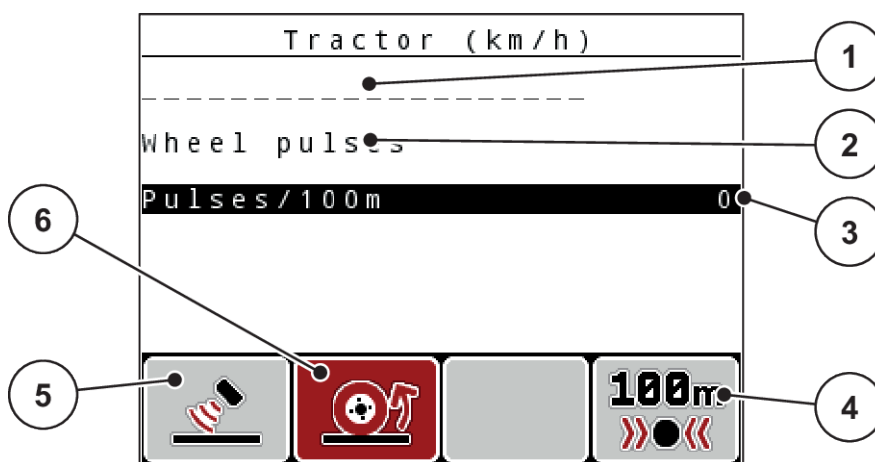
Рис. 33: Меню калібрування «Трактор, км/год»
