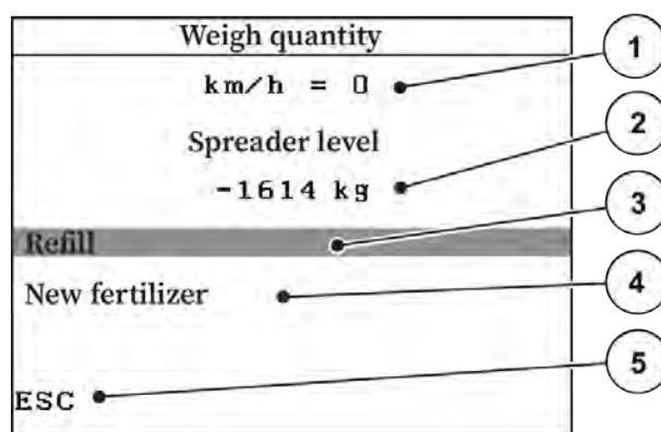
Рис. 20: Меню «Зважити кількість»
