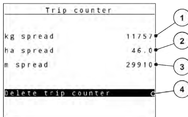
Рис. 18: Меню «Лічильник шляху»
