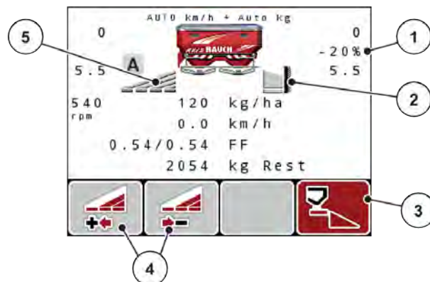
Рис. 53: Робочий екран: секція штанги ліворуч, сторона внесення добрива на межі праворуч
