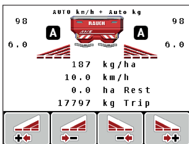
図 56: 操作画面の表示:GPS コントロールを用いた肥料散布
