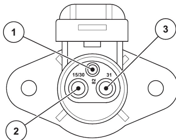
図 9: 電源ソケットのピン配置
