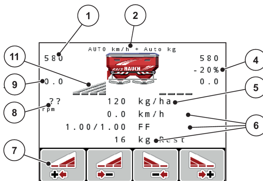
Фиг. 4: Дисплей на блока за управление - пример работен екран AXIS-M EMC
