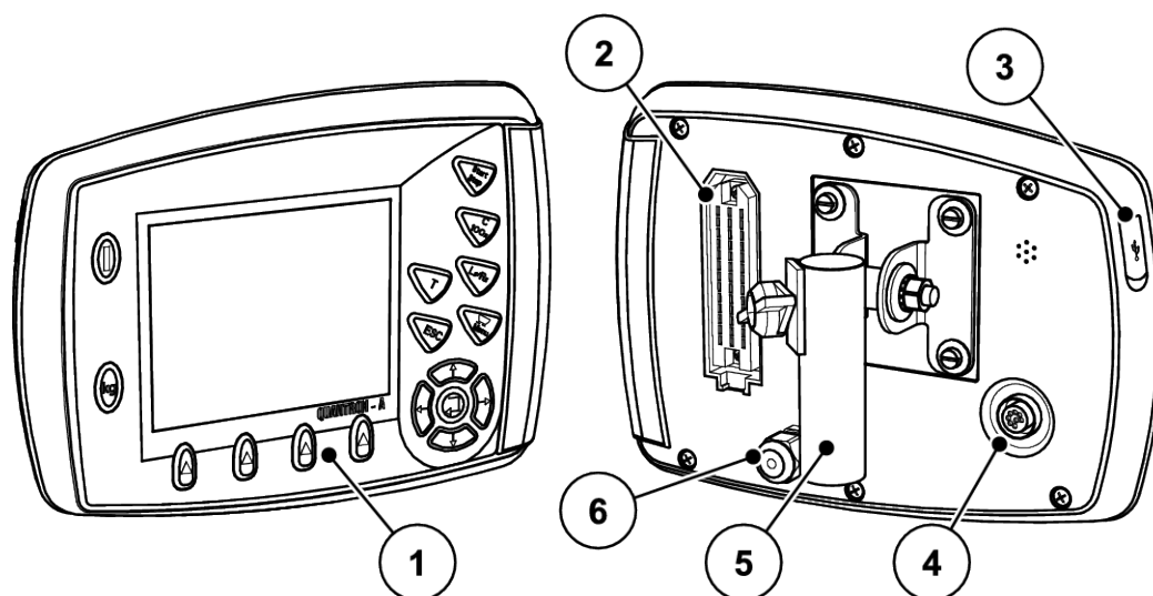
Ilust. 1: Unidad de control QUANTRON-A
