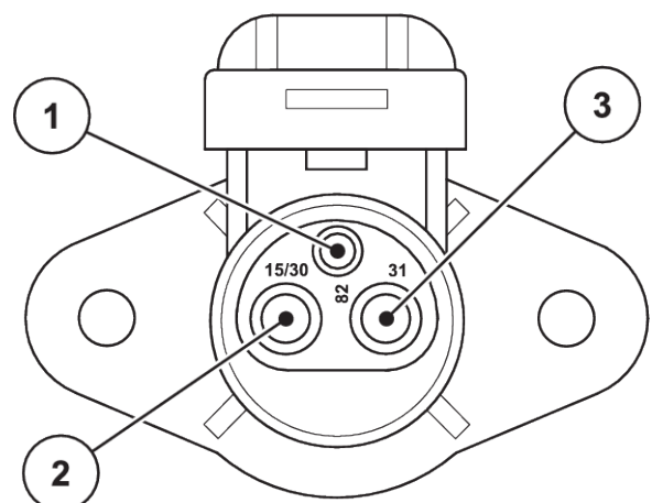
Abb. 9: PIN-Belegung Stromsteckdose
