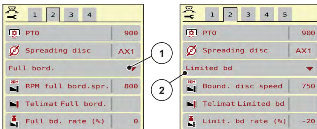
Σχ. 10: Τιμές ρύθμισης λειτουργίας διασκορπισμού ορίων
