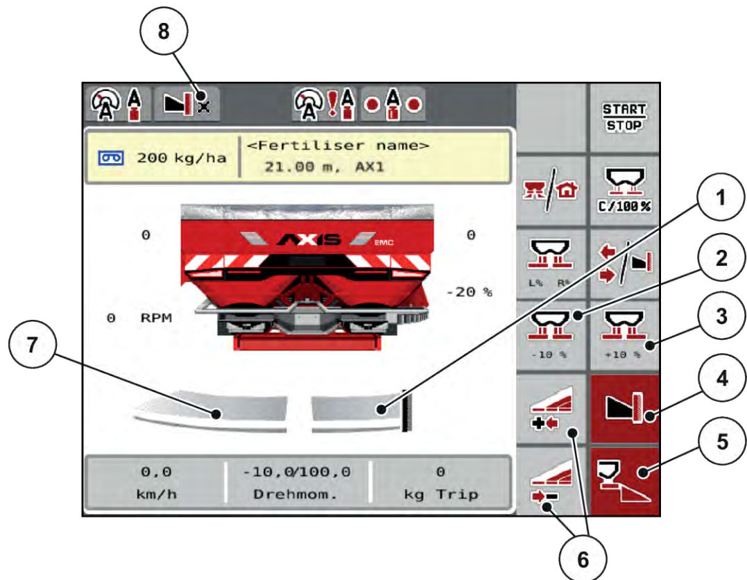
Σχ. 29: Οθόνη λειτουργίας με τμηματικό εύρος αριστερά, πλευρά διασκορπισμού ορίων δεξιά
