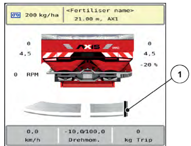
Σχ. 26: Ένδειξη TELIMAT X
