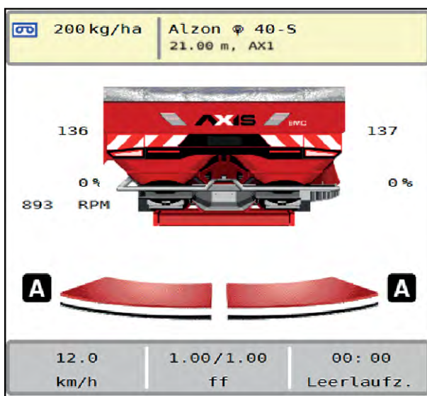
Σχ. 32: Ένδειξη λειτουργίας διασκορπισμού με GPS-Control στην οθόνη λειτουργίας
