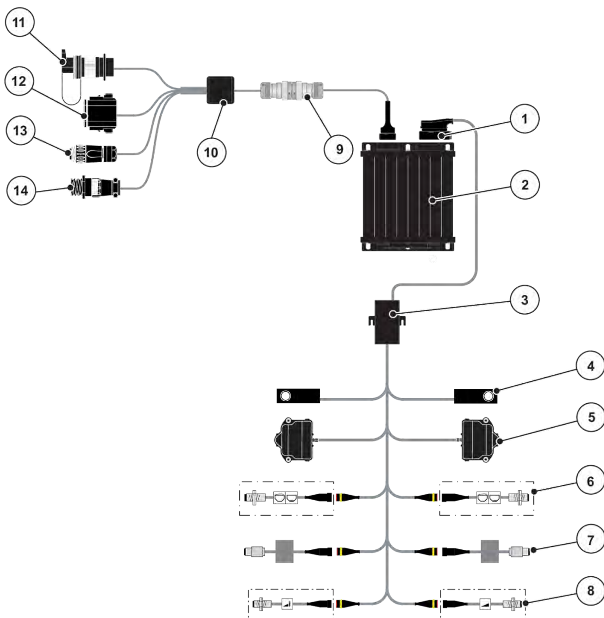
Fig. 6: AXIS 25: Aperçu schématisé du raccordement
