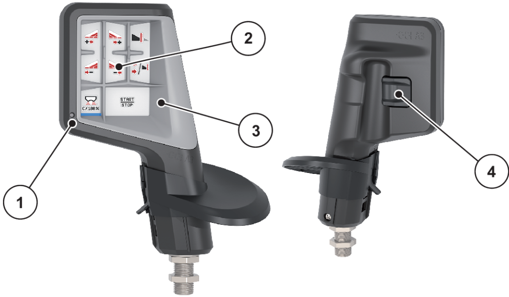
Şek. 39: CCI A3 kumanda çubuğu, ön ve arka taraf
