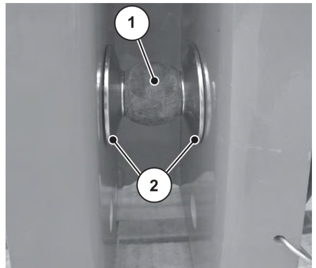
Ábr. 11: A távtartó tárcsák helye a gép összeszerelése során
