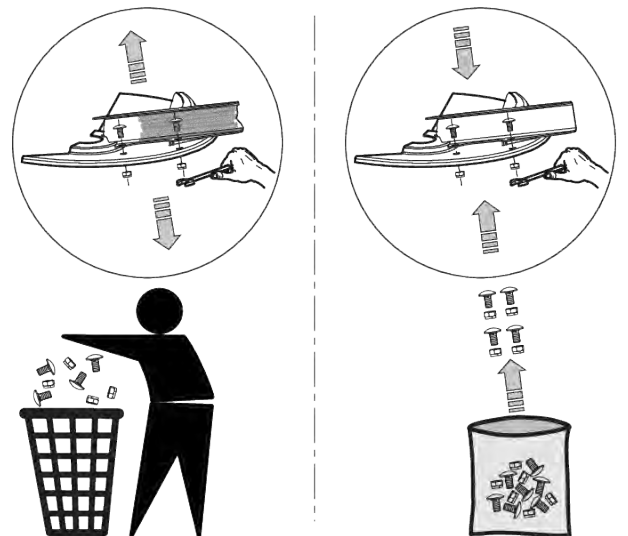
Ábr. 57: Használjon új önzáró anyát
