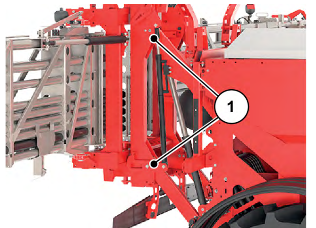
Fig. 98: Lejebolte påbygningsramme
