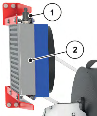
Fig. 69: Temperatursensor på oliekoeleren
