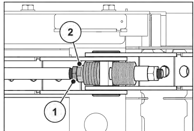
Fig. 60: Ændring af holdespænding på den 2. hydrocylinder
