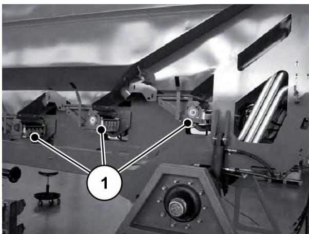
Fig. 80: Hydromotorer i venstre side på doseringen
