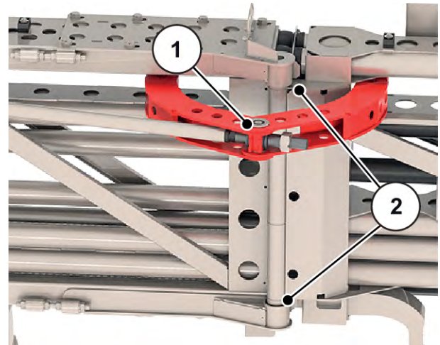
Fig. 94: Bommidterdel
