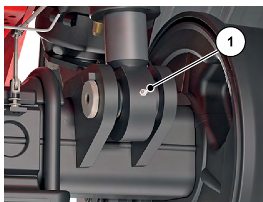
Fig. 100: Ledlejer på hydrocylinder til akselaffjedring
