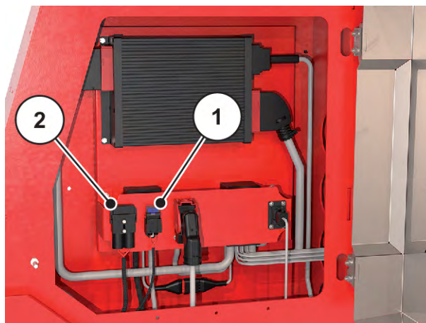
Fig. 65: Sikringer på ISOBUS-kablet
