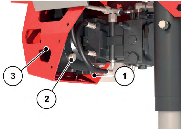
Fig. 78: Aftapning af gearolie
