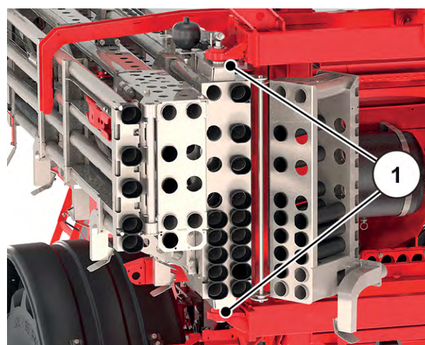
Fig. 91: Ledlejer til bom på pendulramme
