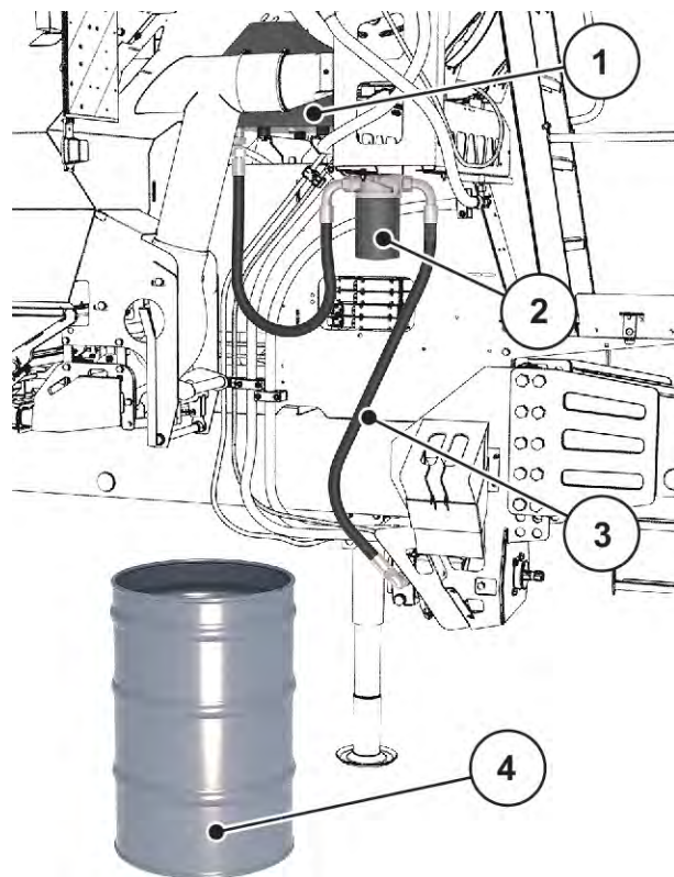
Fig. 76: Oliefilter
