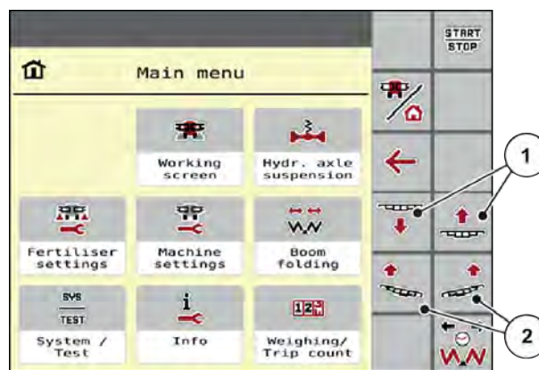
Fig. 45: Funktionstaster til justering af bomhældning/-højde
