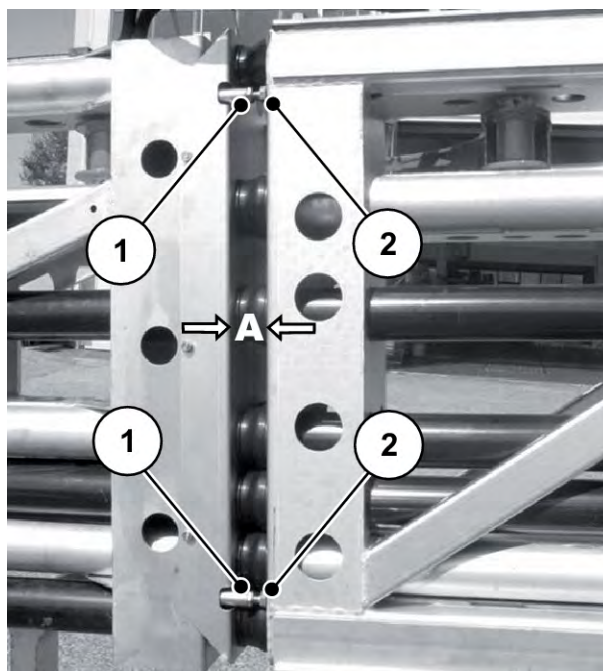
Fig. 57: Vertikal indstilling af udklappede bomsegmenter
