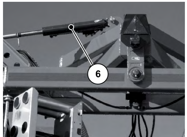
Fig. 73: Hydraulikcylinder skråningshældning
