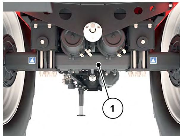
Fig. 87: Bjærgning af maskinen med tov/wire
