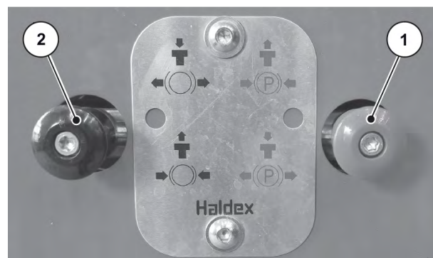
Fig. 28: Trykluft-bremse
