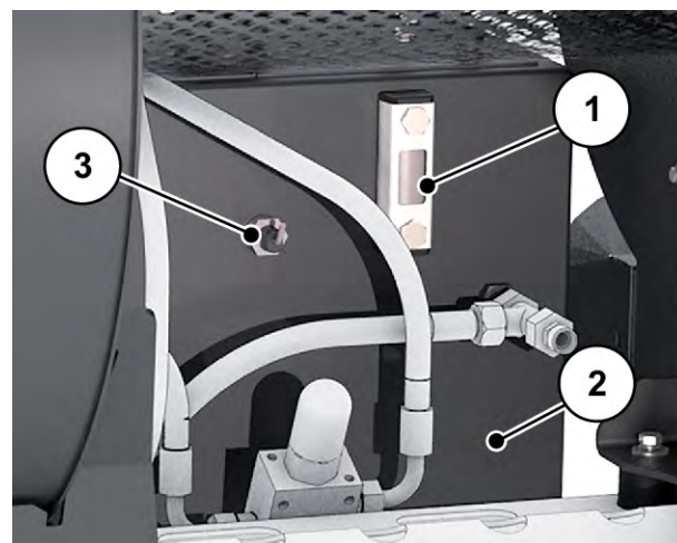
Fig. 77: Påfyldning af olie
