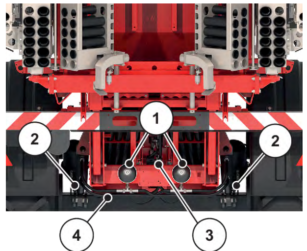
Fig. 84: Contrôler la suspension de l'essieu
