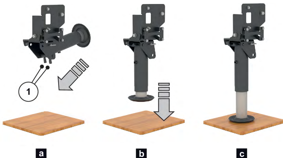
Fig. 56: Dépliage de la béquille
