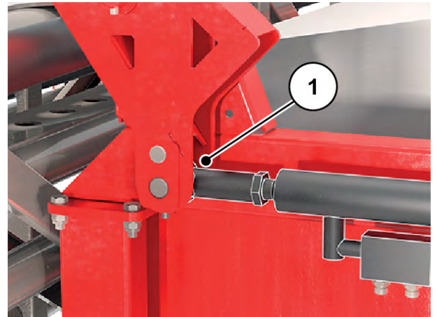
Fig. 92: Vérin hydraulique pour le dispositif de sécurité de la rampe
