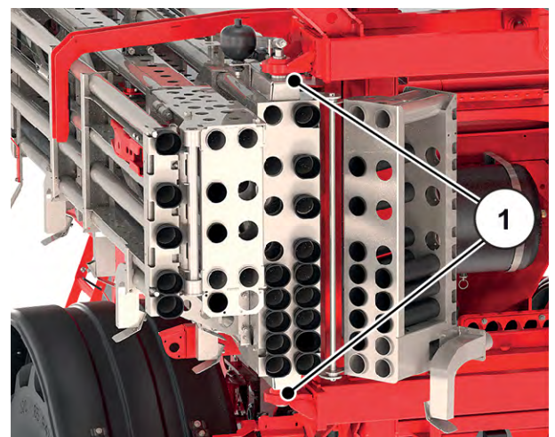
Fig. 91: Support articulé pour rampe sur le châssis pendulaire
