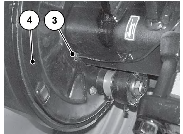
Fig. 68: Moyeu de roue gauche
