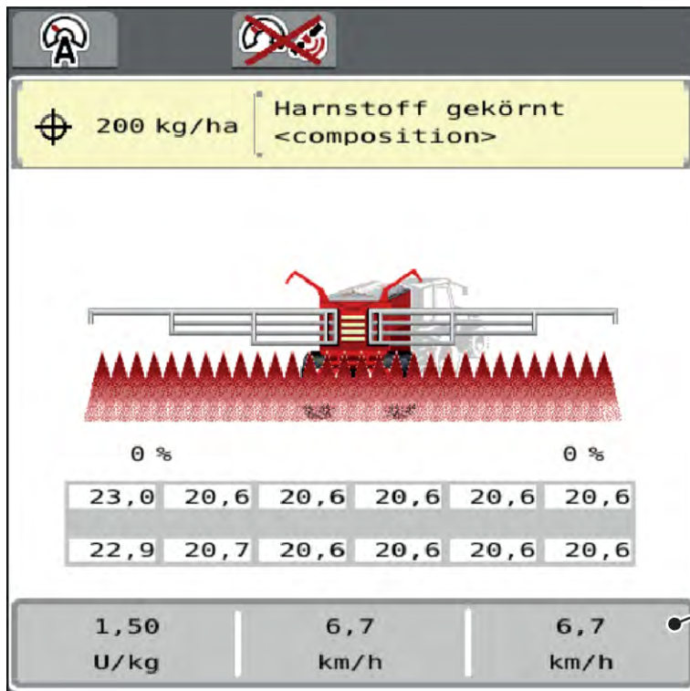
Fig. 67: Écran de travail
