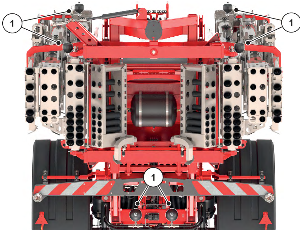
Fig. 70: Accumulateur d'azote
