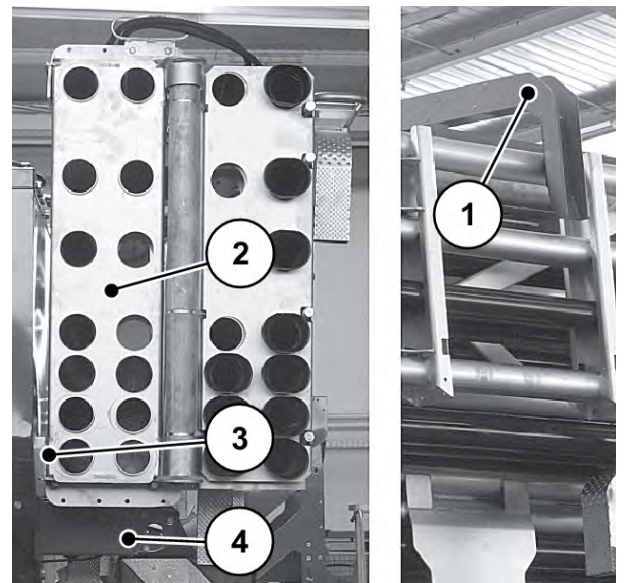
Fig. 61: Contrôle de la rampe pliée
