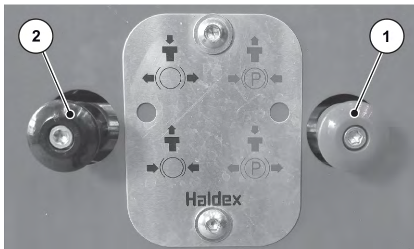
Fig. 53: Serrage du frein de stationnement manuel
