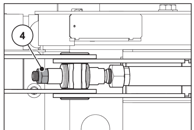
Fig. 63: Partie centrale de la rampe
