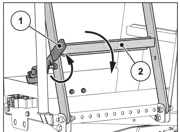
Fig. 31: Dépliage du marchepied
