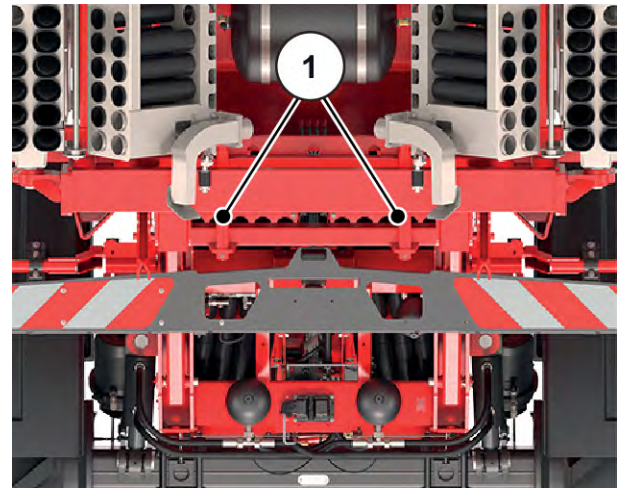
Fig. 90: Surface lisse entre la goupille de centrage et le châssis pendulaire
