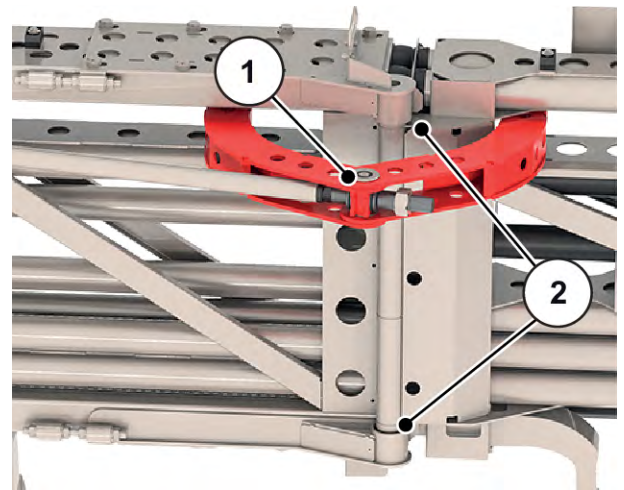
Fig. 94: Partie centrale de la rampe
