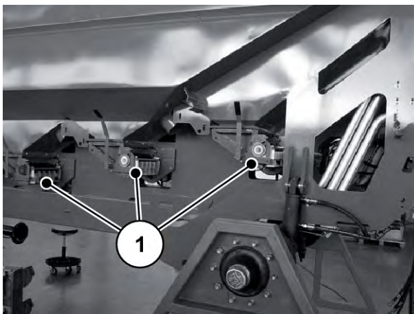
Fig. 80: Moteurs hydrauliques à gauche du dispositif de dosage
