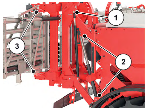
Fig. 97: Support articulé sur le vérin hydraulique destiné au parallélogramme
