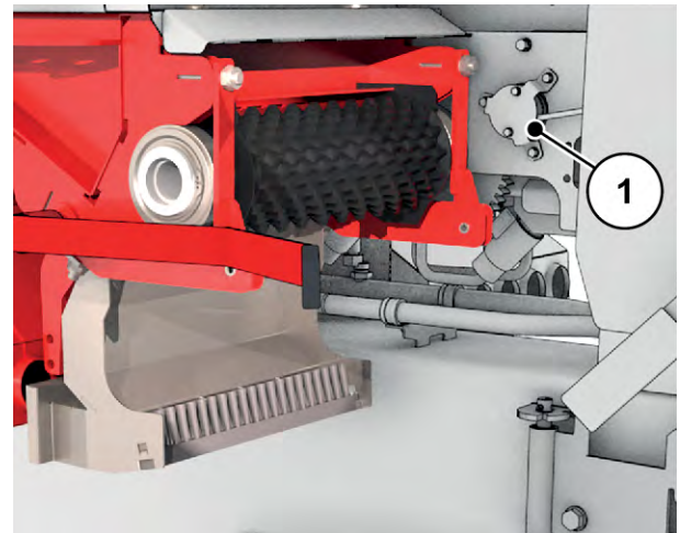
Fig. 66: Dosage à droite
