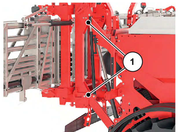
Fig. 98: Boulons d'appui sur le cadre additionnel
