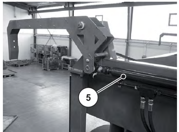
Fig. 72: Vérin hydraulique pour le dispositif de verrouillage de transport
