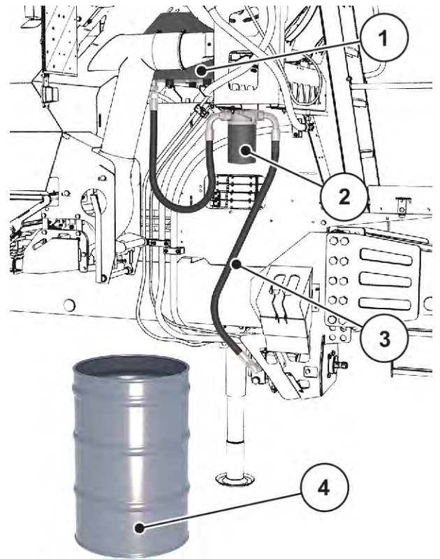
Fig. 76: Filtre à huile
