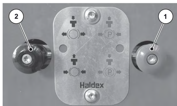
Fig. 28: Frein pneumatique
