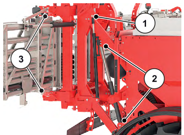
Fig. 88: Support articulé sur le vérin hydraulique destiné au verrouillage du châssis pendulaire
