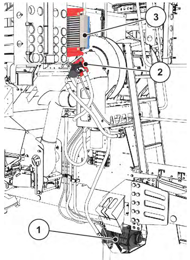
Fig. 79: Contrôle de la pompe à piston axial, du moteur à piston axial et du refroidisseur d'huile
