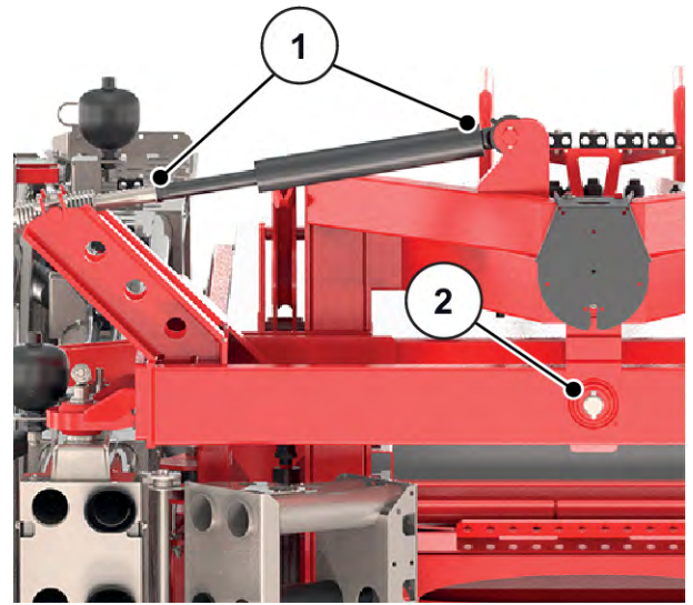
Fig. 89: Point de lubrification du châssis pendulaire
