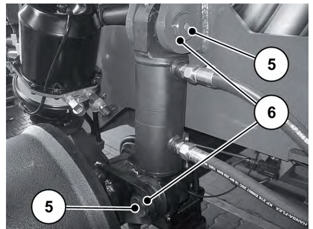
Fig. 85: Contrôle des fixations du cylindre de suspension
