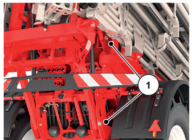
Fig. 99: Boulons d'appui parallélogramme
