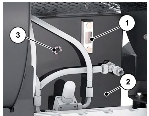
Fig. 74: Position du réservoir d'huile de l'entraînement Vario
