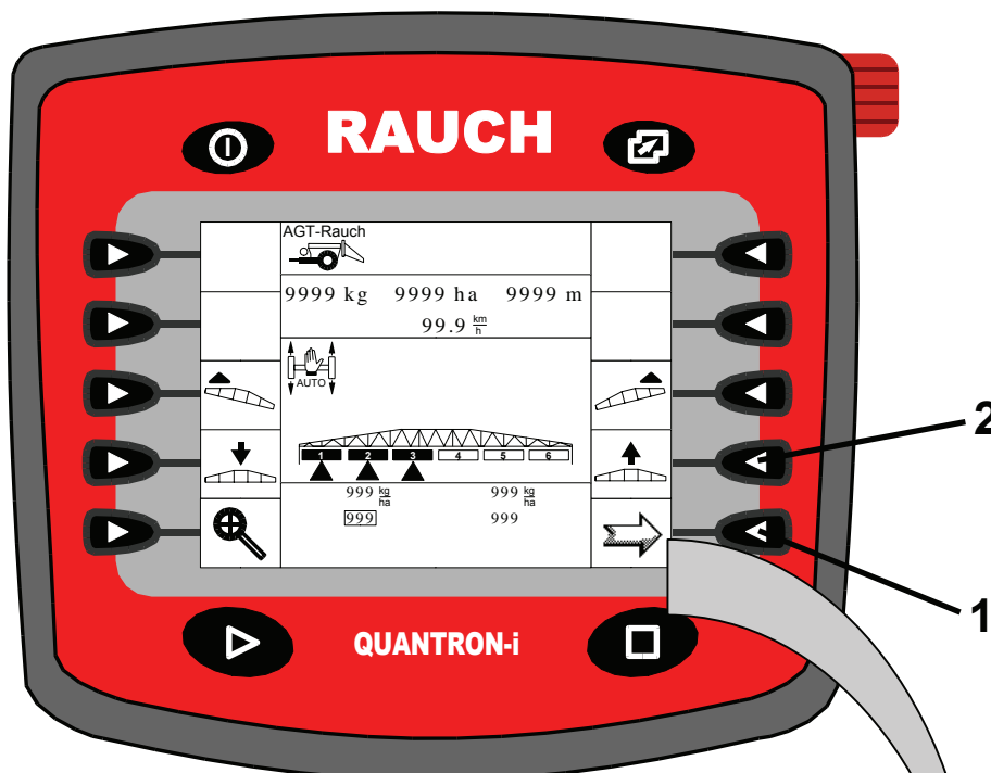
Betriebsbild 2
