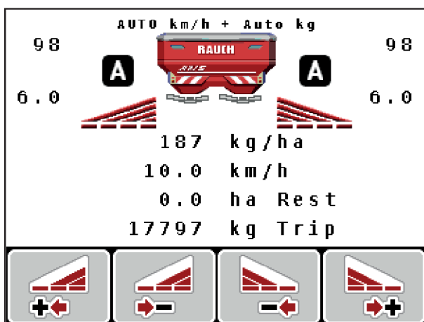
Рис. 56: Відображення на робочому екрані: Режим внесення добрива з GPS Control
