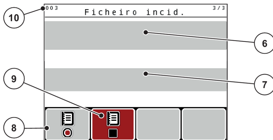
Ilust. 38: Indicação do ficheiro de incidências atual
