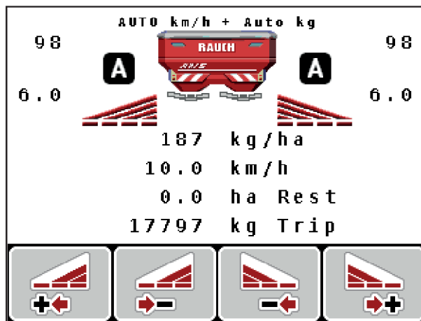
Ilust. 56: Indicação no ecrã de trabalho: Modo de dispersão com GPS Control
