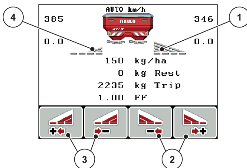
Ilust. 51: Imagem de funcionamento do modo de dispersão com larguras parciais
