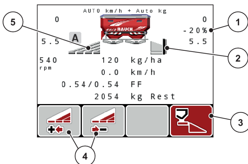
Ilust. 53: Imagem de funcionamento de uma largura parcial esquerda, lado da dispersão limite direito
