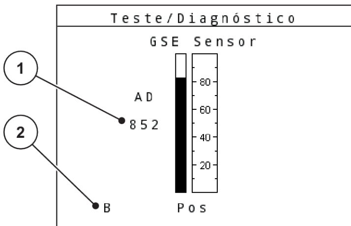
Ilust. 45: Teste/Diagnóstico; Exemplo: Linbus
