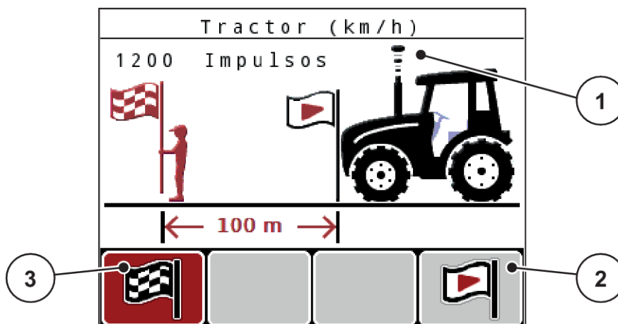
Ilust. 34: Imagem de funcionamento de marcha de calibragem e sinal de velocidade
