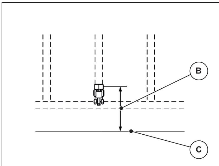
Sl. 57: Razmak isključivanja (prema granici polja)
