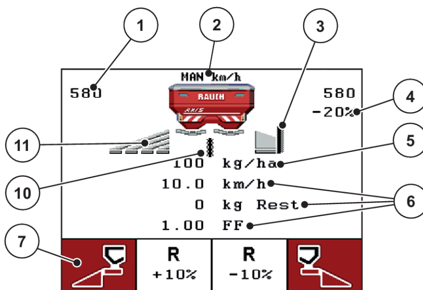
Sl. 3: Displej upravljačke jedinice – primer radnog ekrana za AXIS-M
