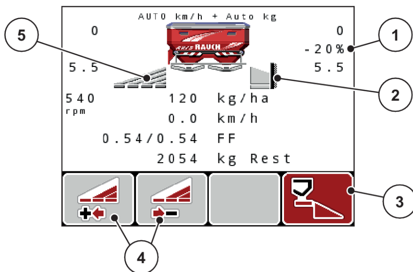
Sl. 51: Radni ekran za jednu sekciju levo, strana graničnog rasipanja desno
