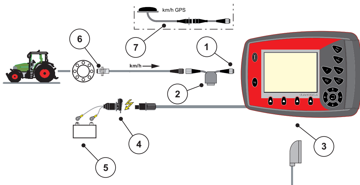
Obrázok 3.4: Schematický prehľad pripojenia QUANTRON-A (snímač koleša)
