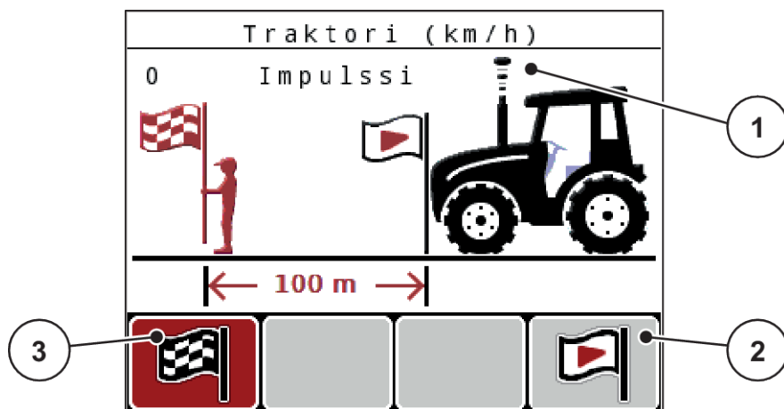
Kuva 33: Näyttökuva Kalibrointiajon nopeussignaali
