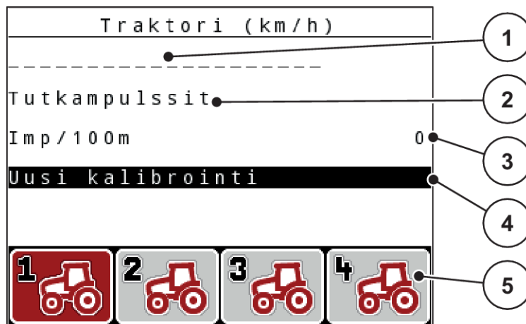
Kuva 31: Valikko Traktori (km/h)
