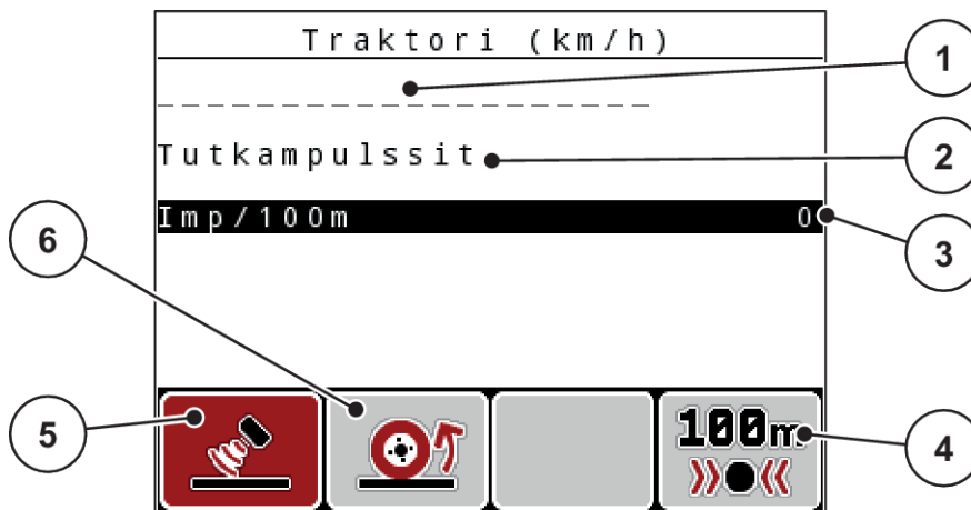
Kuva 32: Kalibroitivalikko Traktori (km/h)
