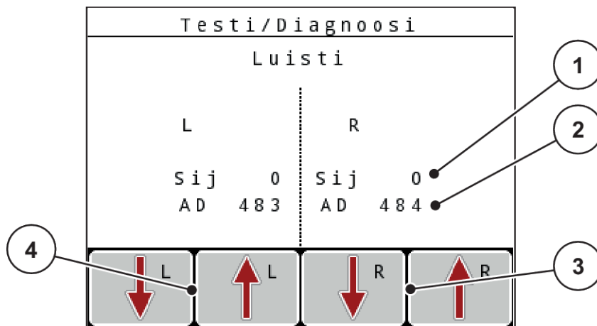
Kuva 42: Testi/diagnoosi, esimerkki: annostusluisti
