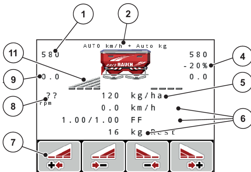
Kuva 4: Ohjausyksikön näyttö – esimerkkinä näyttökuvaa AXIS-M EMC
