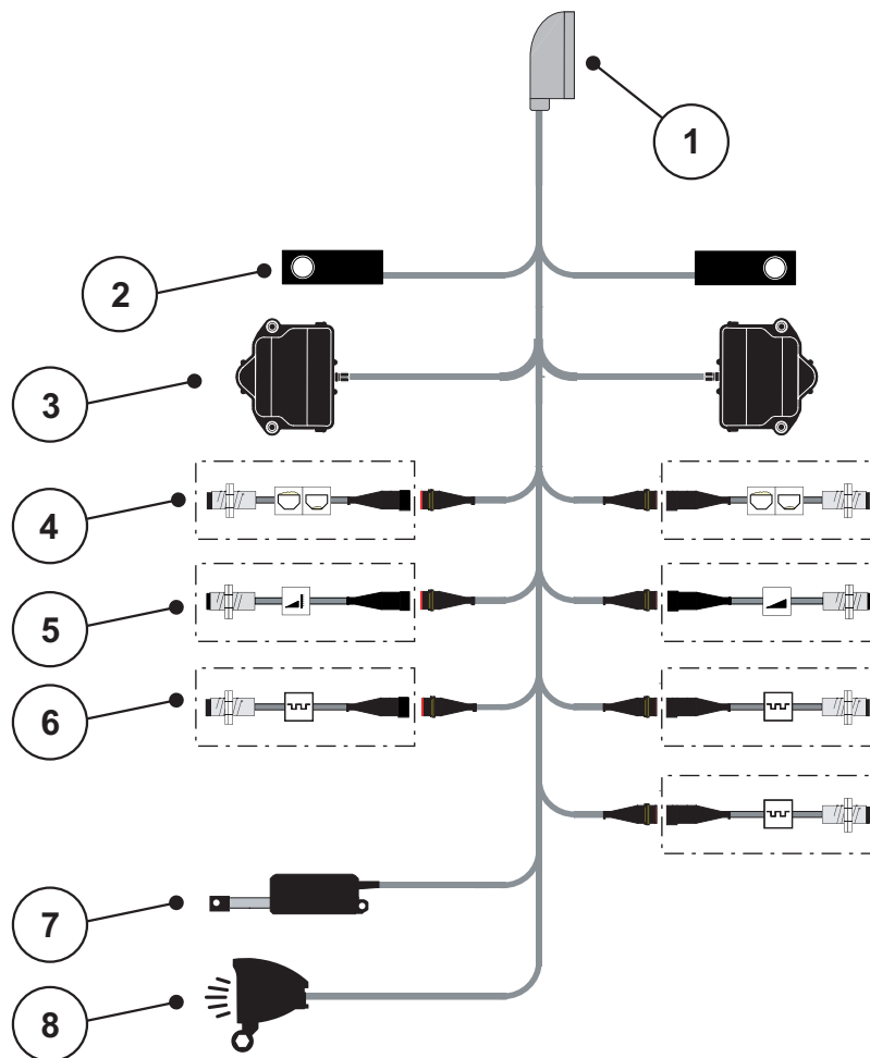
Kuva 3.8: Liitäntäkaavio QUANTRON-A
