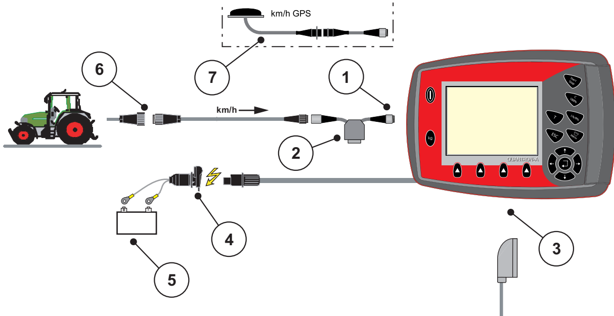
Kuva 3.3: Liitännäkaavio QUANTRON-A (vakio)
