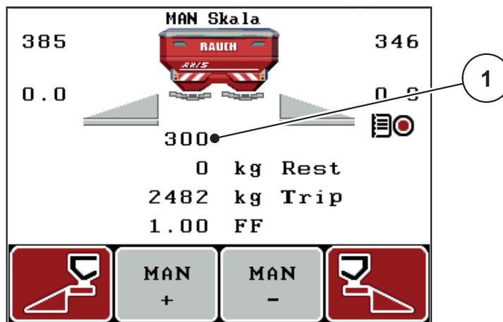
Kuva 5.5: Käyttökuvassa MAN asteikko
