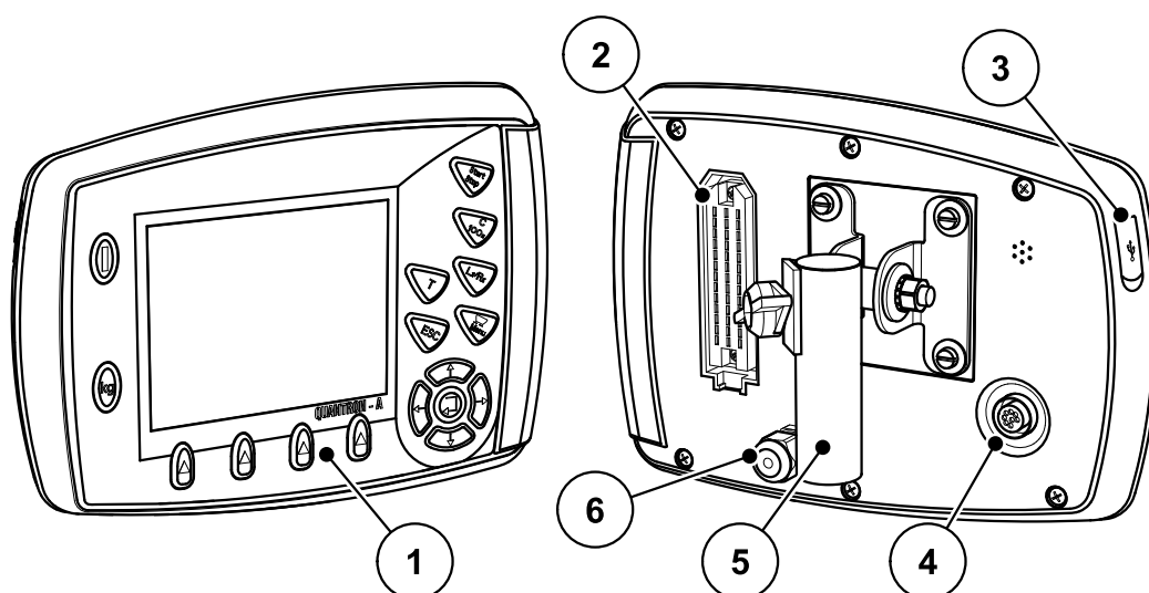
Kuva 2.1: Käyttöyksikkö QUANTRON-A
