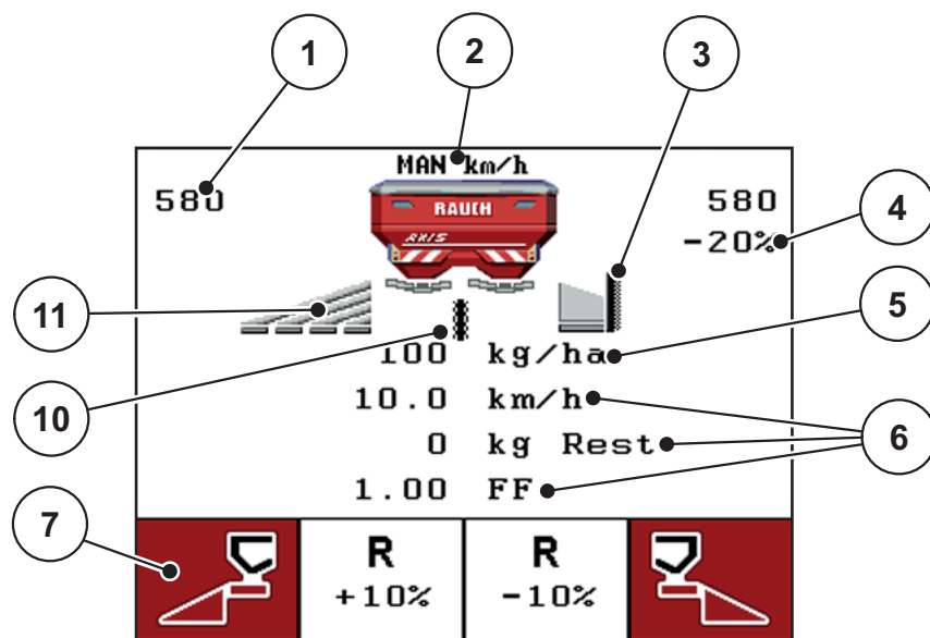
Kuva 2.3: Käyttöyksikön näyttö (esimerkki käyttökuvasta AXIS-M)
