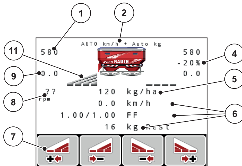
Joonis 2.4: Juhtseadme displei (AXIS-M EMC käitusvaate näide)
