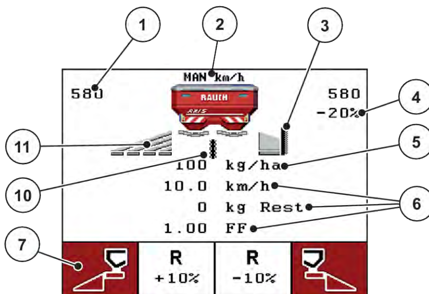
Fig. 3: Display-ul unității de operare - exemplu imaginea de operare AXIS-M
