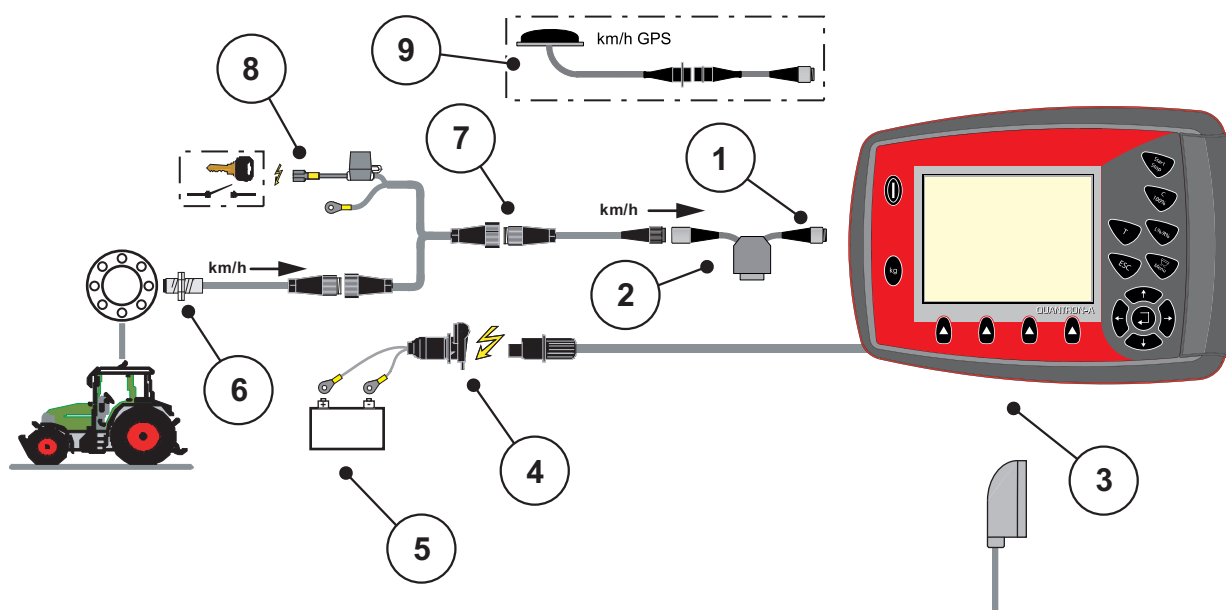
Bild 3.5: Schematisk anslutningsöversikt för QUANTRON-A (Strömförsörjning via tändningslås)
