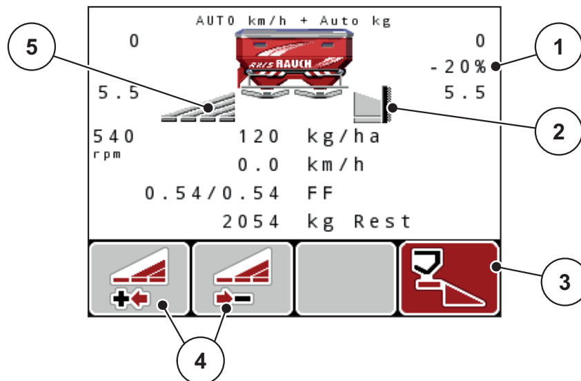
Bild 5.2: Driftsbild för en delbredd vänster, gränsspridningssida höger
