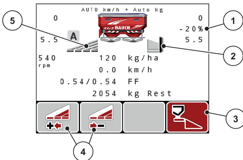
Fig. 53: Driftsbilde for en delbredde venstre, grensespredeside høyre
