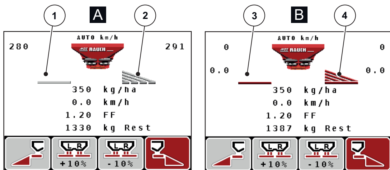
Фиг. 2.7: Индикация за състоянието на дозирация шибър MDS
