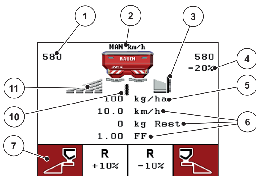
Фиг. 2.3: Дисплей на блока за управление (пример работен екран AXIS-M)
