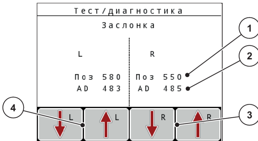
Рис. 43: Тест/диагностика; пример: заслонка дозатора
