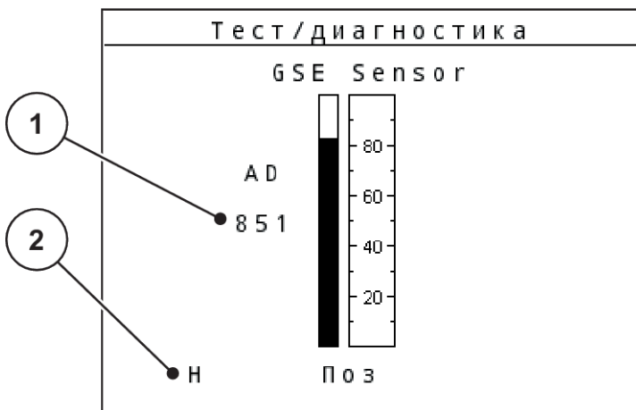
Рис. 45: Тест/диагностика; пример: Linbus
