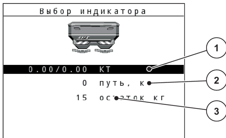
Рис. 42: Поля индикации
