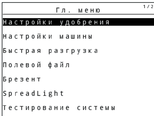
Рис. 21: Гл. меню
