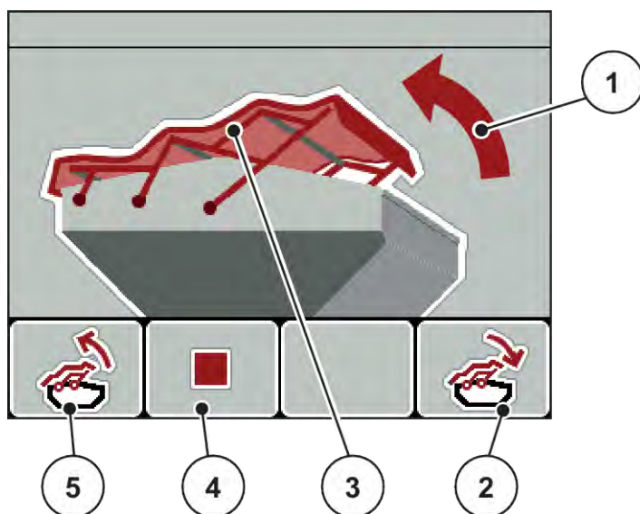
Рис. 47: Меню «Брезент»
