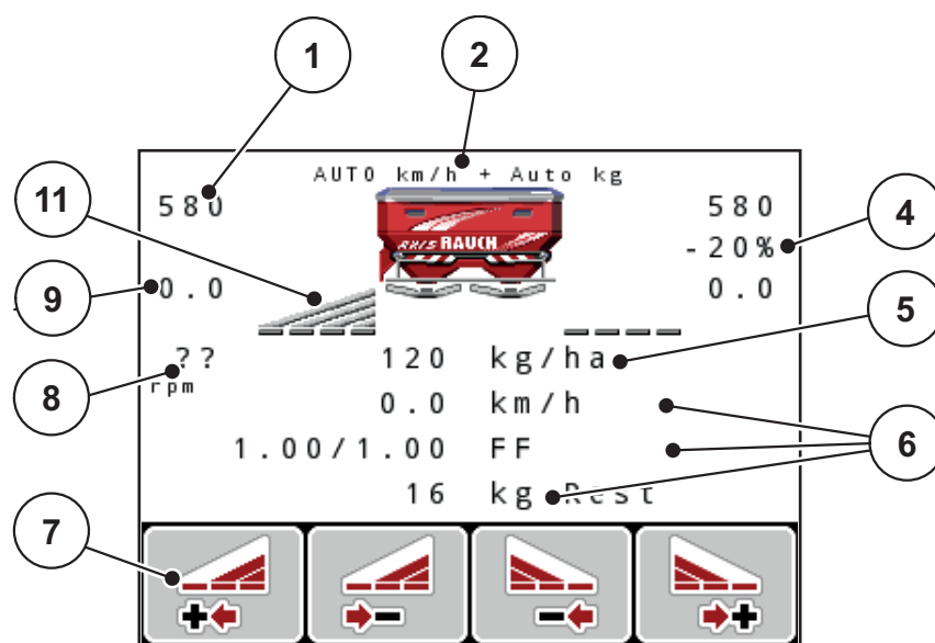
Рисунок 2.4: Дисплей блока управления (пример рабочего экрана AXIS-M EMC)
