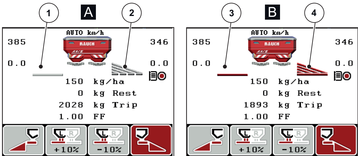
Рисүнок 2.6: Индикация состояний заслонки дозатора AXIS
