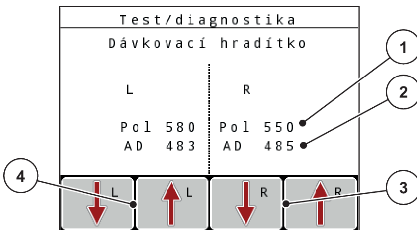
Obr. 43: Test/diagnostika; příklad: Dávkovací hradítko
