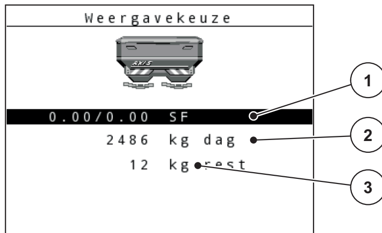
Afb. 4.26: Menu Weergavekeuze
