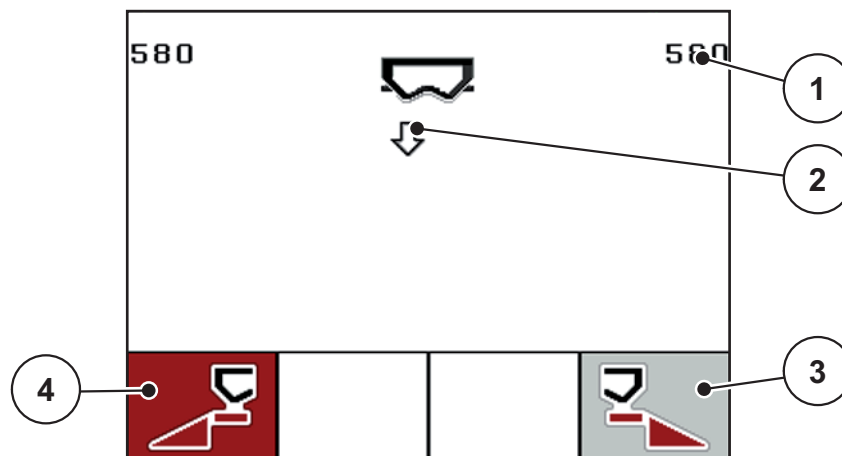
Afb. 4.20: Menu Snellossen
