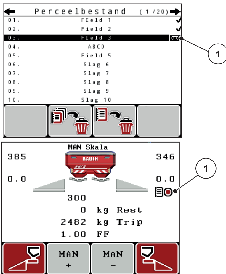
Afb. 4.23: Weergave opnamesymbool
