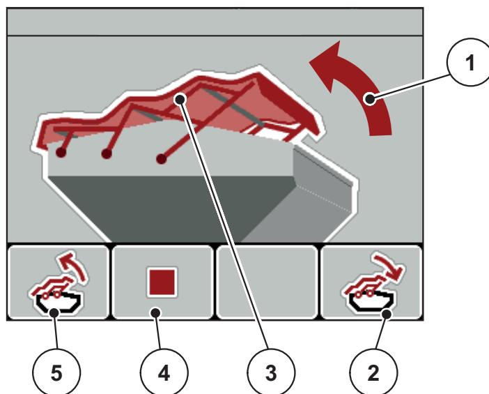
Afb. 4.31: Menu Afdekzeil
