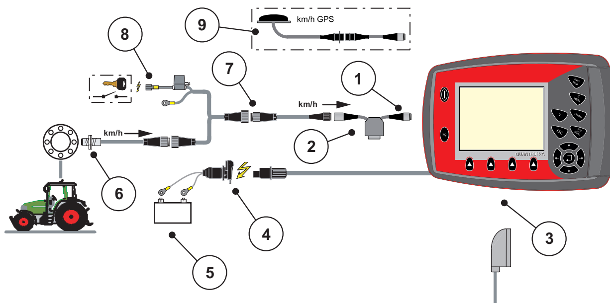
Billede 3.5: Skematisk tilslutningsoversigt QUANTRON-A (Strømforsyning via tændingslås)
