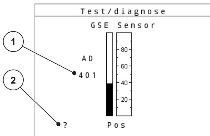
Billede 4.29: Test/diagnose; eksempel: Linbus
