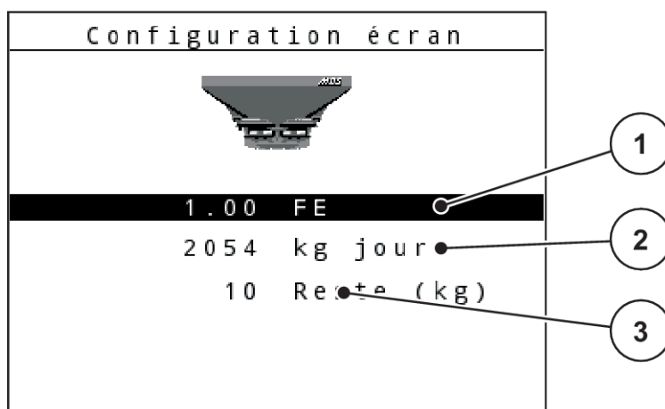
Fig. 42: Champs d'affichage
