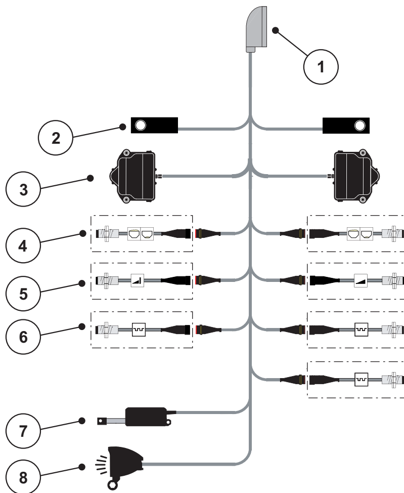
Bild 3.8: Schematische Anschlussübersicht QUANTRON-A
