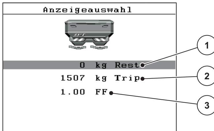
Bild 4.26: Menü Anzeigerauswahl
