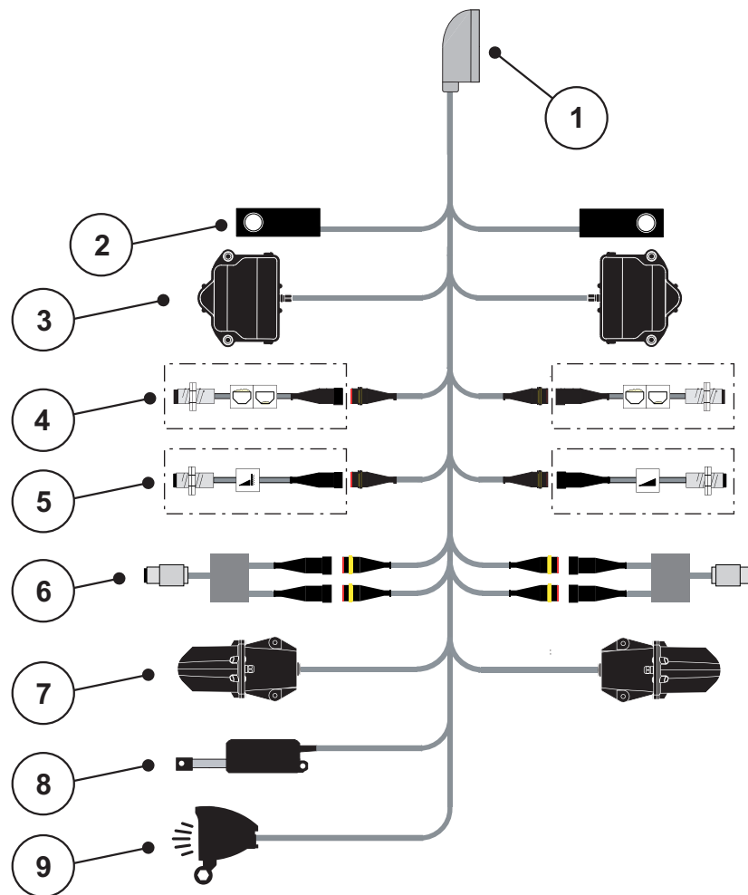
Bild 3.9: Schematische Anschlussübersicht QUANTRON-A
