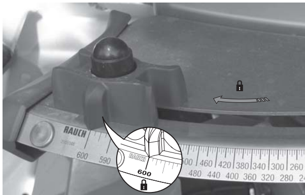
Bild 3.10: Vorbereitung des AXIS Dosierschiebers (Beispiel)
