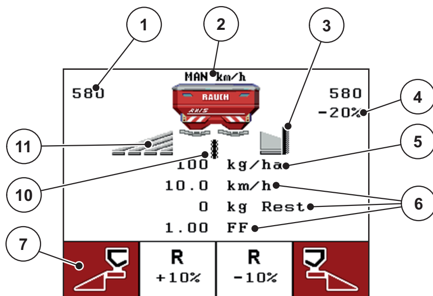
Bild 2.3: Display der Bedieneinheit (Beispiel Betriebsbild AXIS-M)
