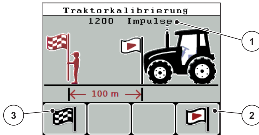
Bild 4.18: Betriebsbild Kalibrierfahrt Geschwindigkeitssignal
