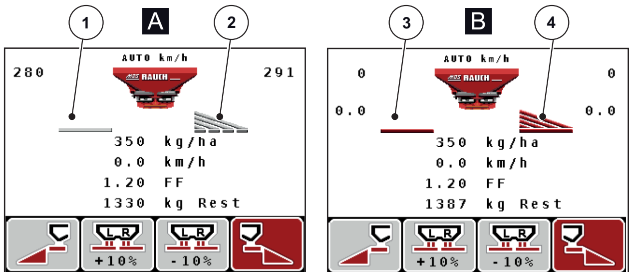
Bild 2.7: Anzeige der Dosierschieberzustände MDS
