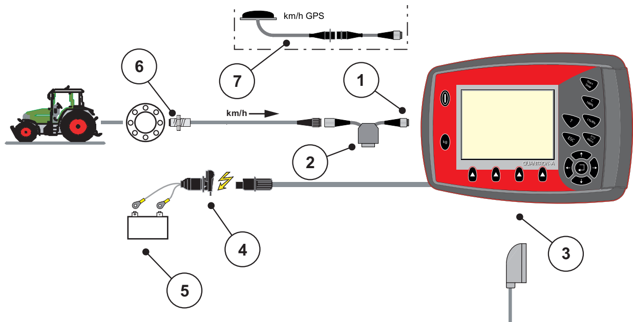
Bild 3.4: Schematische Anschlussübersicht QUANTRON-A (Radsensor)
