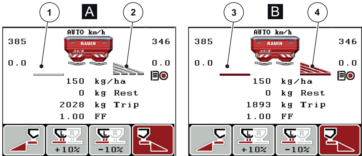
Bild 2.6: Anzeige der Dosierschieberzustände AXIS
