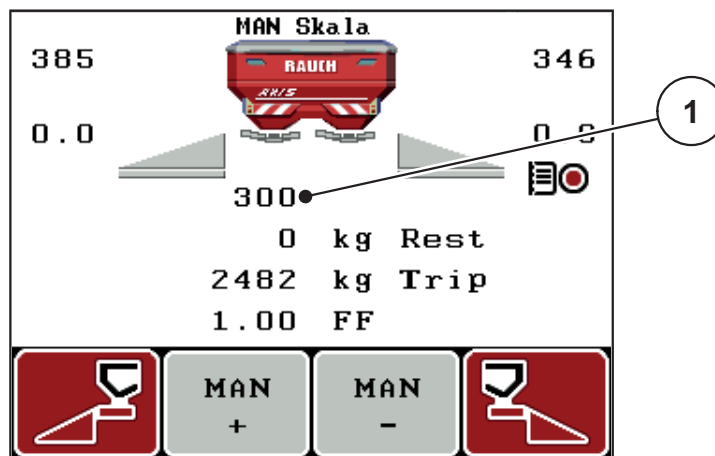
Bild 4.19: Betriebsbild MAN Skala
