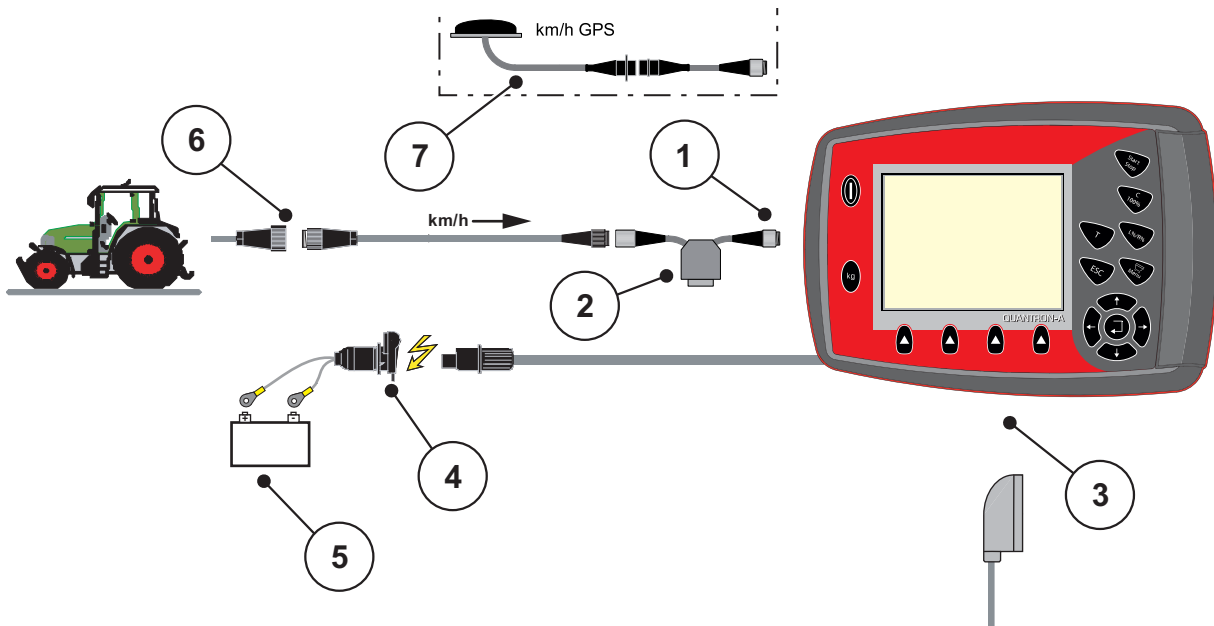
Bild 3.3: Schematische Anschlussübersicht QUANTRON-A (Standard)
