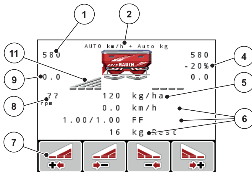
Bild 2.4: Display der Bedieneinheit (Beispiel Betriebsbild AXIS-M EMC)
