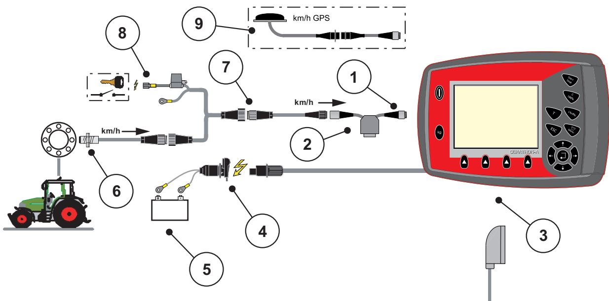
Bild 3.5: Schematische Anschlussübersicht QUANTRON-A (Stromversorgung über Zündschloss)
