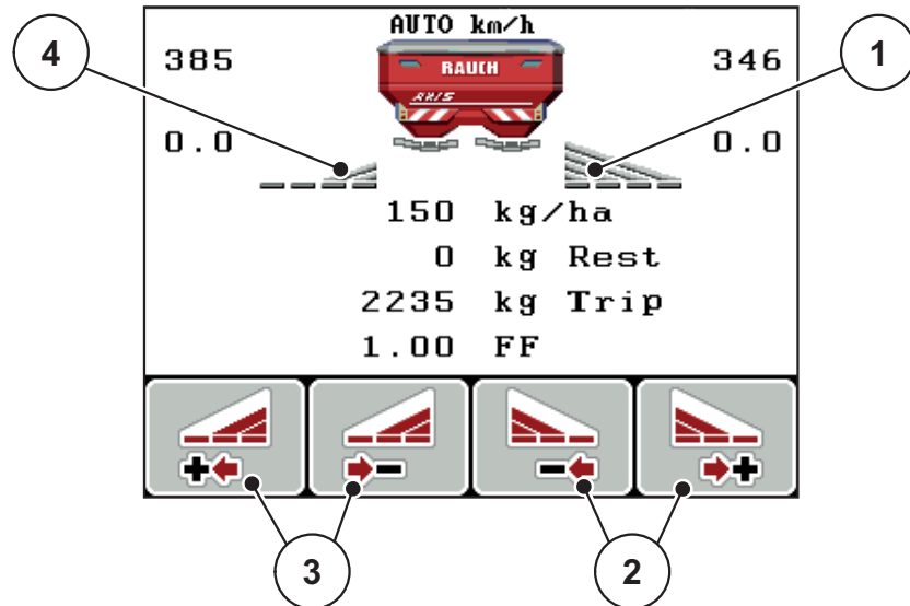
Bild 5.1: Betriebsbild Streubetrieb mit Teilbreiten
