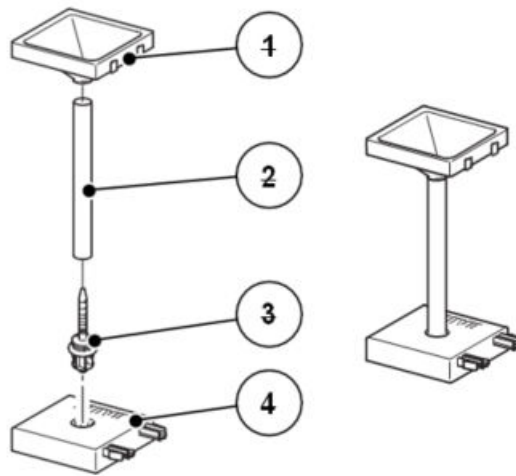
Fig. 1: Assemblage des éprouvettes
