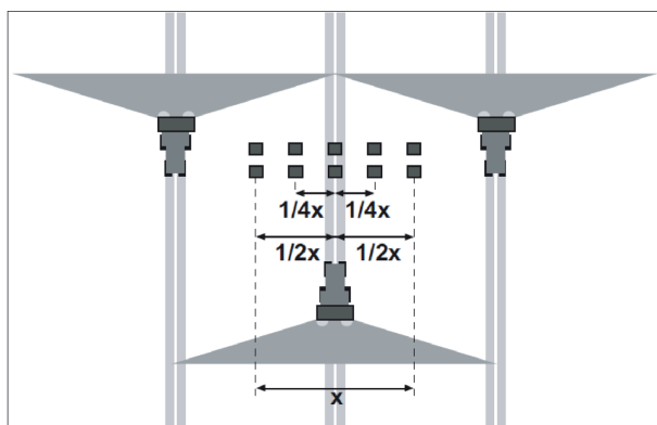
Fig. 7: Installation pour 3 passages
