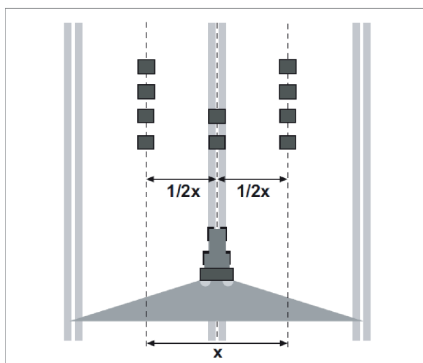
Fig. 5: Installation pour un passage
