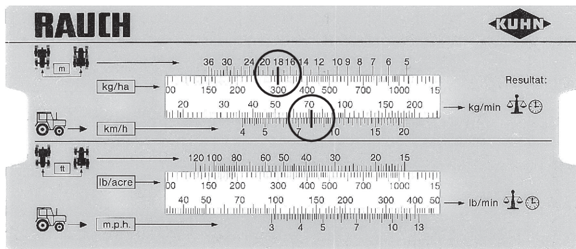
Obr. 32: Stupnice na stanovení požadovaného výstupního množství za minutu
