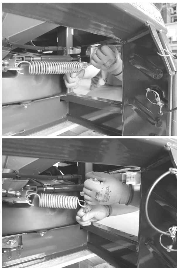
Obr. 69: Vyvěšení pružiny
