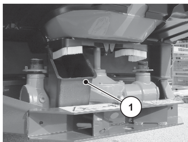
Obr. 36: Zavěšení žlabu na provedení zkoušky dávky
