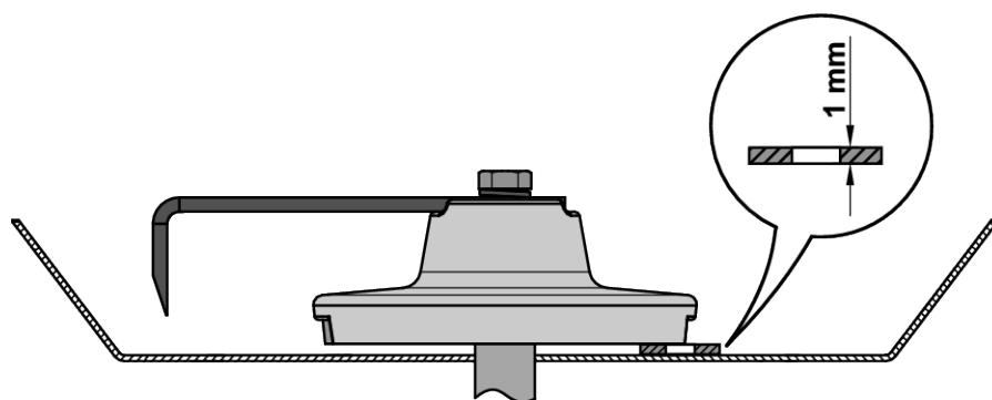
Obr. 78: Nastavení míchadla
