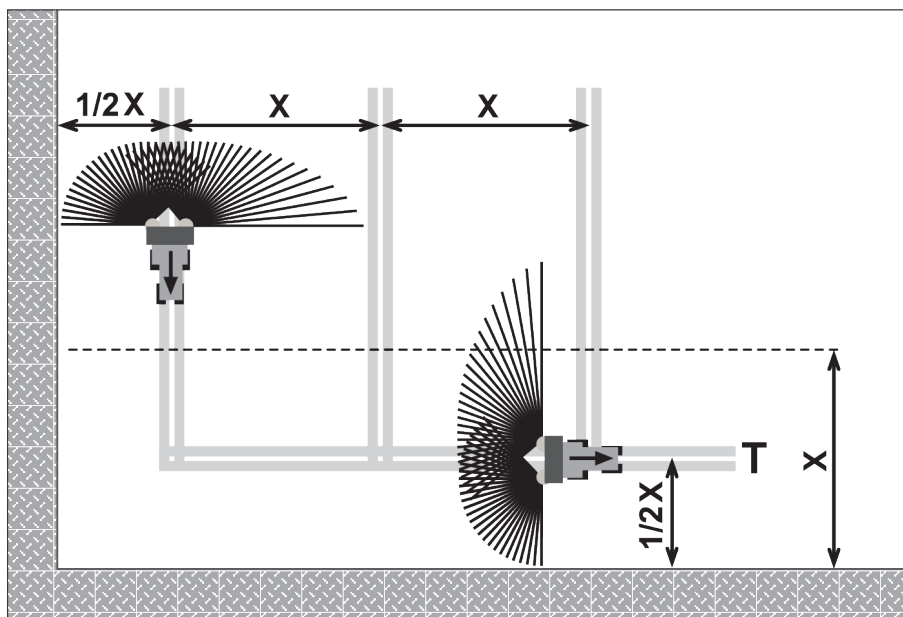
Obr. 57: Hraniční rozmetání
