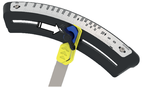
Obr. 73: Posunutí dorazu
