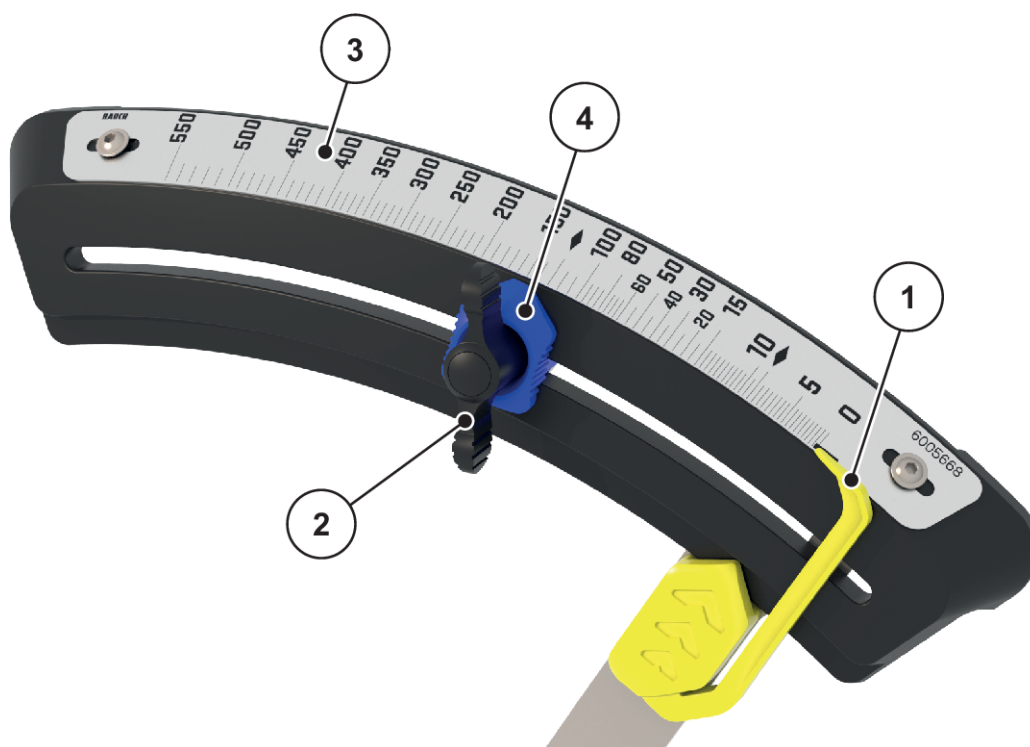
Obr. 39: Stupnice nastavení rozmetávaného množství (směr jízdy vpravo, varianty K/D/C)
