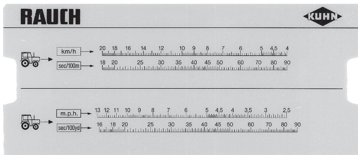
Obr. 31: Stupnice na stanovení přesné rychlosti jízdy
