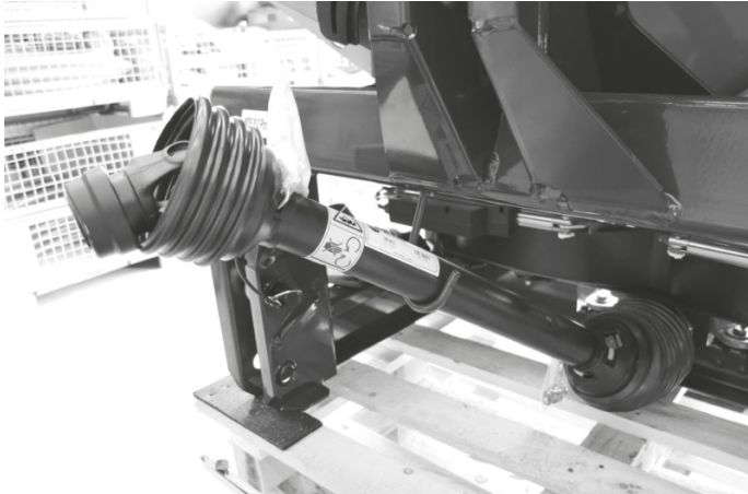
Obr. 62: Uložení kloubového hřídele, uložení kabelů a hydraulických hadic
