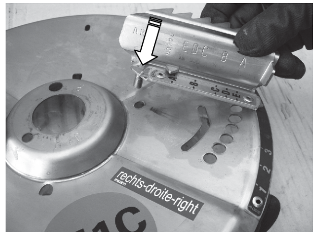
Obr. 90: Montáž hlavní lopatky
