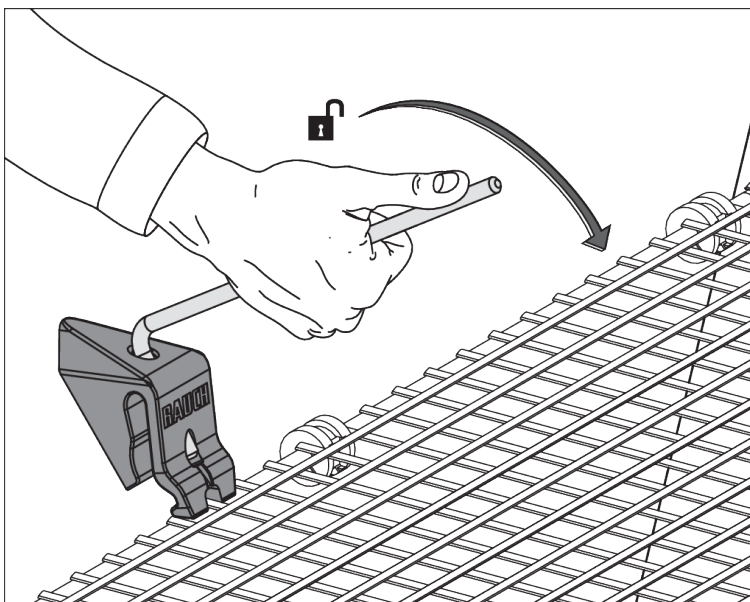
Obr. 66: Otevřete blokování ochranné mříže.
