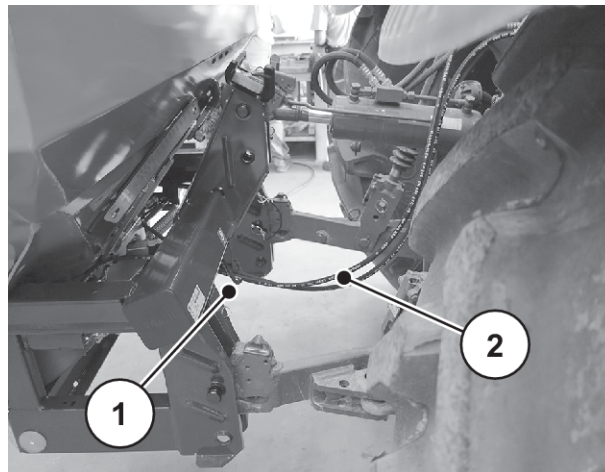
Obr. 23: Vedení hydraulických hadic
