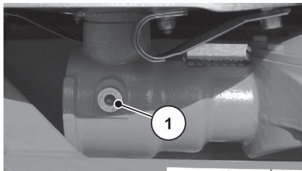
Obr. 95: Místa plnění a vypouštění pro převodový olej
