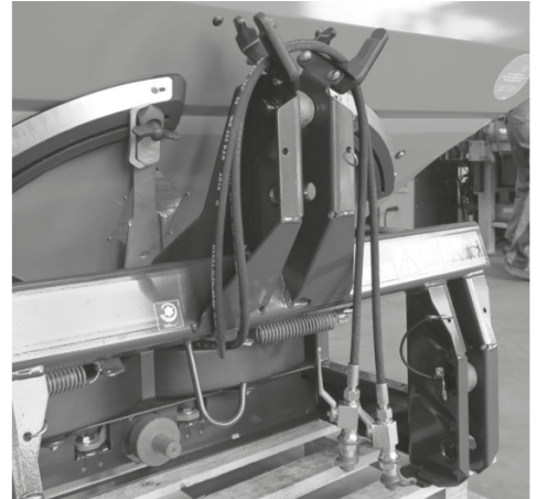
Obr. 62: Uložení kloubového hřídele, uložení kabelů a hydraulických hadic
