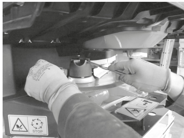
Obr. 76: Povolení uzavřené matice
