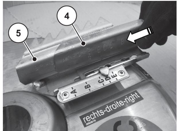
Obr. 83: Nová prodlužovací lopatka
