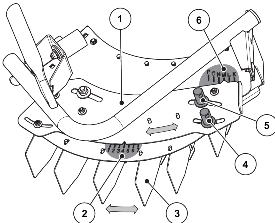
Obr. 55: TELIMAT Nastavení zařízení
