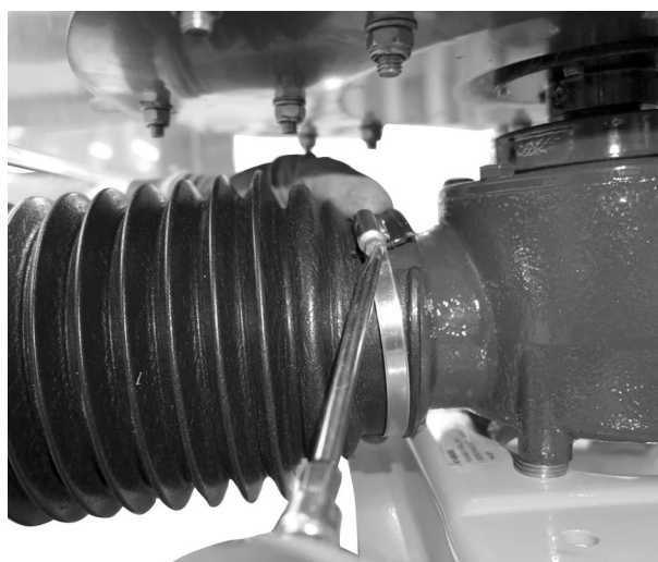
Obr. 14: Montáž krytu kloubového hřídele
