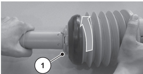
Obr. 17: Povolení krytu kloubového hřídele
