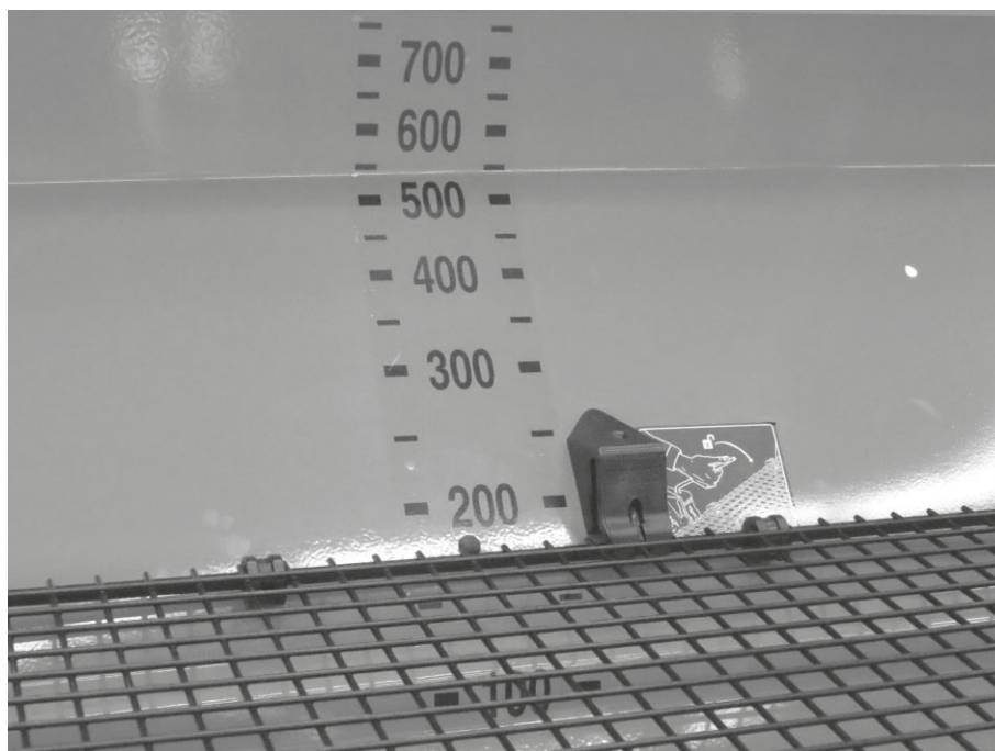
Obr. 30: Stupnice hladiny náplně (údaje v litrech)
