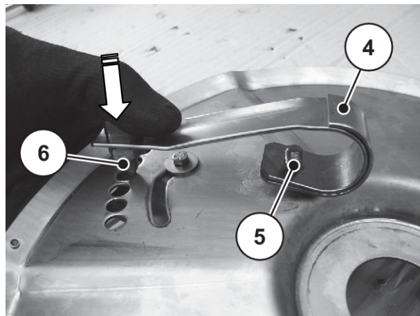
Obr. 93: Plochá pružina rozmetacího disku
