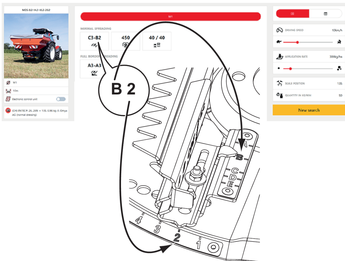
Obr. 41: Nastavení rozmetací lopatky; poloha B2; A až E: Nastavení délky 1 až 6: Nastavení úhlu
