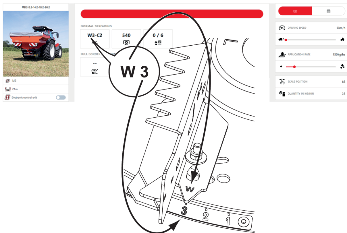
Obr. 42: Nastavení rozmetací lopatky, rozmetací disk M2, poloha W3; W: pevné nastavení délky 1 až 6: nastavení úhlu
