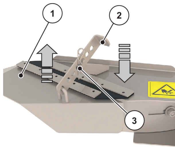
Obr. 61: Změna nastavení na řádkovém rozmetacím zařízení
