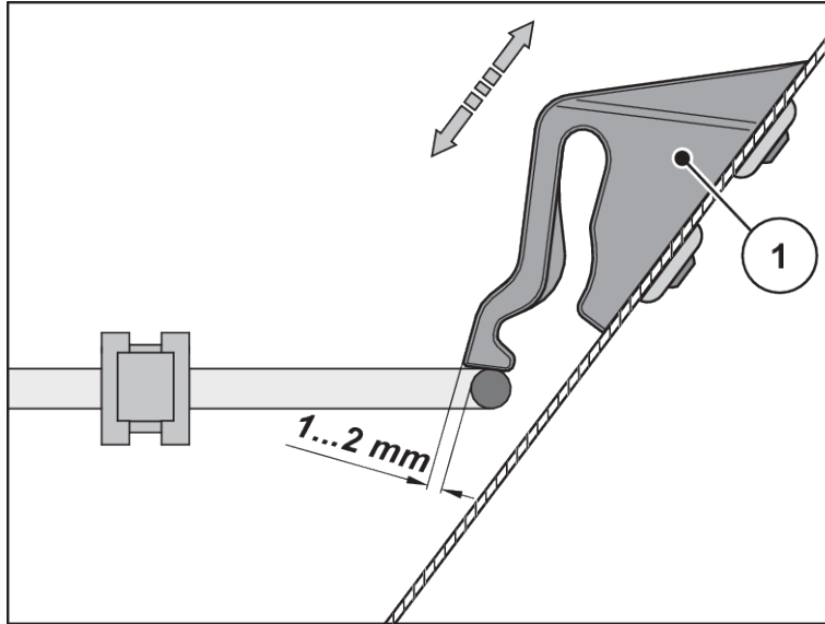
Obr. 67: Kontrolní rozměr pro funkční kontrolu blokování ochranné mříže
