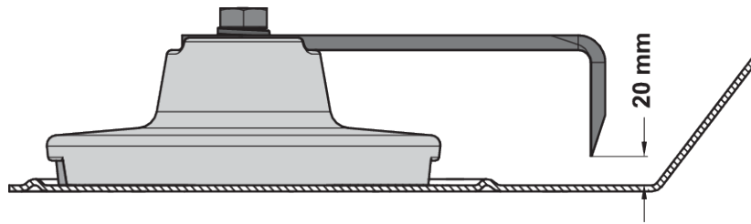
Obr. 75: Rozsah opotřebení míchacího palce
