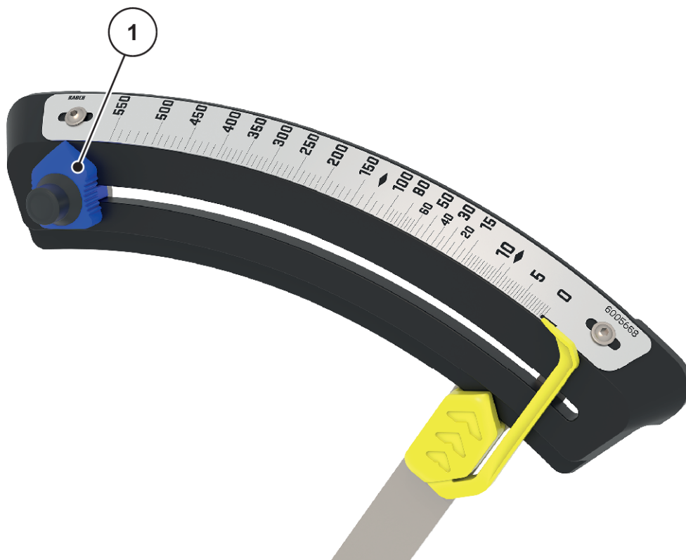
Obr. 40: Stupnice nastavení rozmetávaného množství (směr jízdy vpravo, varianta Q)
