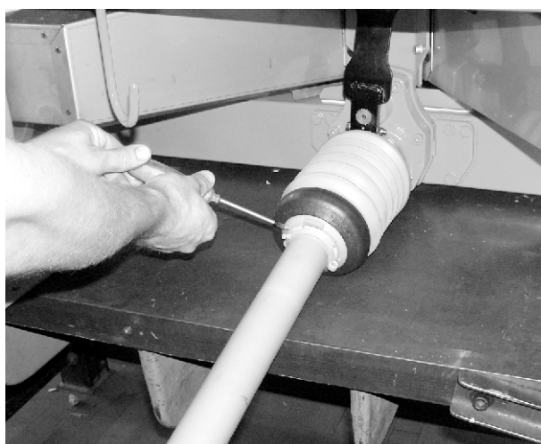
Obr. 21: Zajištění krytu kloubového hřídele
