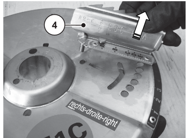
Obr. 89: Sejmутí rozmetací lopatky
