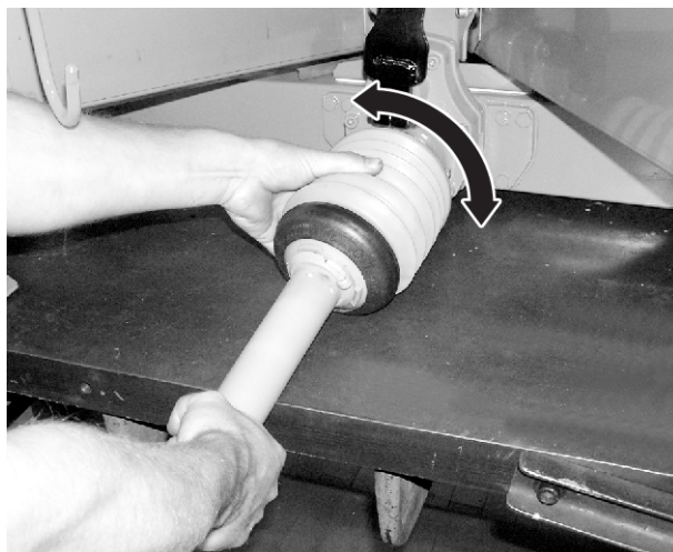
Obr. 20: Nasazení krytu kloubového hřídele
