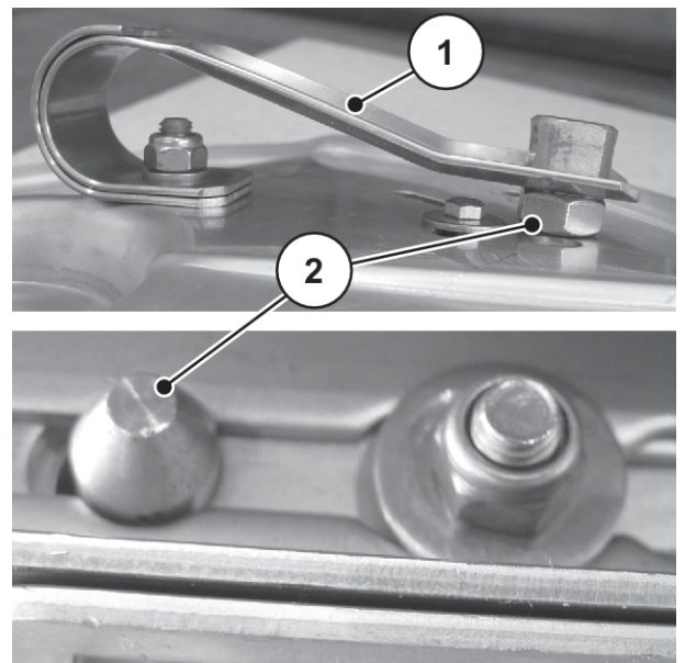
Obr. 77: Aretační čep je správně aretován
