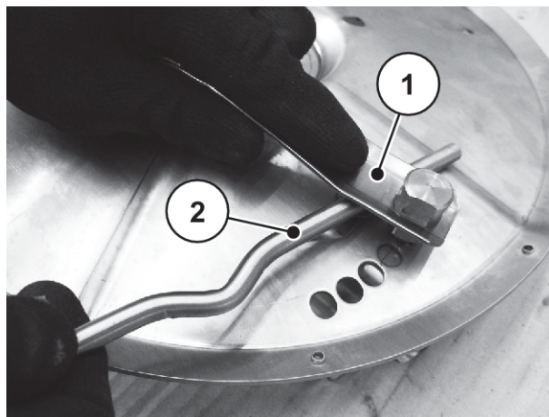
Obr. 87: Odstranění ploché pružiny
