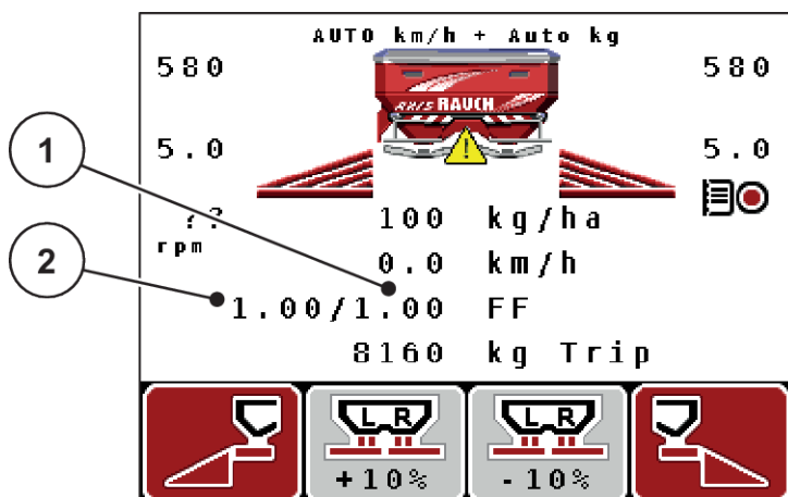
Pav. 26: Kairės ir dešinės pusės byrėjimo koeficiento reguliavimas atskirai (aktyvinta funkcija M EMC)
