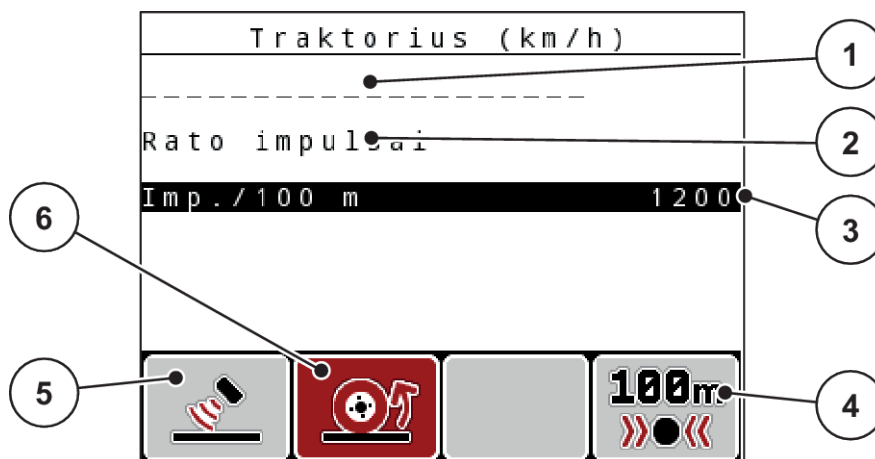
Pav. 32: Kalibravimo meniu Traktorius (km/h)
