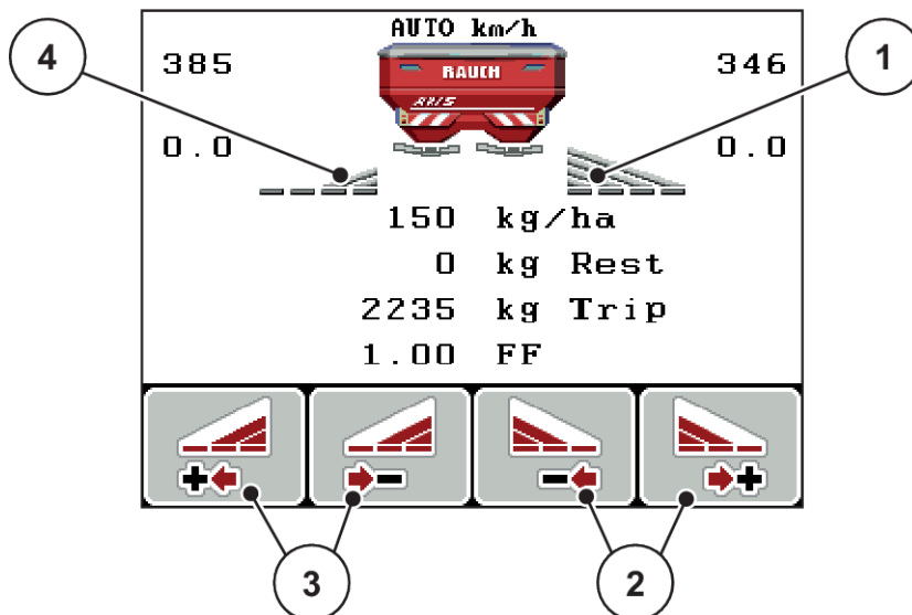
Pav. 50: Barstymo režimo su sekcijomis darbinis langas
