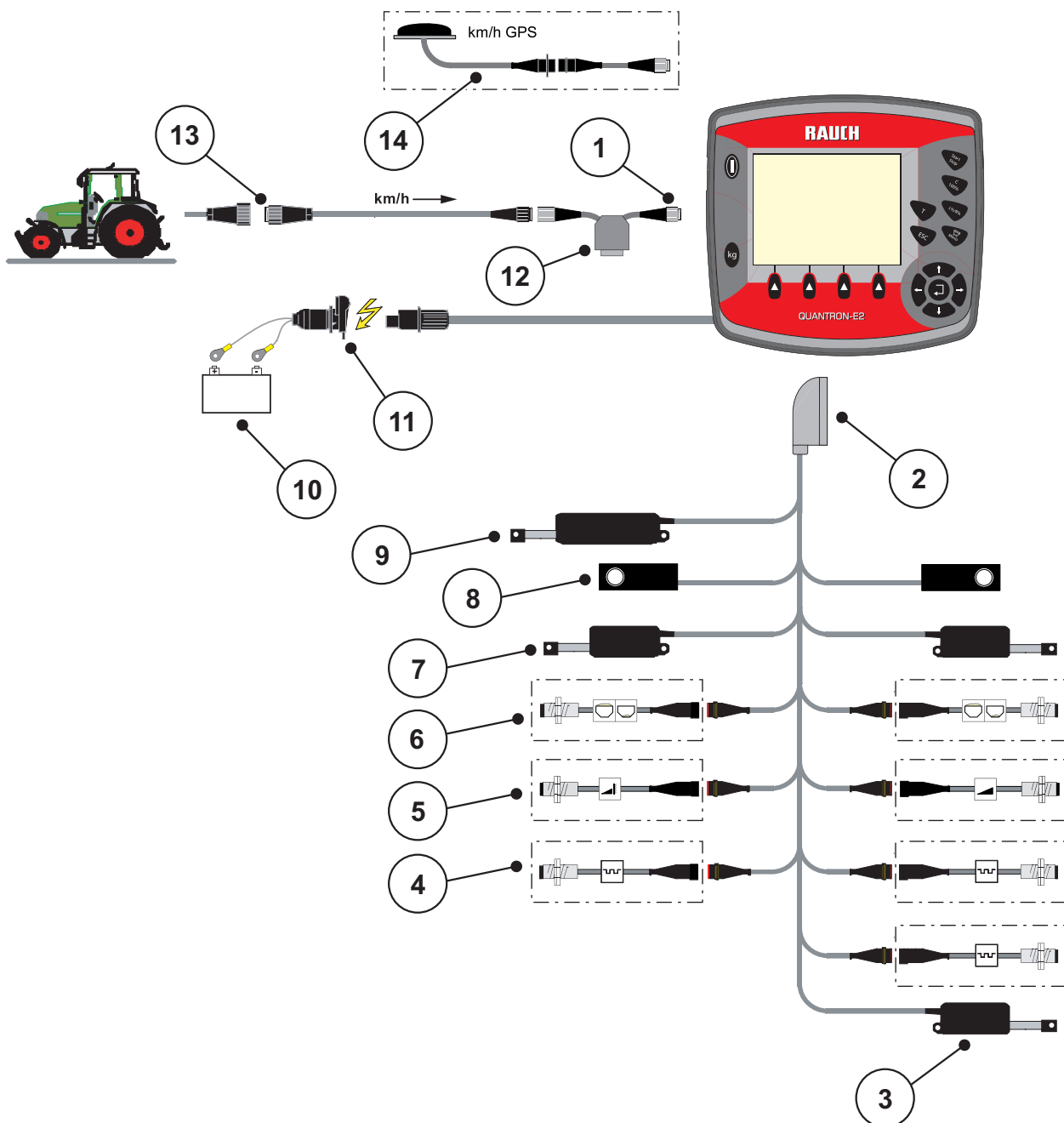
Фиг. 3.3: Схематичен изглед на свързването QUANTRON-E2
