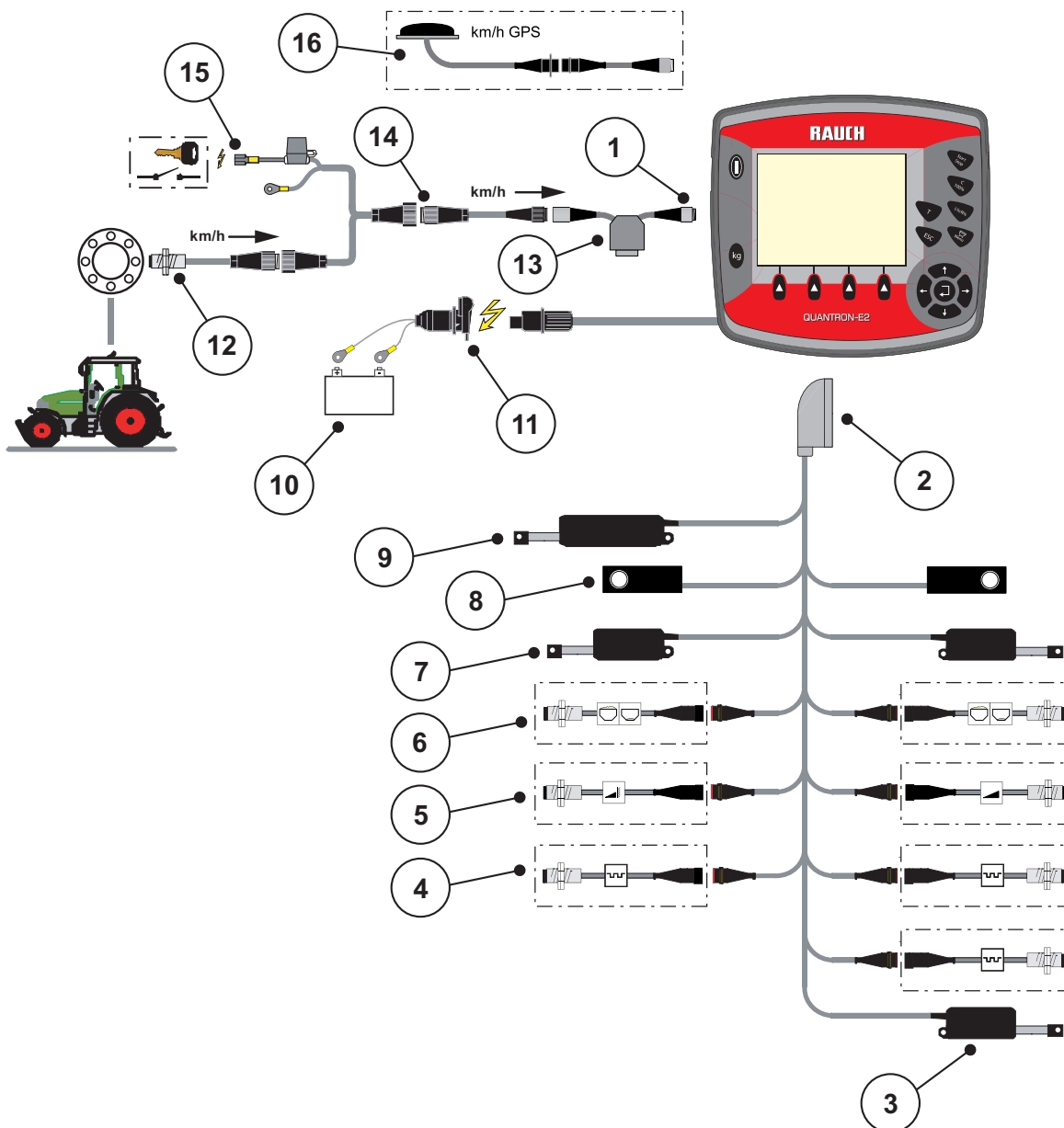
Фиг. 3.5: Схематичен изглед на свързването QUANTRON-E2
