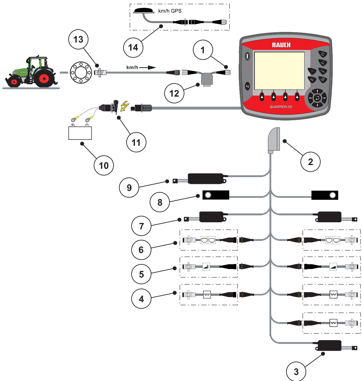
Фиг. 3.4: Схематичен изглед на свързването QUANTRON-E2
