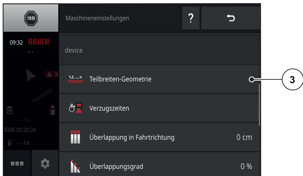
Bild 4.11: Menü Maschineneinstellungen
