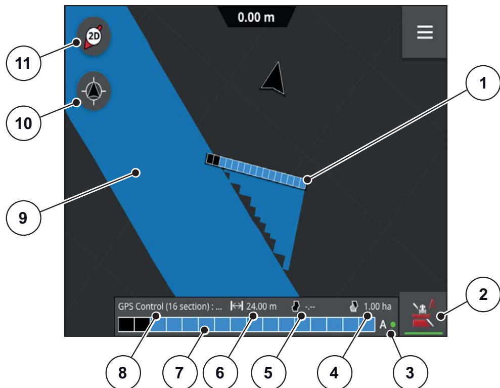
Bild 4.13: Betriebsbild Streufahrt
