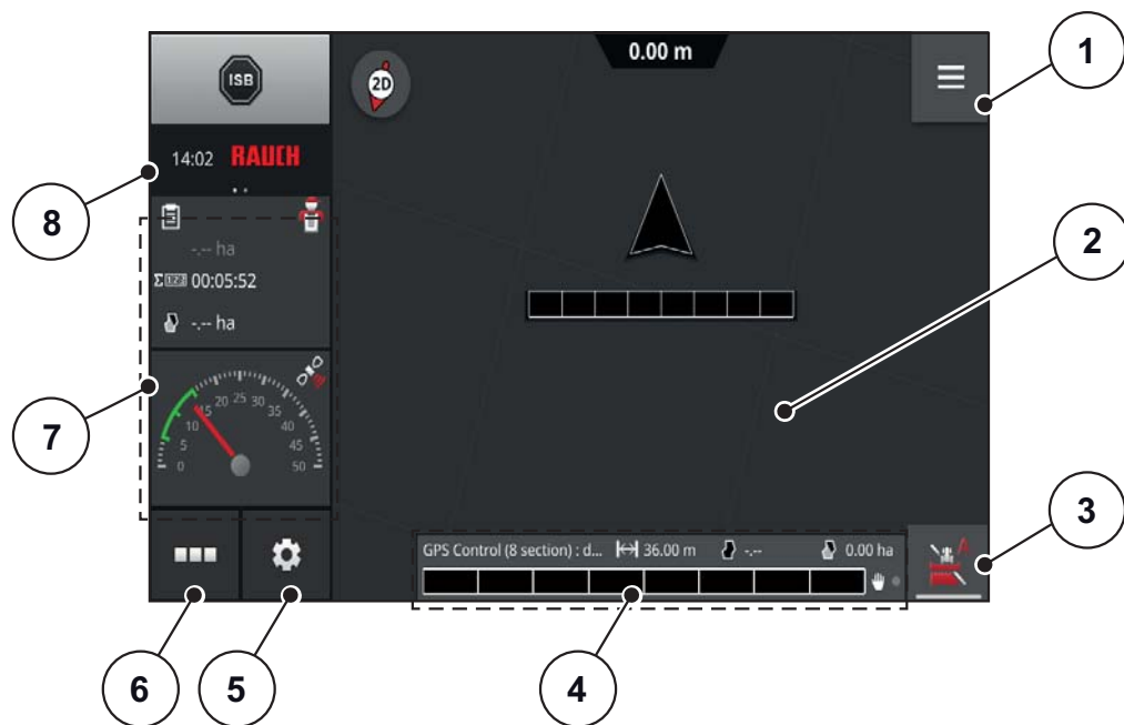
Bild 2.2: CCI 800 Bereiche im Betriebsbild (Beispiel)
