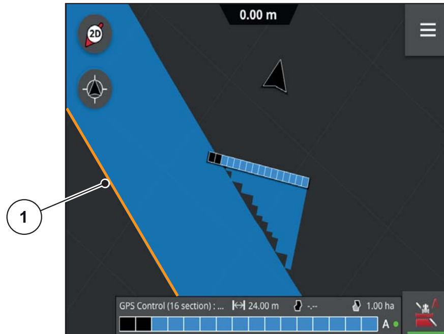
Bild 4.14: Streuen mit Feldgrenze
