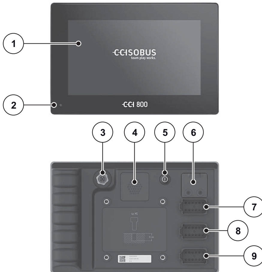
Bild 2.1: CCI 800, Übersicht
