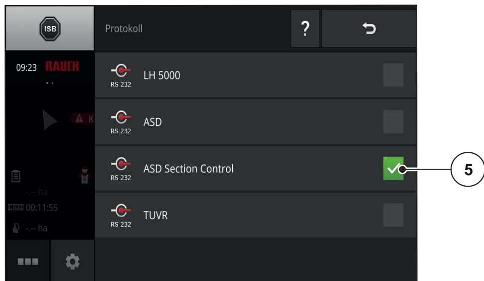
Bild 4.5: Menü Protokoll
