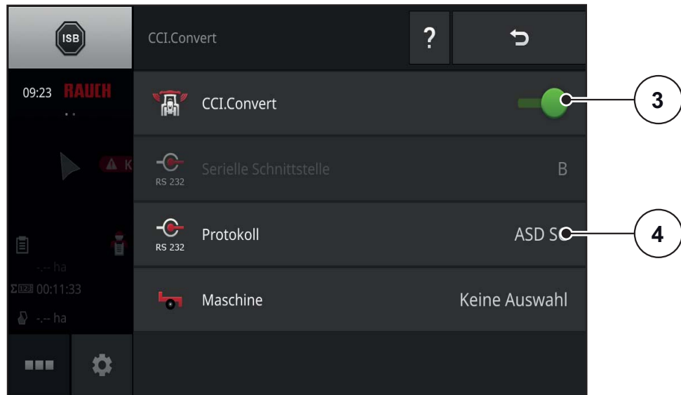
Bild 4.4: Menü CCI.Convert
