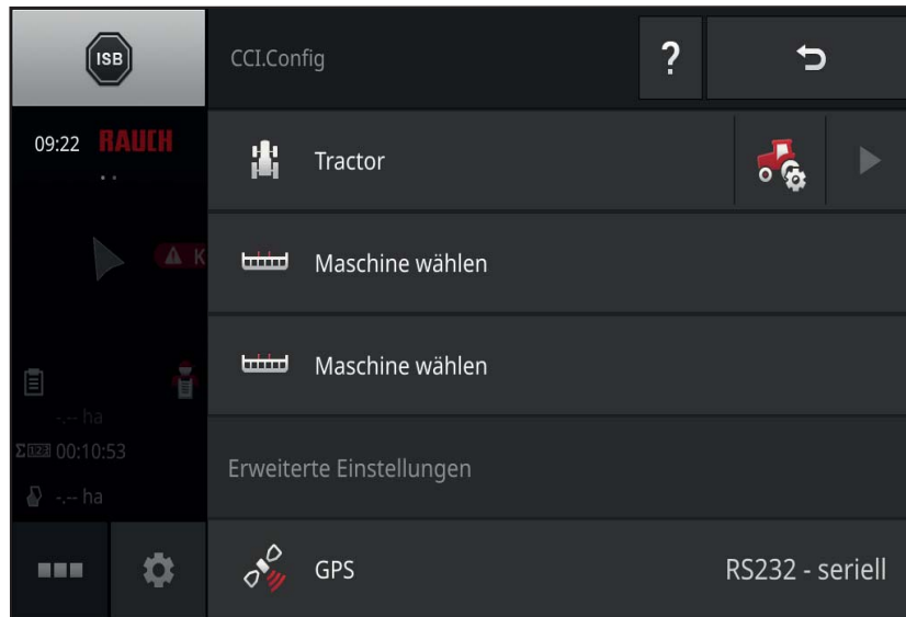
Bild 4.2: Menü CCI.Config
