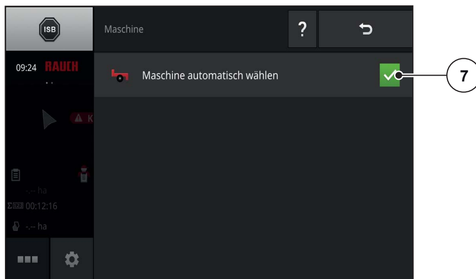
Bild 4.7: Menü Maschine
