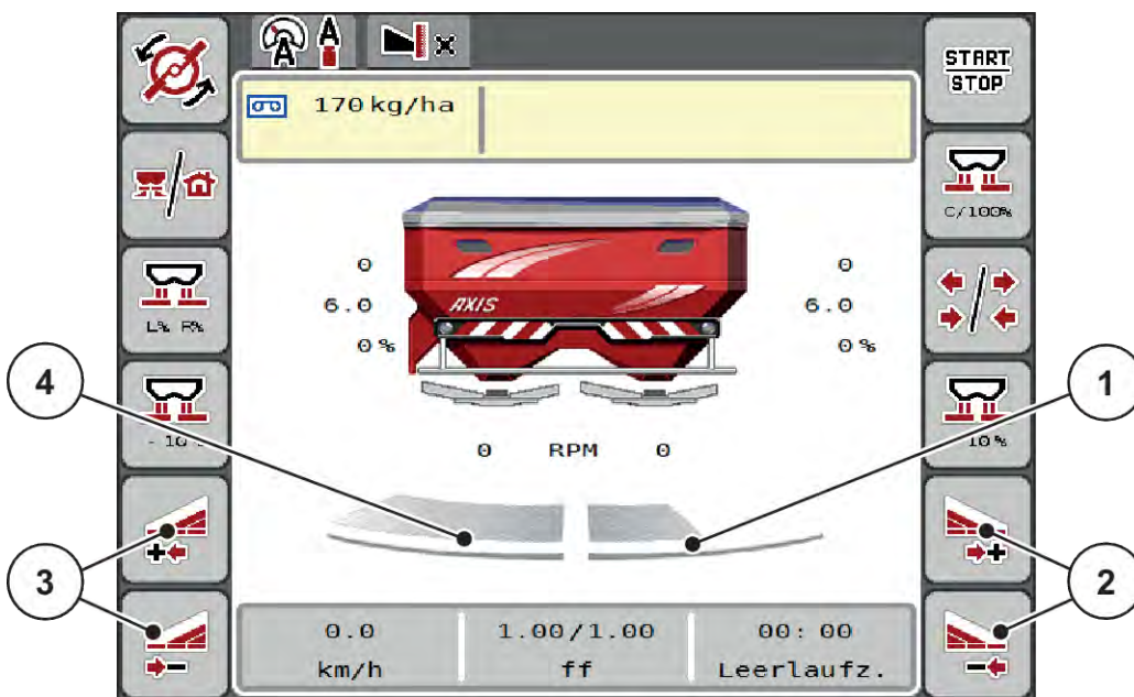
Рис. 38: Робочий екран: Секції штанги з 4 кроками
