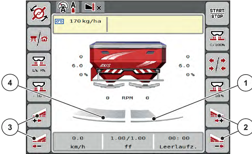
Şek. 38: Çalışma ekranı: 4 kademeli kısmi genişlikler
