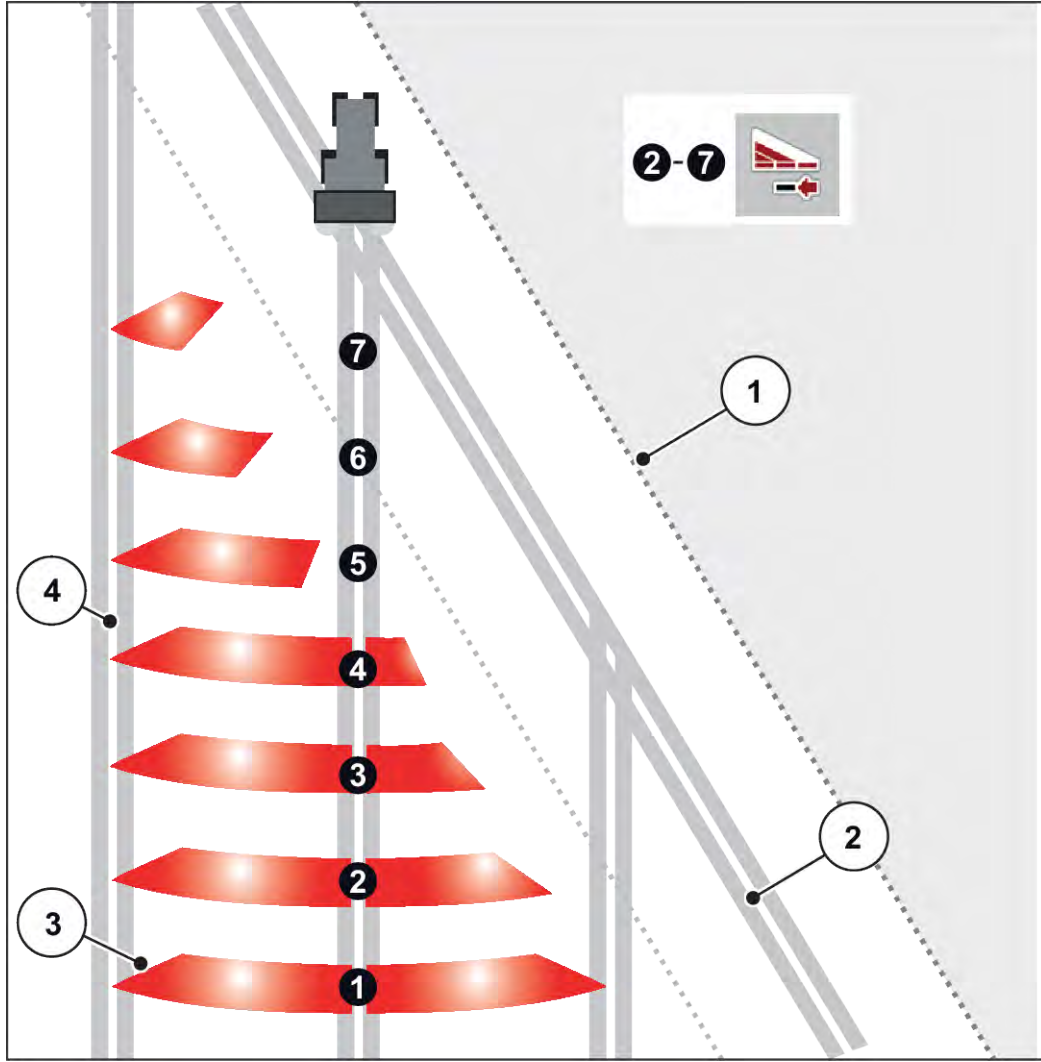
Şek. 41: Otomatik kısmi genişlik anahtarlama
