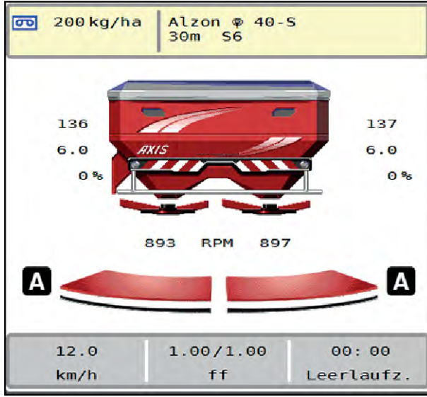
Şek. 46: GPS Control ile çalışma ekranında serpme göstergesi
