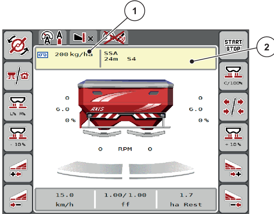
Şek. 17: Serpme tablosunun dokunmatik ekran üzerinden yönetilmesi
