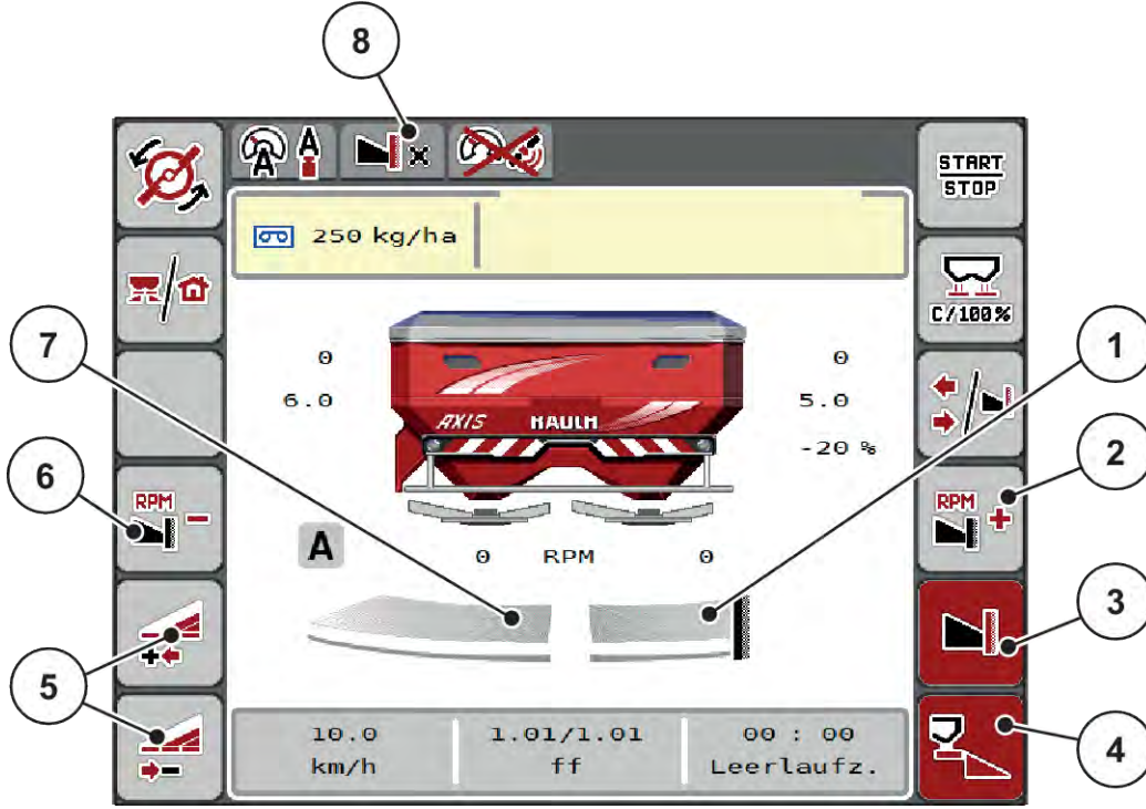
Şek. 42: Çalışma ekranı: Sol kısmi genişlik, sağ sınır serpme tarafı
