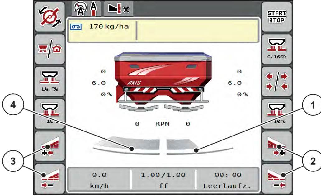
Şek. 40: Çalışma ekranı: Kademesiz kısmi genişlik anahtarlama
