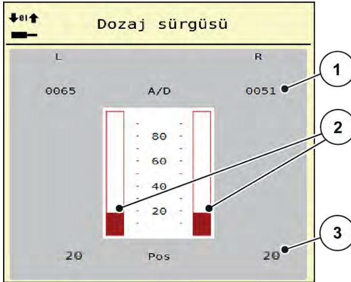
Şek. 23: Test/Teşhis; Örnek: Dozaj sürgüsü
