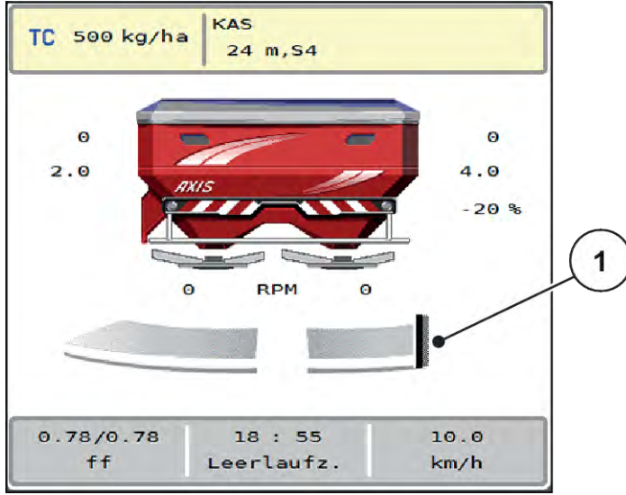
Şek. 37: TELIMAT göstergesi
