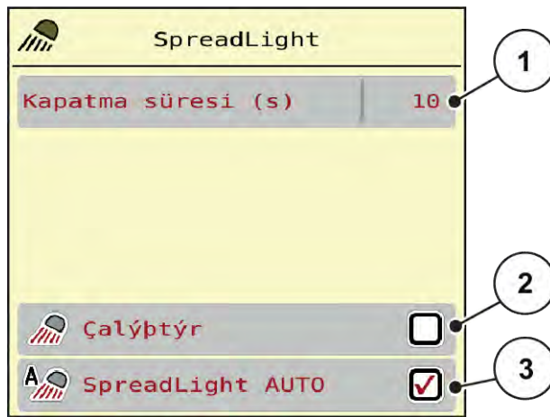
Şek. 28: SpreadLight menüsü
