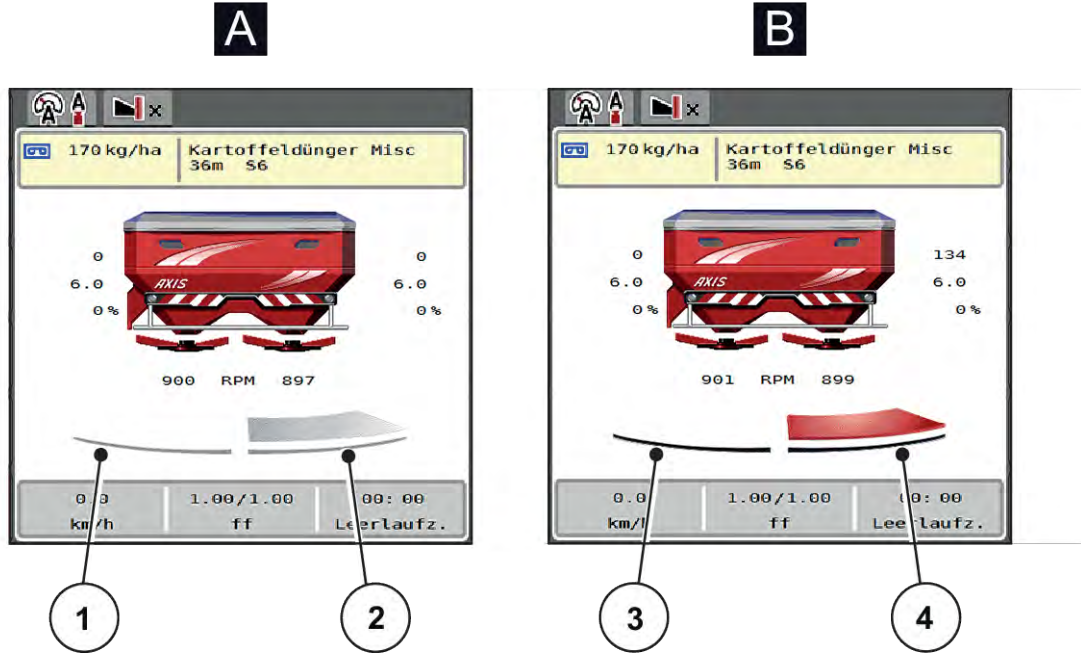
Şek. 4: Dozaj sürgü durumunun göstergesi
