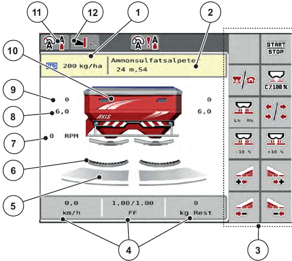
Şek. 2: Makine kumanda sisteminin ekranı
