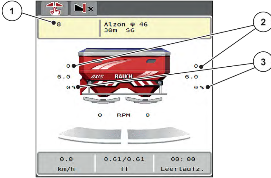
Şek. 45: MAN Skala çalışma ekranı
