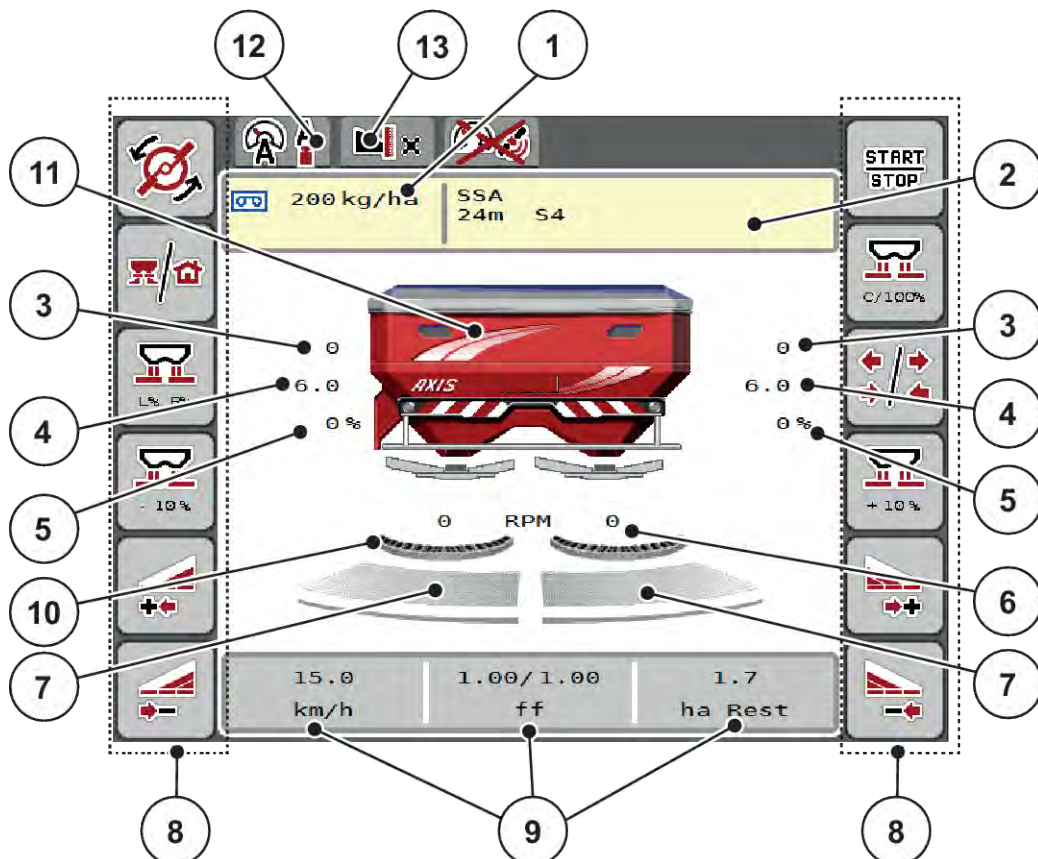
III. 1: Display del comando della macchina
